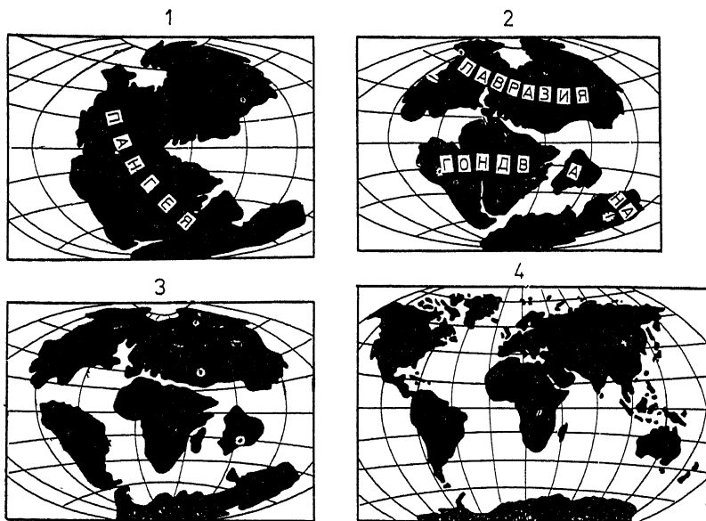
Рис. 20. Распад Пангеи и формирование современных материков (по Р. Диц и Дж. Холден, 1974):
