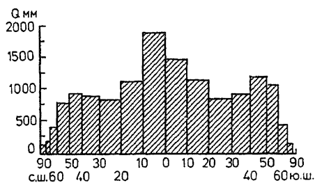
Рис. 24. Распределение средних зональных годовых сумм осадков (С. П. Хромов, 1983)
