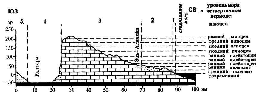
Рис. 36. Геоморфологический профиль через северную часть известнякового Миоценового плато Египта в районе Эль-Аламейна и депрессии Каттара, показывающий связь между современными ландшафтами и геологической историей северного побережья Африки:
