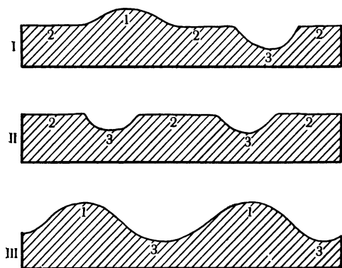
Рис 46 Три типа микрорельефа гильган (по Howard, 1932). I — crabhole, II — melonhole, III — gylgai; 1 — бугорок, 2 — шельф, 3 — депрессия
