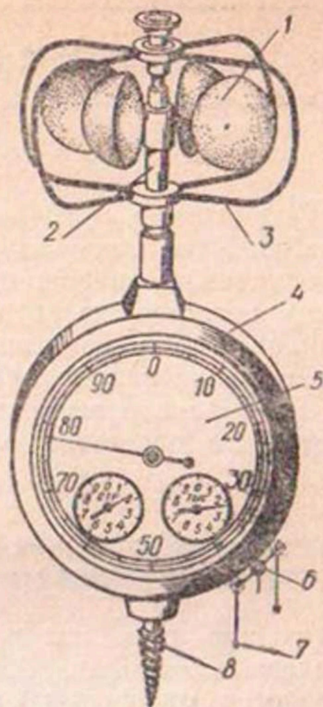
Рис. 3. Ручной анемометр:
