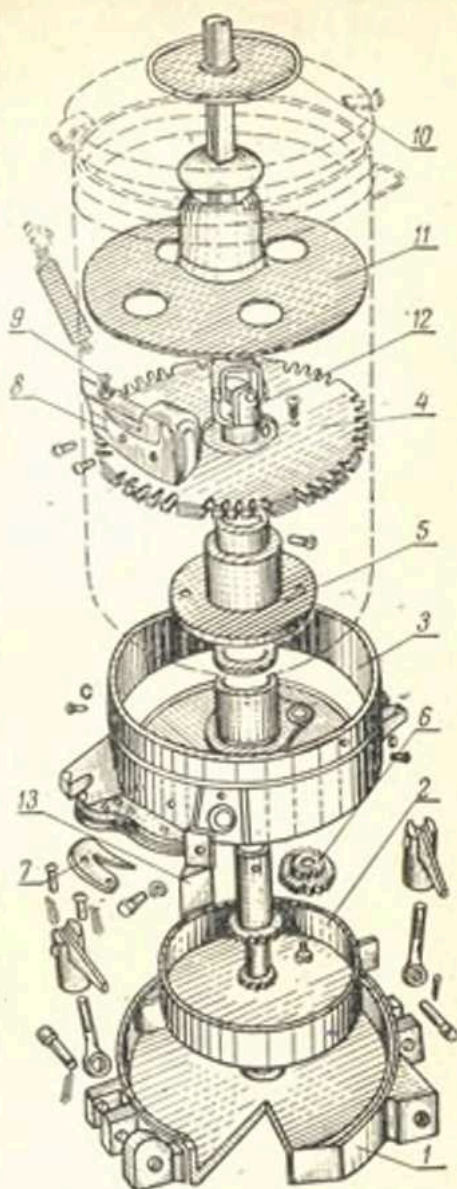
Рис. 10. Высевающий аппарат сеялки СТБХ-4:
