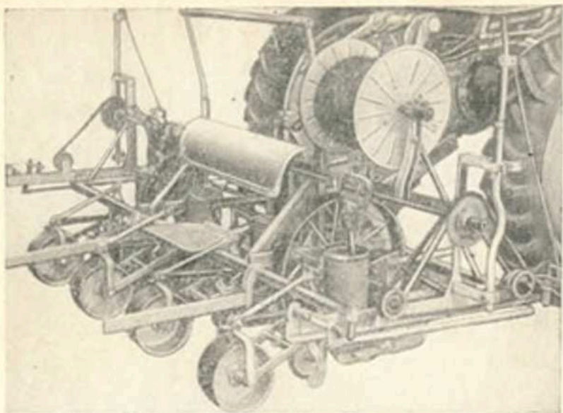
Рис. 8. Сеялка СТВХ-4 (общий вид).
