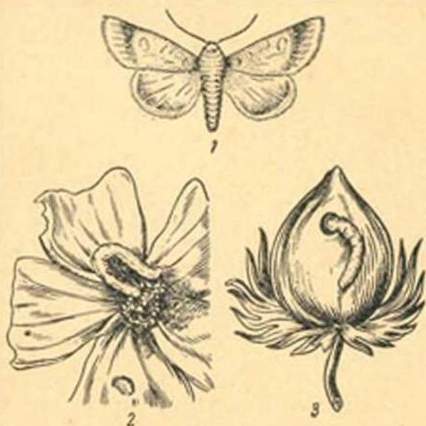
Рис. 37. Хлопковая совка:
