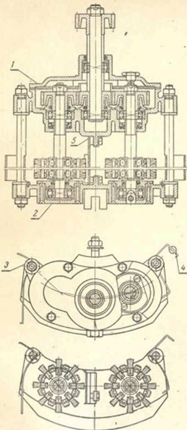
Рис. 24. Щеточный съемник:
