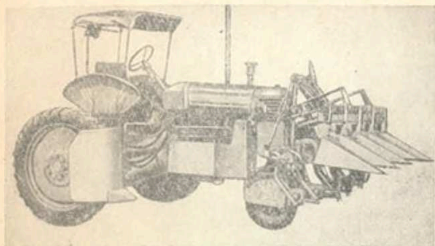
Рис. 17. Приспособление для чекилки хлопчатника ЧВХ-4 к культиватору-удобрителю НКУ-4-6А.
