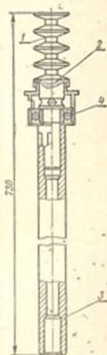
Рис. 23. Шпиндель хлопкоуборочной машины ХВС-1,2:
