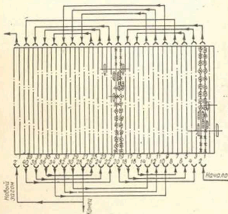
Рис. 28. Схема заездов в рядки машины ХВС-1,2.
