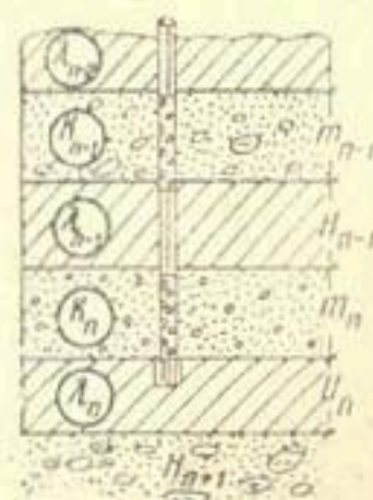
Рис. 1. Схема заложения скважины в n пластах.
