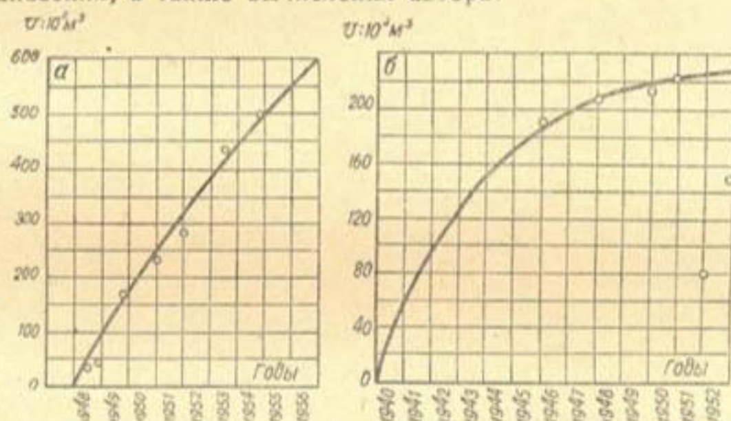
Рис. 2. Изменение объема занесения и подпертом бьефе: а — Сары-Курганского; б — Кампыр-Раватского. 1 — расчетная кривая; 2 — данные полевых исследований.
