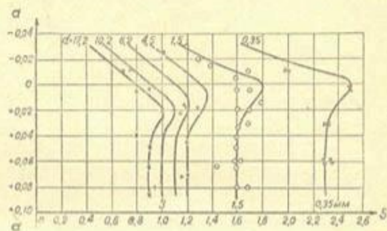
Рис. 6. Длина вымояны S при расходе q = 0,056 м 3 /сек. L = 1,5H ; H = 0,28 м; d от 0,35 до 17,2 мм.
