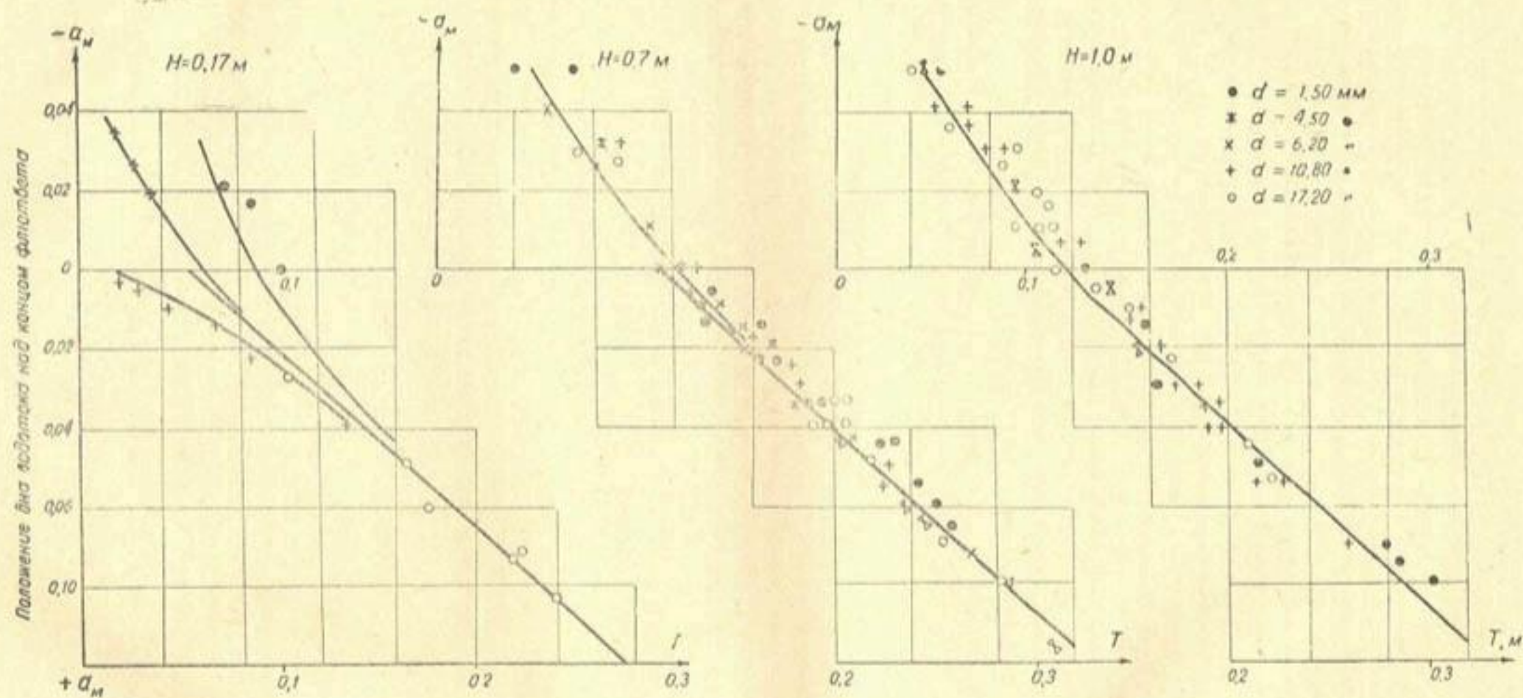
Рис. 5. Наибольшая глубина размыва при q = 0.056 \text{ м}^3/\text{сек} . Линия 0—0 на отметке dna крепления. Длительность пропуска воды в опыте равна 1 часу:
