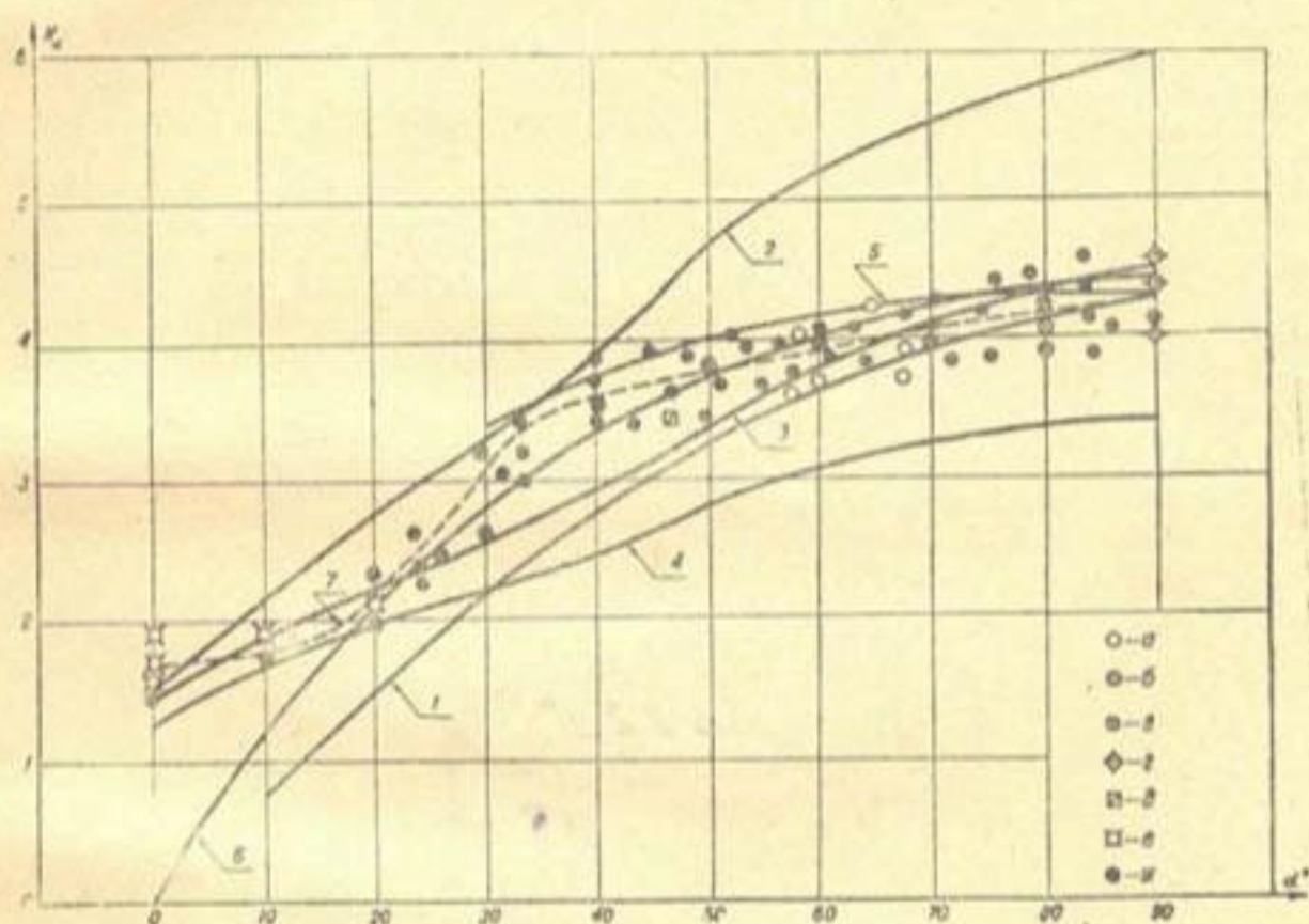
Рис. 2. Зависимость k_a = f(\alpha) по формулам: Замарина (1), Вызго — для легко размываемых, слабых и прочных грунтов (2, 3, 4), Михалева (5), Рэлей (6), автора (7).
