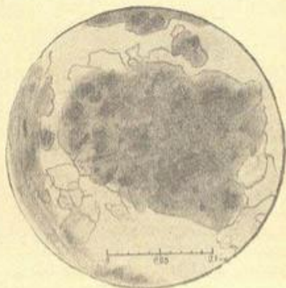
Рис. 2. Микроагрегат диаметром 0,25–0,1 мм типичного серозема. Гориз. 0–5 см. Увеличение 550, препарат № 50 (микрозарисовка автора).
