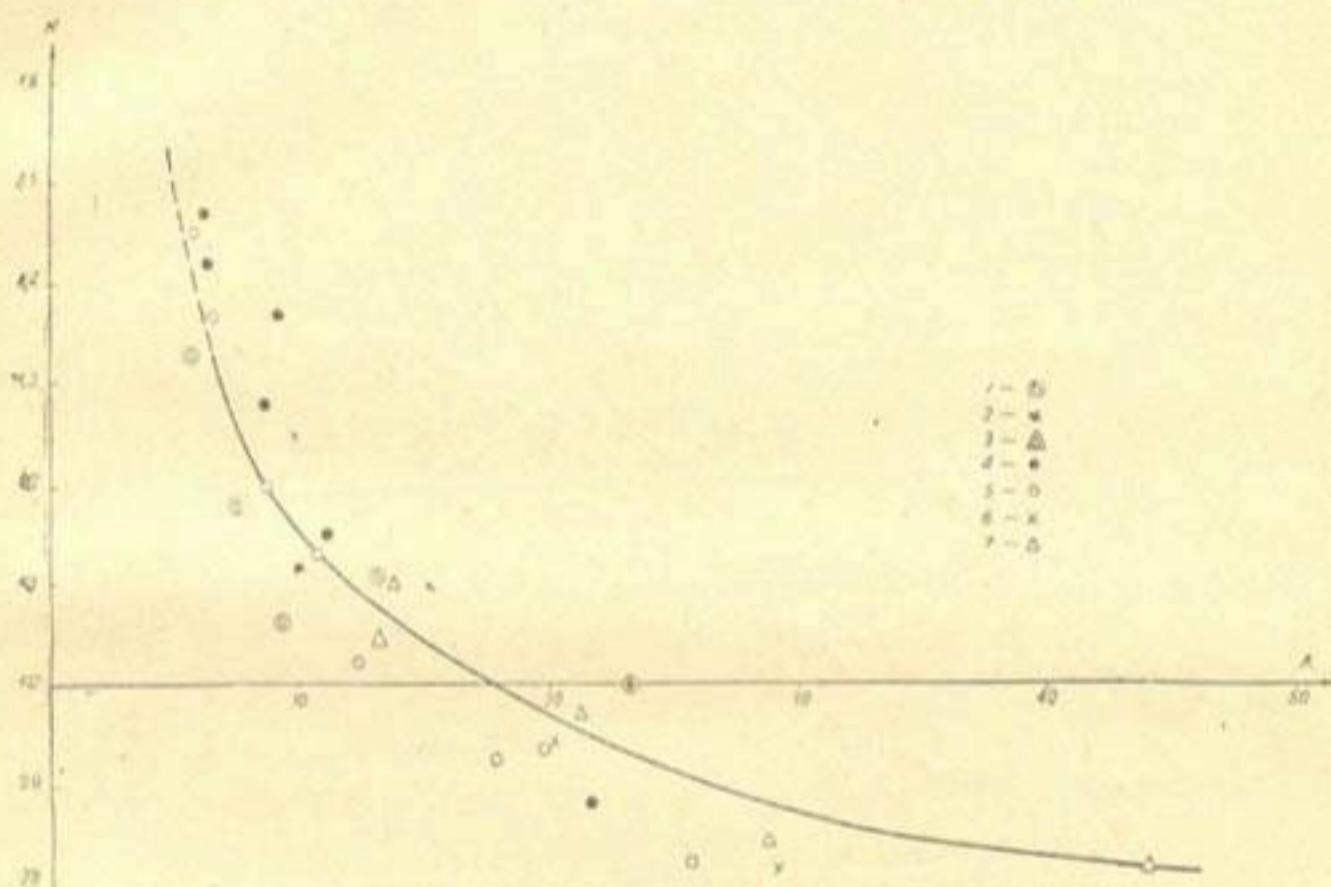
Рис. 7. Опыты по местному размыву за горизонтальным креплением при \eta_{ср} = 4,3 . Значения K приведены к условиям мелкого песка и шероховатости стального дна. Условные обозначения:
