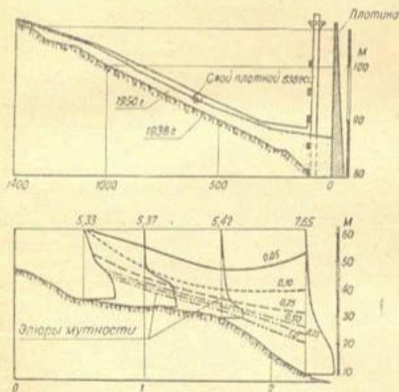
Рис. 3. Протекание потока, насыщенного взвешенными наносами.
