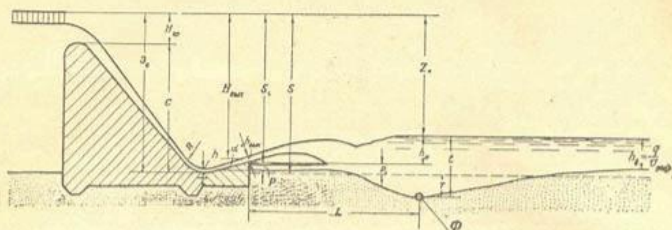
Рис. 1. Общая схема. Обозначения: \Phi — фокус размыва; пунктир — дно русла до размыва.
