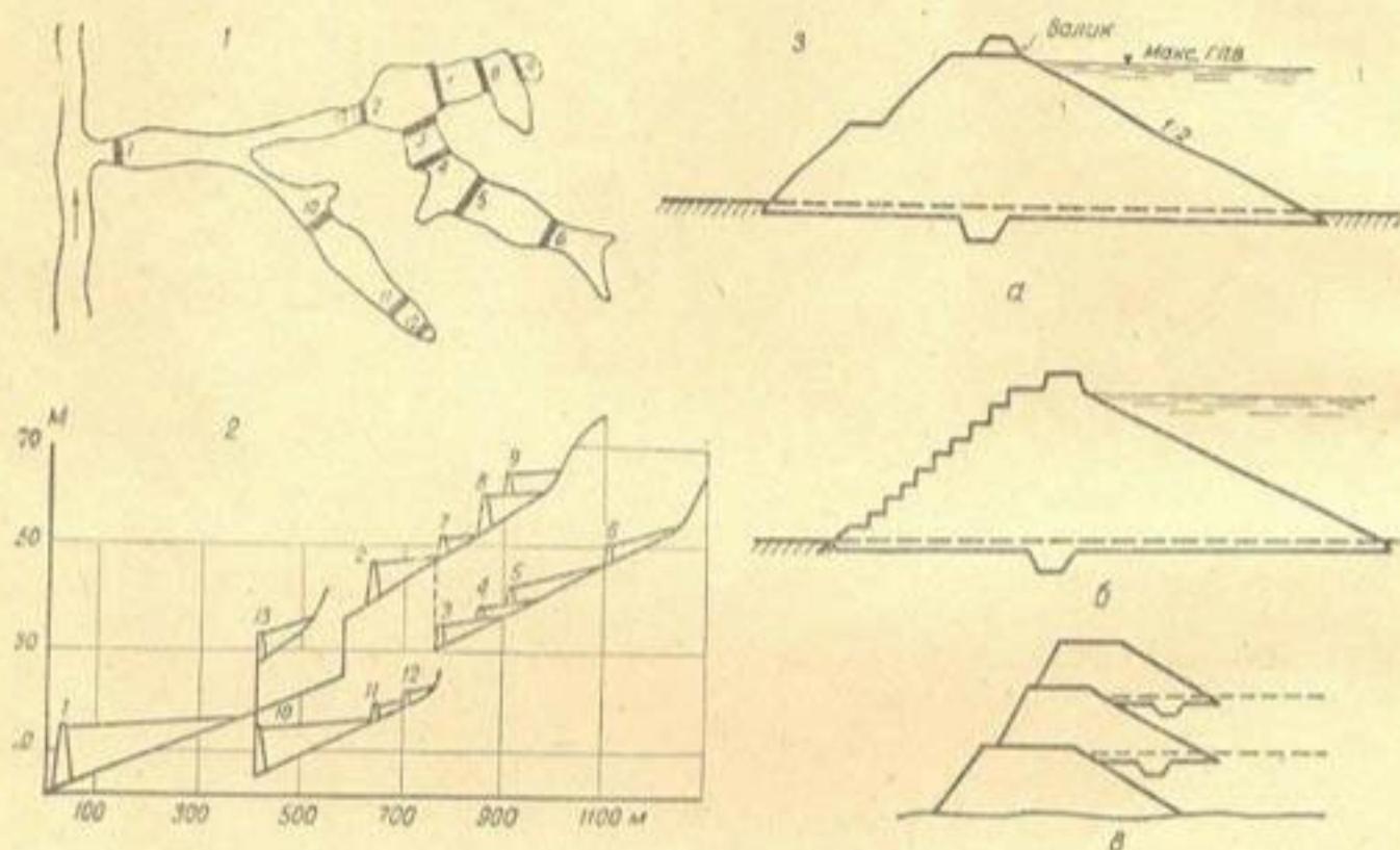
Рис. 7. Размещение и профили земляных плотин по удержанию почвы от смыва (уезд Митань, овраг Нянь-Пянь Мах):
