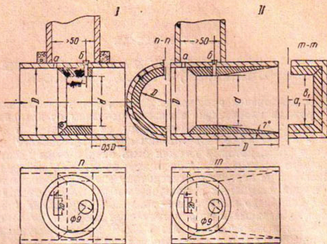
Рис. 1. Водомерное устройство на выходе трубчатого регулятора: I — цилиндрическое кольцо; II — тип Вентури.
