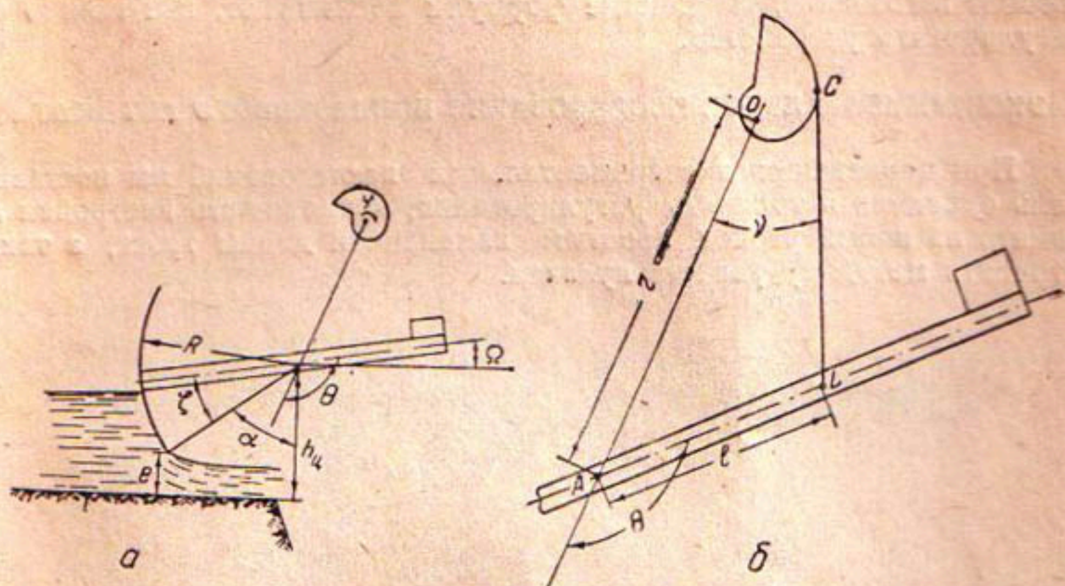
Рис. 2. Положение основных элементов автомата.
