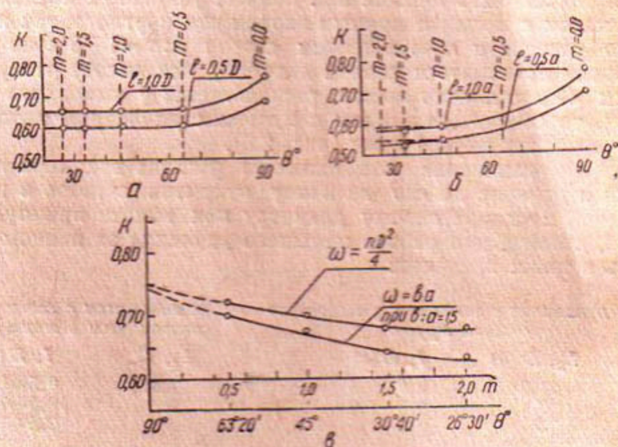
Рис. 4. Графики K = f(\theta) для приставок круглого и прямоугольного сечения.
