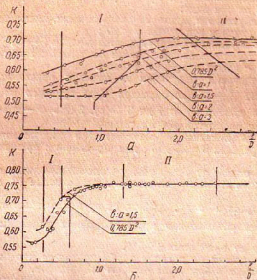
Рис. 2. Графики K = f_1 \left( \frac{l}{D} \right) или K = f_2 \left( \frac{l}{a} \right) для приставок круглого (прямая линия) и прямоугольного (пунктирная линия) сечения: a - \theta = 45^\circ , b - \theta = 90^\circ ; I — зона с K = f_1 \left( \frac{l}{D} \right) или K = f_2 \left( \frac{l}{a} \right) ; II — зона с K = \text{const}
