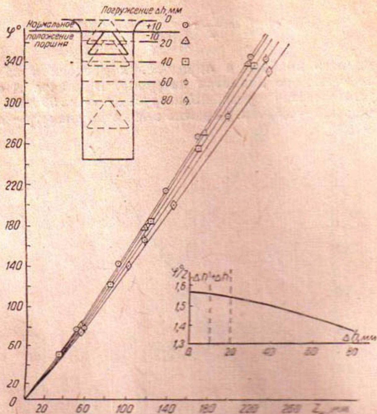
Рис. 6. График \varphi = f(z_h) при различных погружениях поршня в патрубок прибора.
