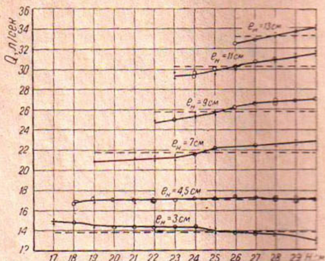
Рис. 6. Работа автомата при различных открытиях затвора.
