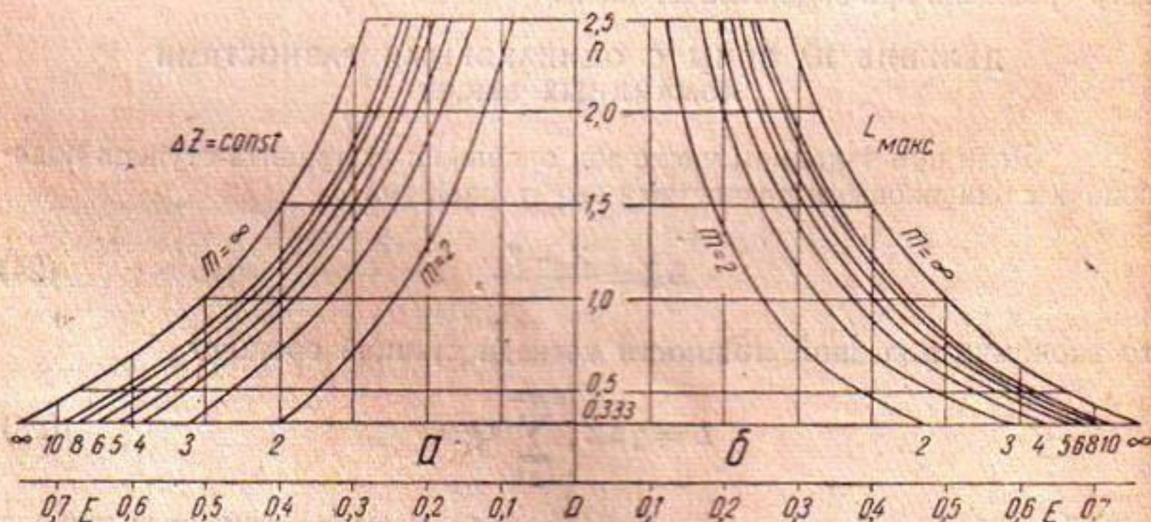
рис. 6. Сравнительный график энергетической экономичности зональных систем: а—равномерное по высоте размещение ступеней володачи; б—энергетически выгодное распределение ступеней.
