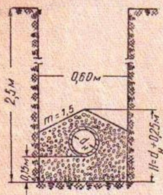
Рис. 4. Конструкция закрытой дрены.
