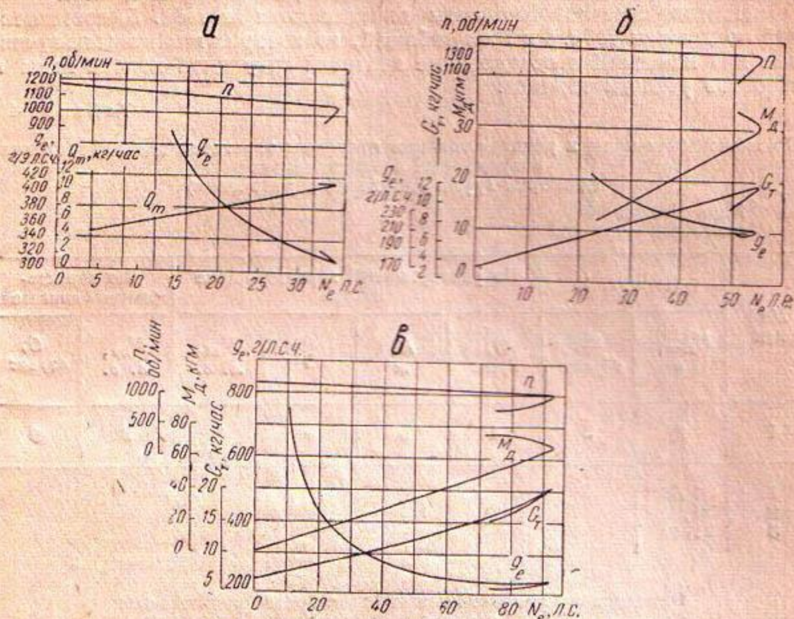
Рис. 5. Регуляторная характеристика двигателя: а—СТЗ-ХТЗ (топливо керосин); б—трактора ДТ-54; в—трактор С-30.
