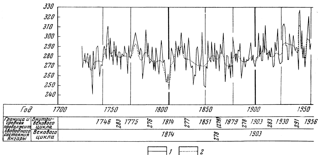
Рис. 24. Многолетние колебания продолжительности свободного состояния р. Ангары у г. Иркутска 1 — годовые значения; 2 — индекс \Sigma a_m/n
