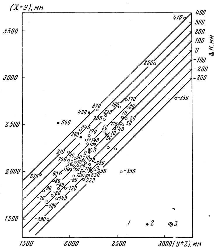
Рис. 16. Графики связи между годовыми значениями прихода, расхода и приращения уровня воды оз. Байкал 1 — годовые значения естественного режима; 2 — то же, зарегулированного; 3 — среднееголетнее значение за 1901—1953 гг.
