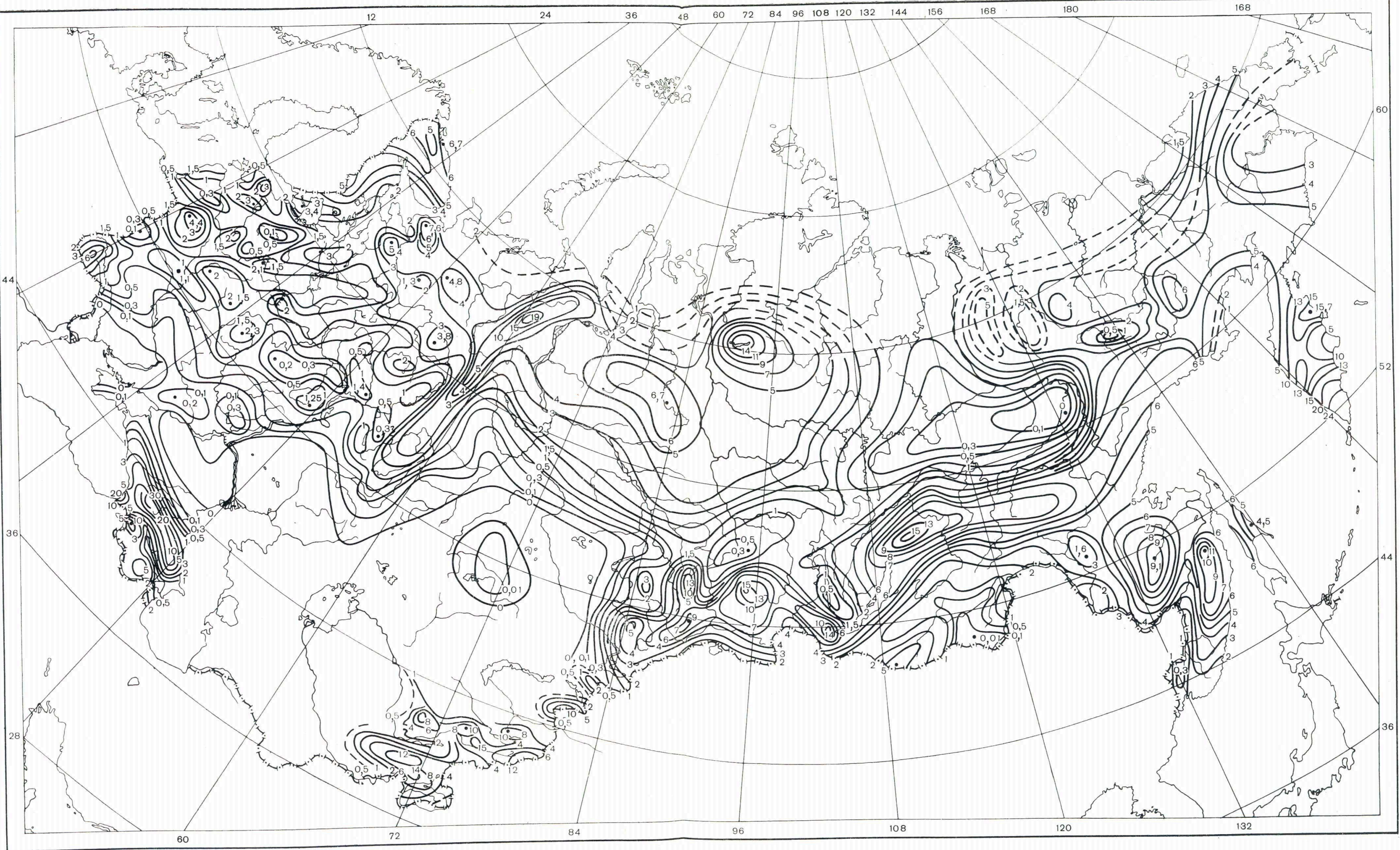
Рис. 39. Карта минимального 30-дневного летне-осеннего стока 80%-ной обеспеченности (л/с·км²).
