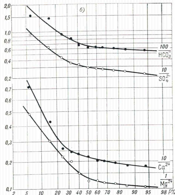
ции (а) и содержания анионов и катионов (б) в реке (мг/л).
