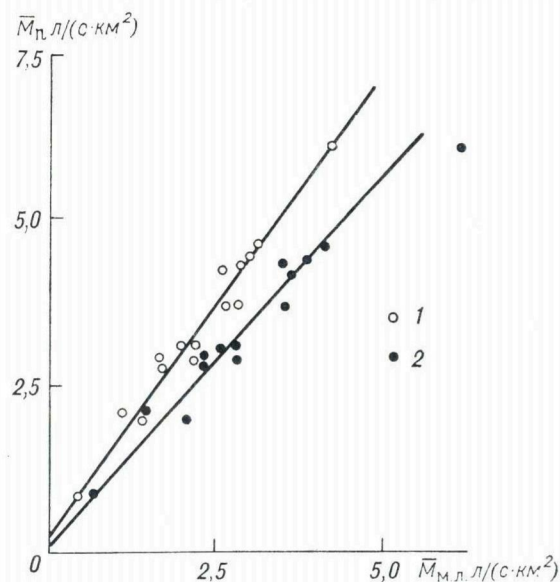
Рис. 4. Связь нормы подземного стока M_p с нормой минимального летне-осеннего стока M_{м.л.} (бассейн р. Немана).
