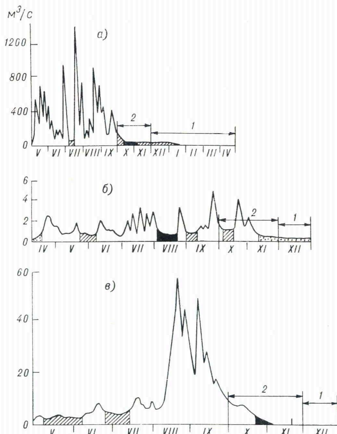
Рис. 21. Гидрографы рек Калакан у с. Калакан (а), Кичмари у ст. Малмыж (б) и Заы у с. Усть-Заза (в).
