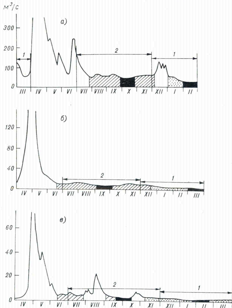
Рис. 14. Гидрографы рек Великой у д. Пятаново (а), Баксы у д. Пиховки (в) в средние по водности годы, р. Колпи у д. Верхний Двор (б) в маловодный год.
