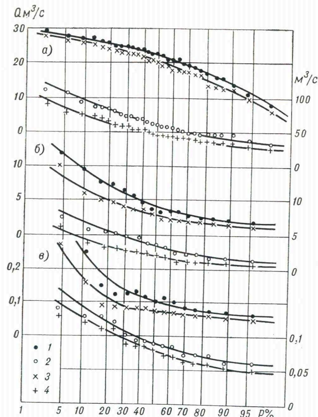
Рис. 46. Эмпирические кривые обеспеченности минимальных 30-дневных и среднесуточных расходов воды.
