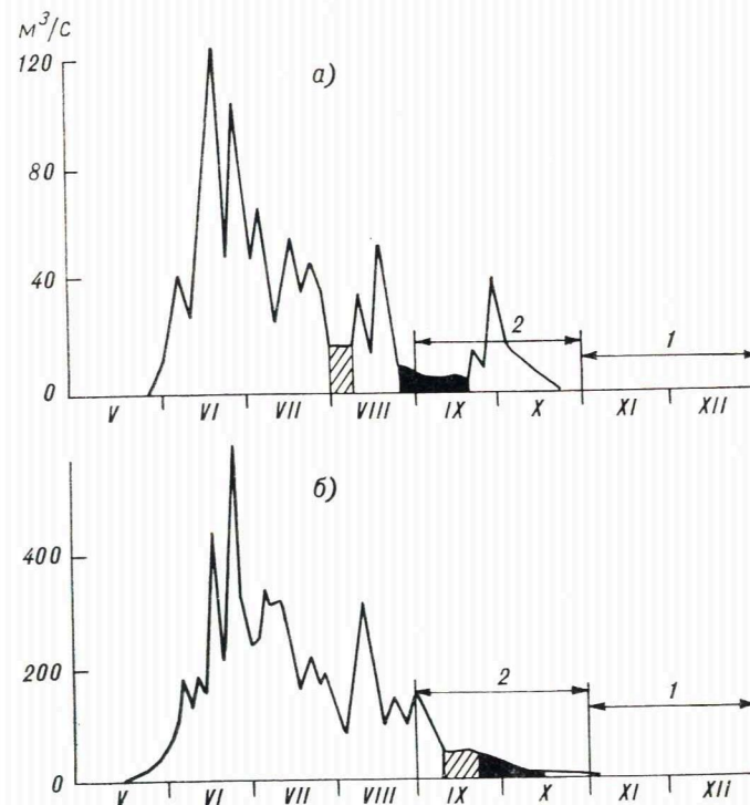
Рис. 19. Гидрографы рек Эбитиэм у м. Эбитем (а) и Чаркы в 3,5 км от устья (б).
