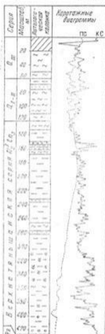
Рис. 11. Характер строения верхне-тиеншаньской серии на окраине пред-нуратинской пролювиальной равнины, разрез скв. 4.
