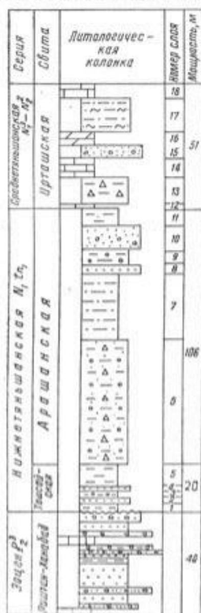
Рис. 4. Строение ташкентской, арашанской и иртышской свит в разрезе Ташкент (Ангренское плато).
