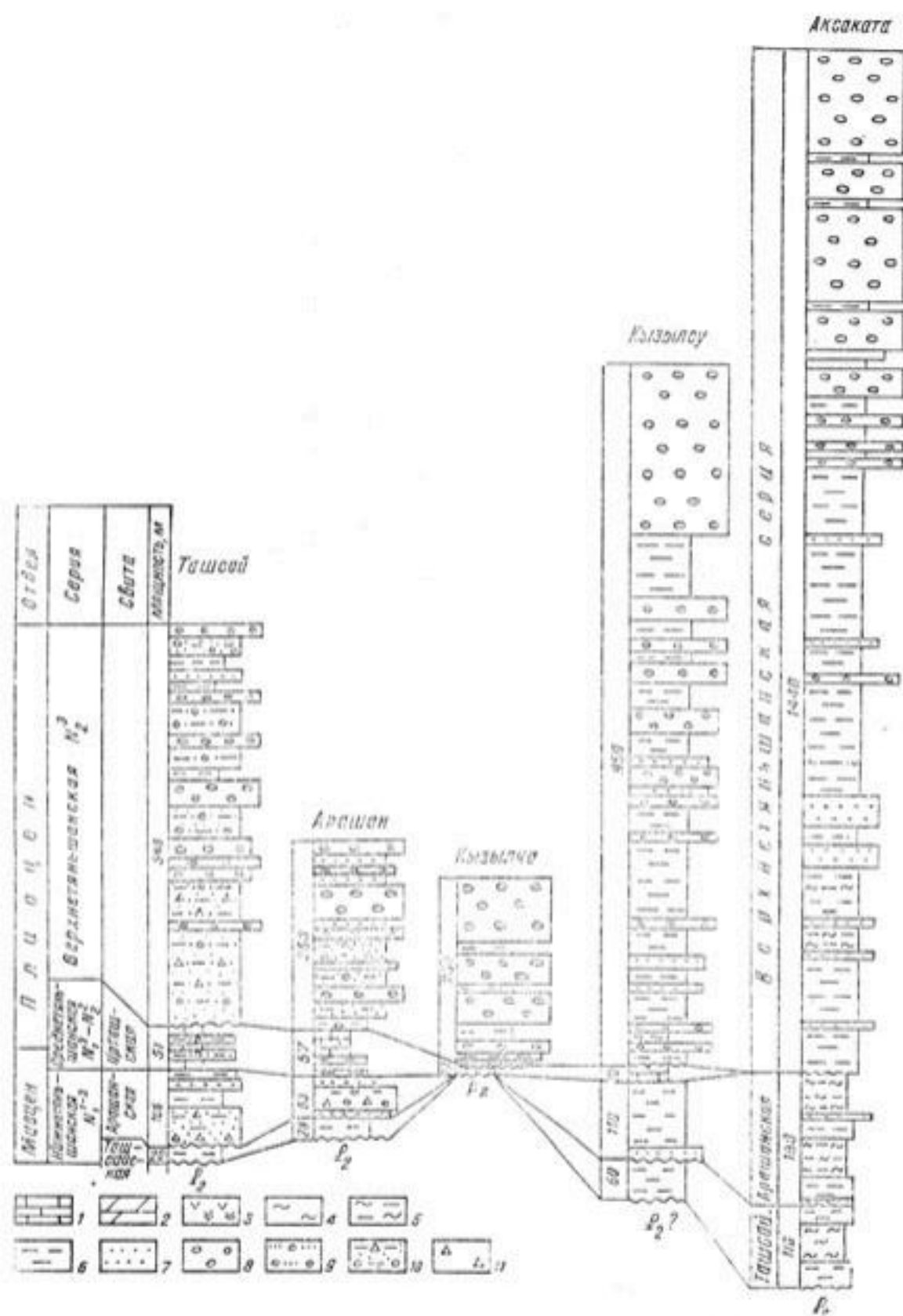
Рис. 3. Схема сопоставления опорных разрезов неогена долины Чирчика (Аксаката, Кызыласу) и Анграна (Ташсай, Арашан, Кызылча). Литологические типы пород:
