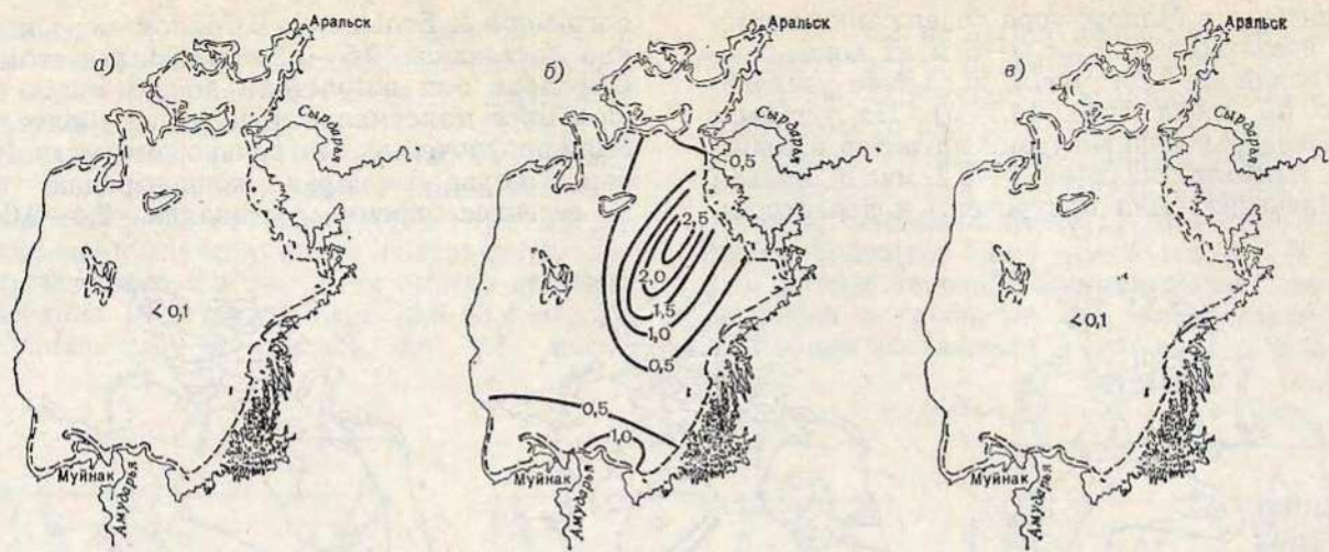
Рис. 14.13. Среднее многолетнее (1971—1975) распределение нитритов на поверхности моря весной (а), летом (б) и осенью (в), мкг/л.
