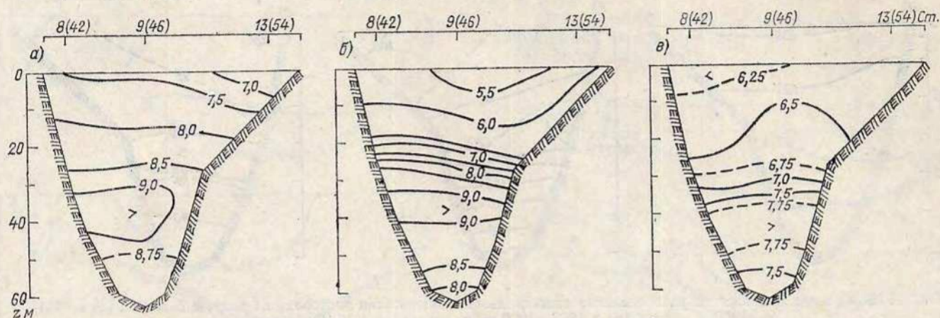
Рис. 16.16. Среднее многолетнее (1961—1965) распределение абсолютного содержания кислорода на разрезе Б весной (а), летом (б) и осенью (в), мл/л.
