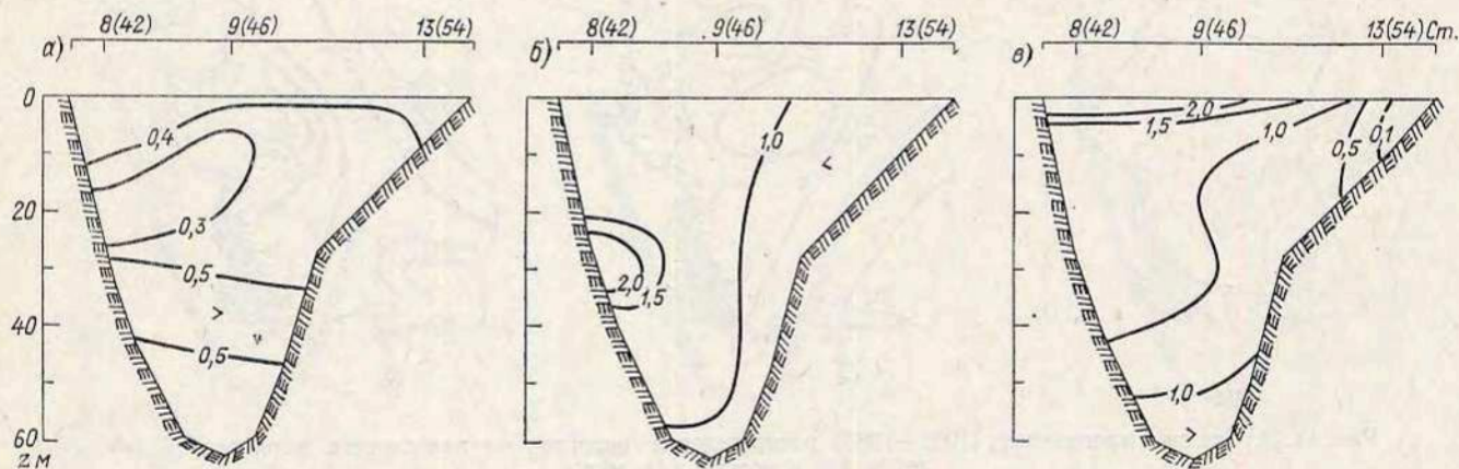
Рис. 14.12. Среднее многолетнее (1961—1965) распределение нитритов на разрезе Б весной (а), летом (б) и осенью (в), мкг/л.
