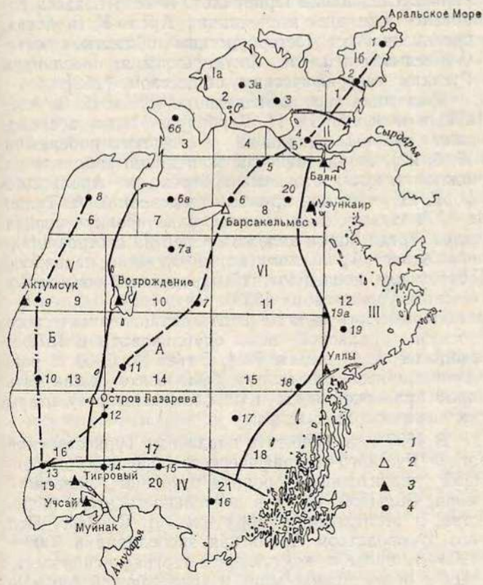
Рис. 1.2. Расположение сети гидрометеорологических станций и постов, вековых океанографических станций и разрезов, гидрологических районов (I—VI) моря. Схема квадратов (1—21), принятых при обработке материалов океанографических наблюдений.
