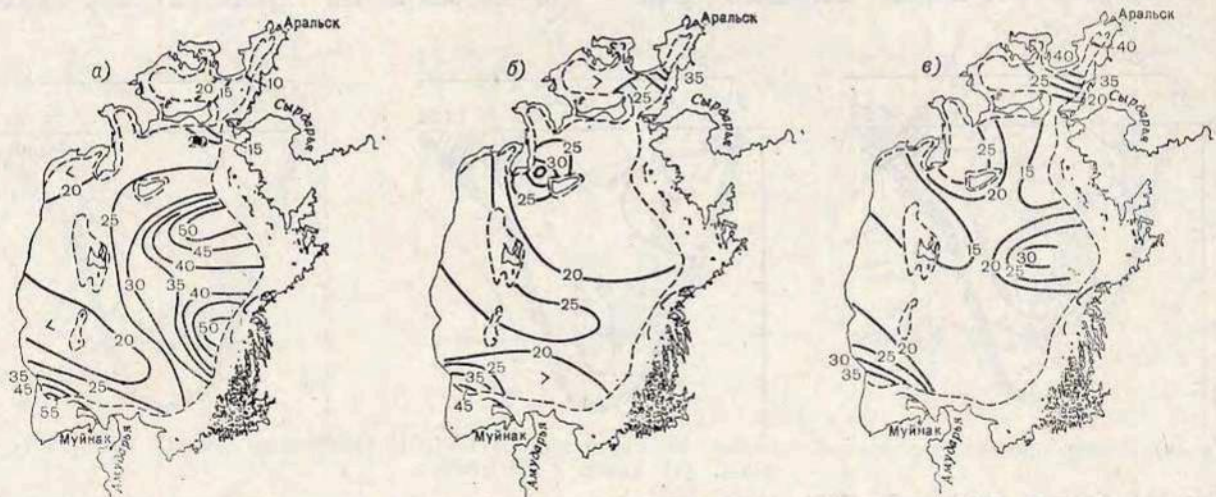
Рис. 14.7. Среднее многолетнее (1981—1985) распределение фосфатов на поверхности моря весной (а), летом (б) и осенью (в), мкг/л.
