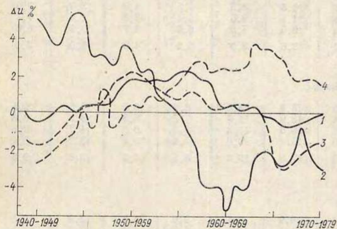
Рис. 2.4. Многолетние изменения 10-летних скользящих средних отклонений от нормы относительной влажности.
