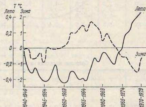
Рис. 2.3. Многолетние изменения 10-летних скользящих средних отклонений от нормы температуры воздуха зимой и летом.
