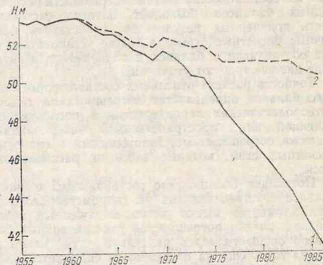
Рис. 4.3. Межгодовая изменчивость фактического (1) и восстановленного (2) уровня Аральского моря.
