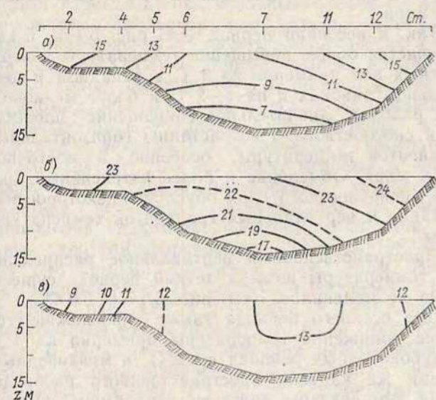
Рис. 5.5. Среднее многолетнее (1976—1985) распределение температуры воды на разрезе А весной (а), летом (б) и осенью (в), °С.
