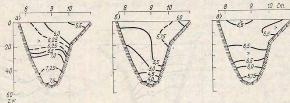
Рис. 16.18. Среднее многолетнее (1981—1985) распределение абсолютного содержания кислорода на разрезе Б весной (а), летом (б) и осенью (в), мл/л.
