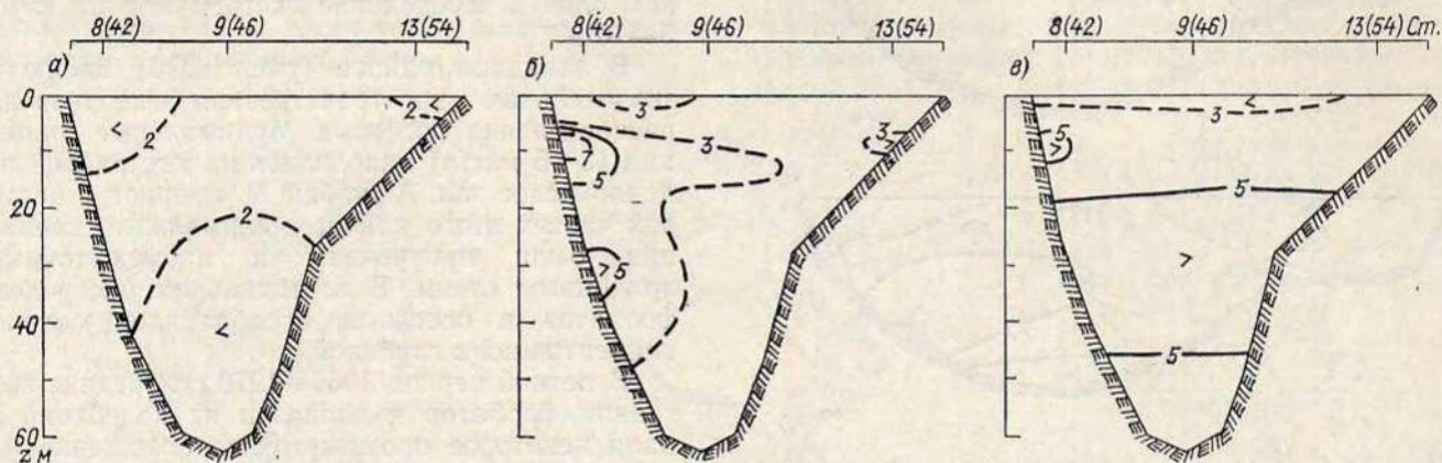
Рис. 14.3. Среднее многолетнее (1961—1965) распределение фосфатов на разрезе Б весной (а), летом (б) и осенью (в), мкг/л.
