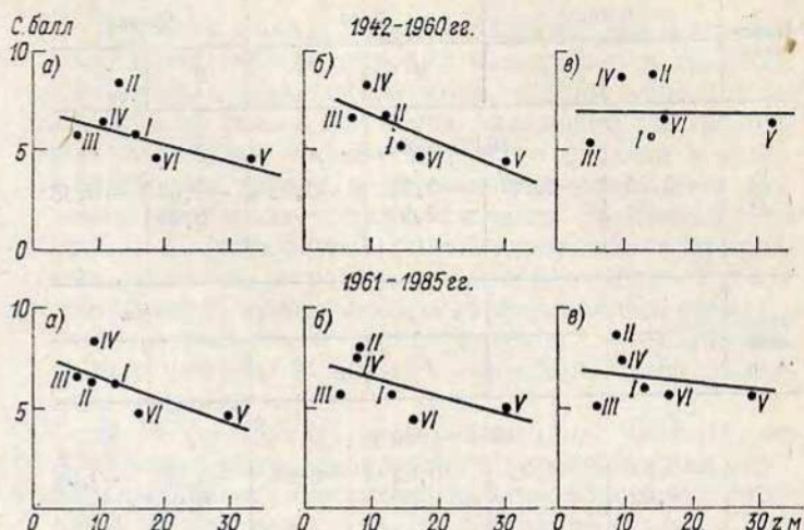
Рис. 11.5. Зависимости средних сезонных значений цвета морской воды от глубины моря для характерных периодов.
