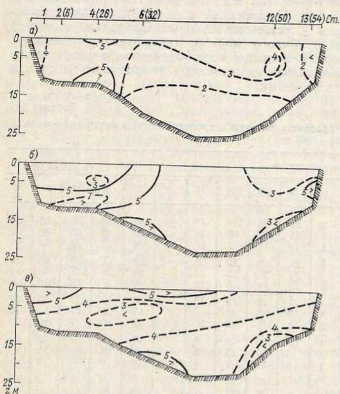
Рис. 14.2. Среднее многолетнее (1961—1965) распределение фосфатов на разрезе А весной (а), летом (б) и осенью (в), мкг/л.
