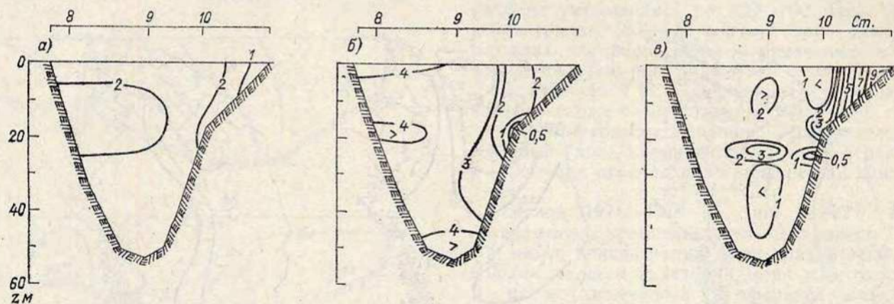
Рис. 14.18. Среднее многолетнее (1981—1985) распределение нитритов на разрезе Б весной (а), летом (б) и осенью (в), мкг/л.
