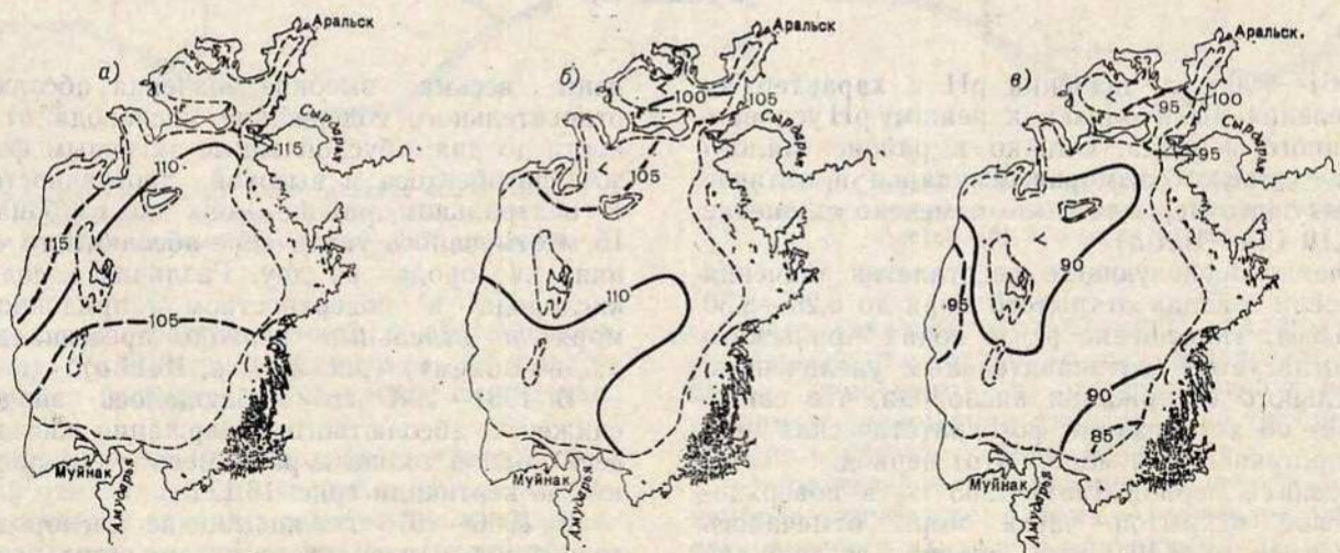
Рис. 16.6. Среднее многолетнее (1981—1985) распределение относительного содержания кислорода на поверхности моря весной (а), летом (б) и осенью (в), %.
