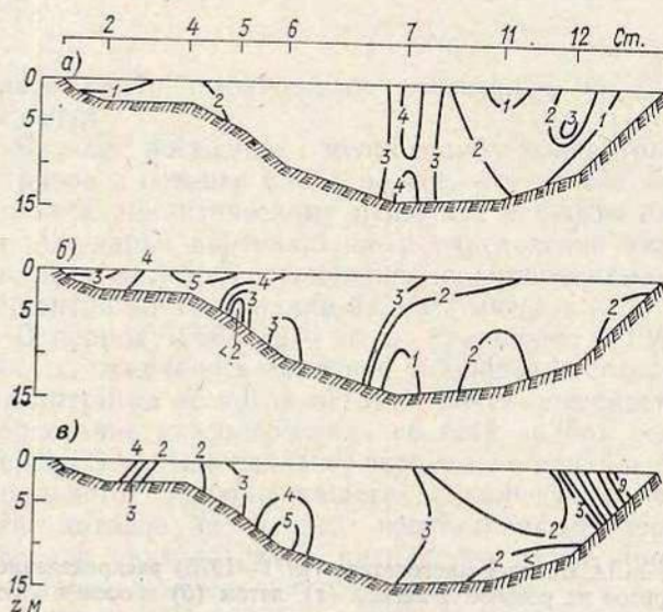
Рис. 14.17. Среднее многолетнее (1981—1985) распределение нитритов на разрезе А весной (а), летом (б) и осенью (в), мкг/л.
