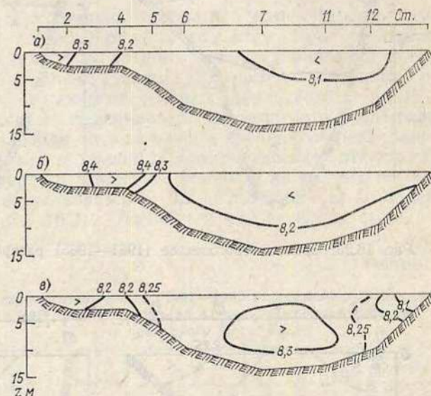
Рис. 16.24. Среднее многолетнее (1981—1985) распределение pH на разрезе А весной (а), летом (б) и осенью (в).
