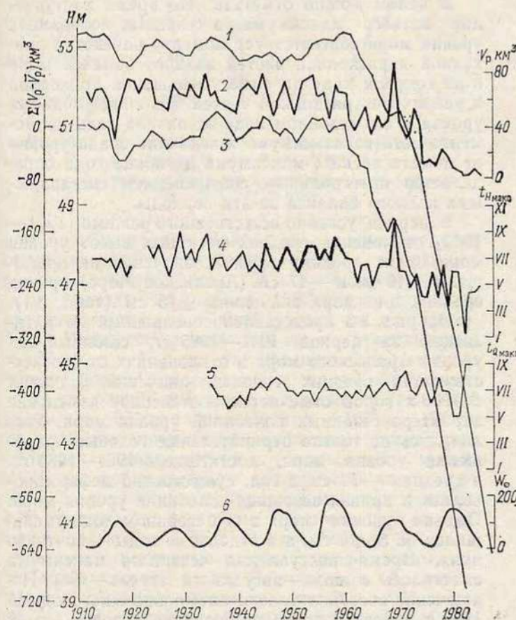
Рис. 3.2. Многолетняя изменчивость некоторых гидрометеорологических и режимобразующих факторов Аральского моря.
