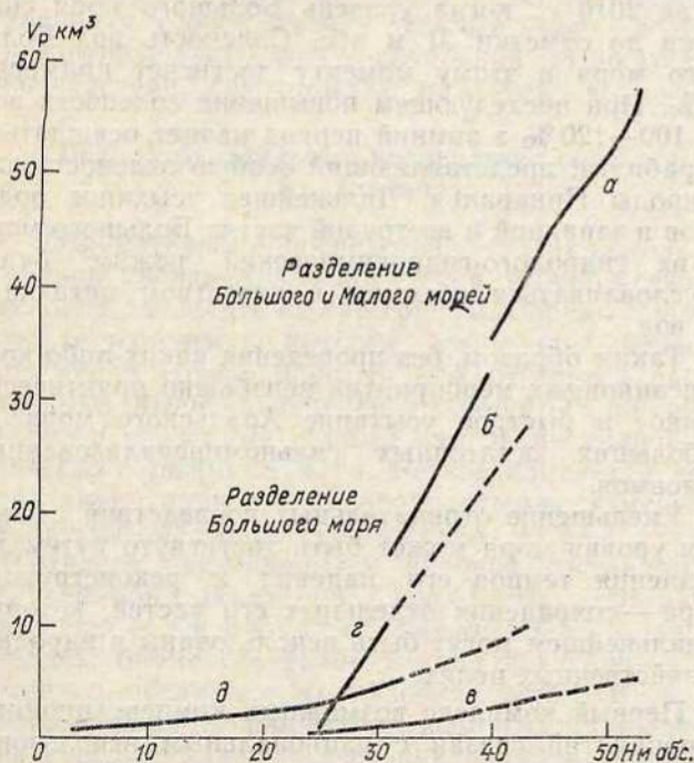
Рис. 19.1. Зависимость уровня равновесия различных частей Аральского моря от объема водного стока.
