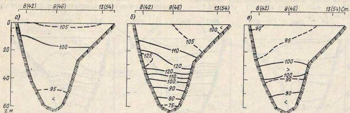
Рис. 16.19. Среднее многолетнее распределение относительного содержания кислорода на разрезе Б весной (а) в 1961—1966 гг., летом (б) в 1966—1970 гг. и осенью (в) в 1961—1966 гг., %.
