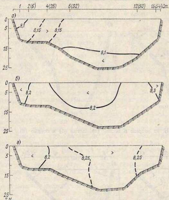
Рис. 16.22. Среднее многолетнее (1961—1965) распределение pH на разрезе А весной (а), летом (б) и осенью (в).
