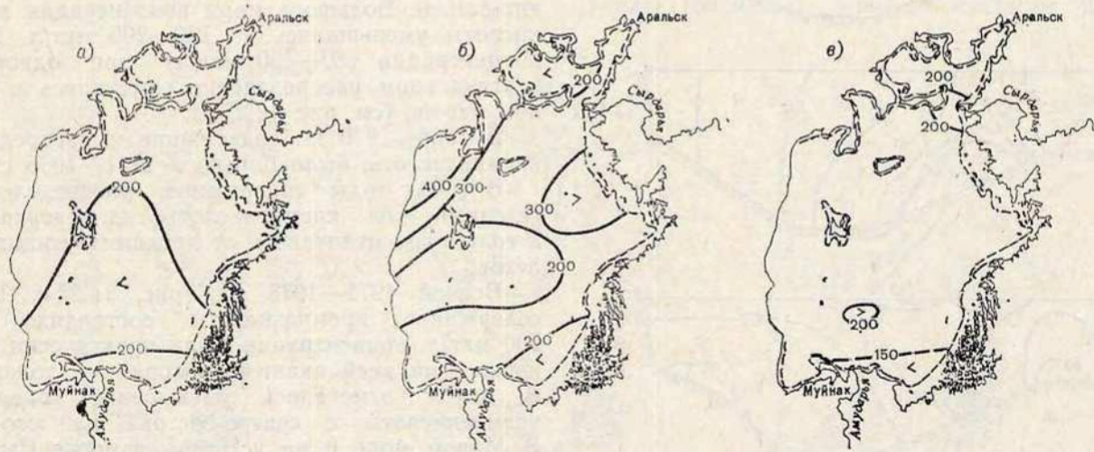
Рис. 14.22. Среднее многолетнее (1971—1975) распределение кремния на поверхности моря весной (а), летом (б) и осенью (в), мкг/л.
