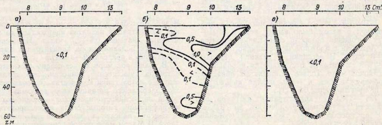
Рис. 14.15. Среднее многолетнее (1971—1975) распределение нитритов на разрезе Б весной (а), летом (б) и осенью (в), мкг/л.
