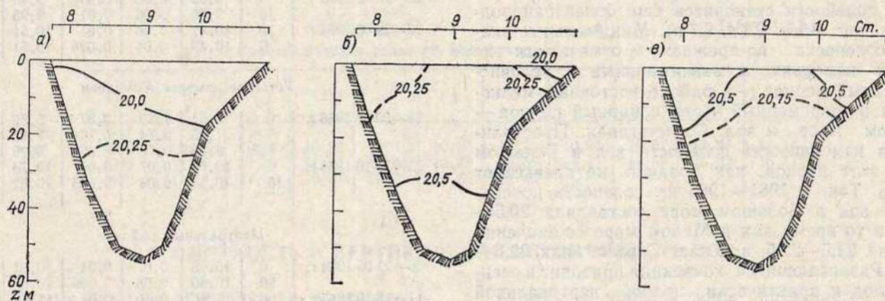
Рис. 8.9. Среднее многолетнее (1981—1985) распределение солености на разрезе Б весной (а), летом (б) и осенью (в), ‰.
