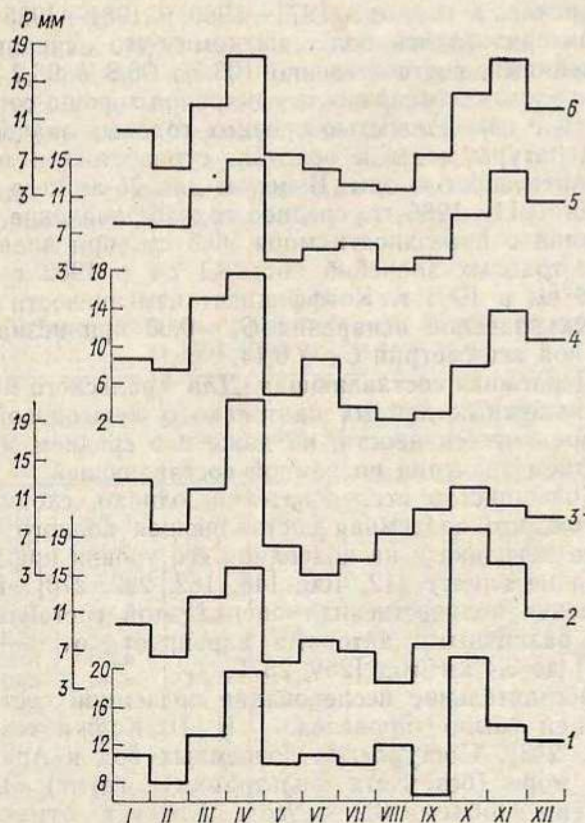
Рис. 4.1. Среднее многолетнее (1961—1985) внутри-годовое распределение осадков в районах береговых и островных гидрометеорологических станций.
