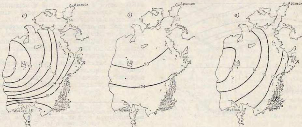
Рис. 5.1. Среднее многолетнее (1950—1960) распределение температуры поверхности моря весной (а), летом (б) и осенью (в), ^{\circ}\text{C} .
