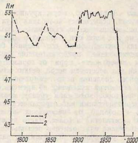
Рис. 3.1. Многолетние изменения уровня Аральского моря.
