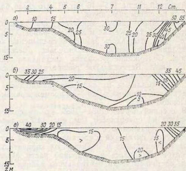
Рис. 14.8. Среднее многолетнее (1981—1985) распределение фосфатов на разрезе А весной (а), летом (б) и осенью (в), мкг/л.
