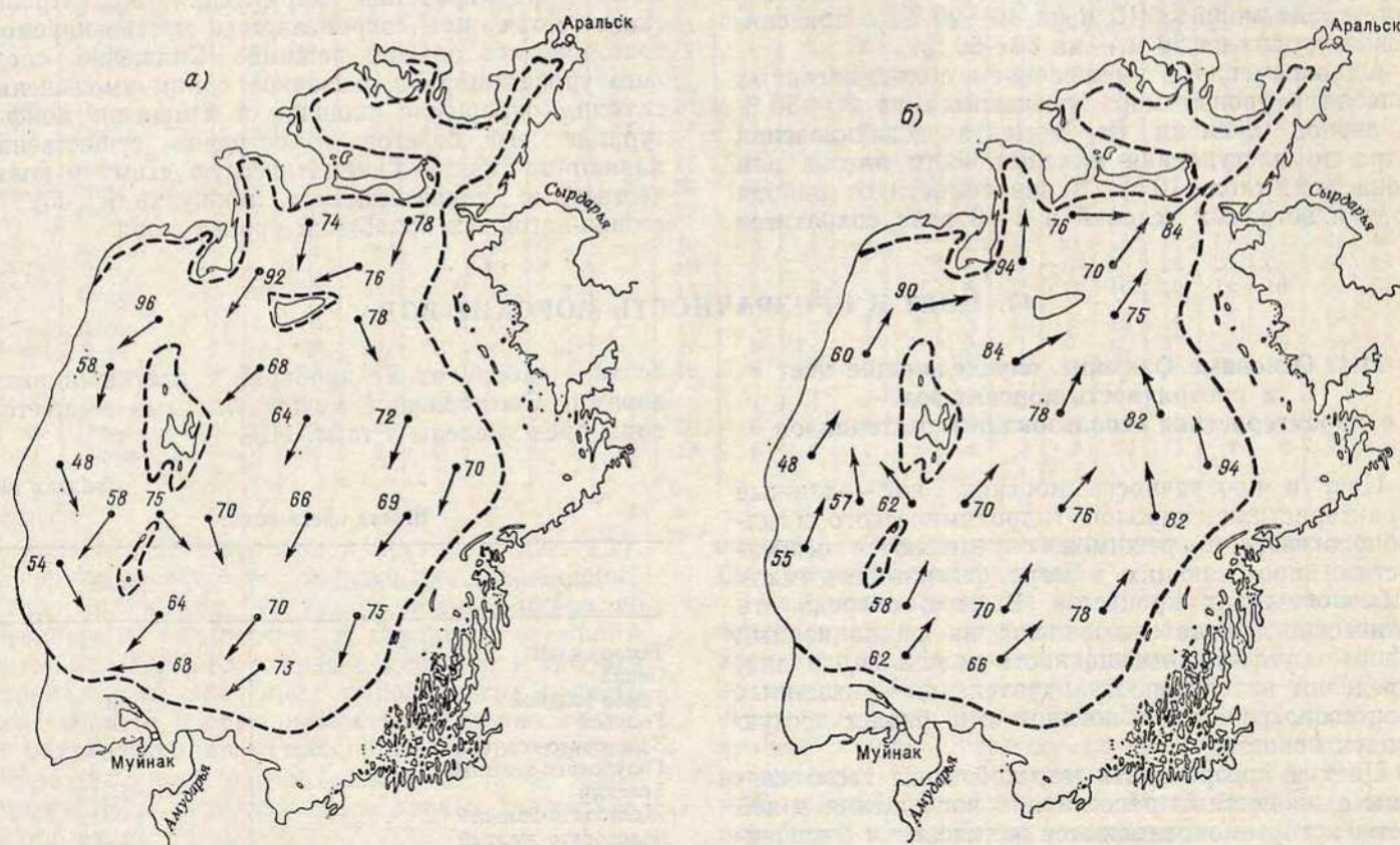
Рис. 10.1. Направление и скорость (см/с) максимального поверхностного течения при северо-восточном (а) и юго-западном (б) ветре 25 м/с и отметке уровня 43 м абс.
