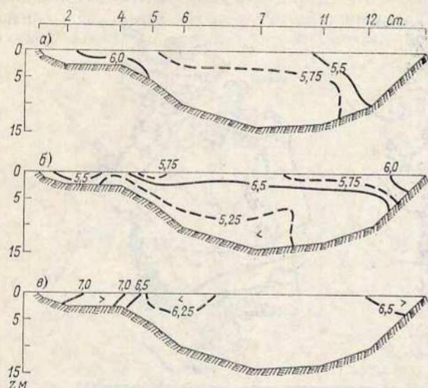
Рис. 16.12. Среднее многолетнее (1981—1985) распределение абсолютного содержания кислорода на разрезе А весной (а), летом (б) и осенью (в), мл/л.
