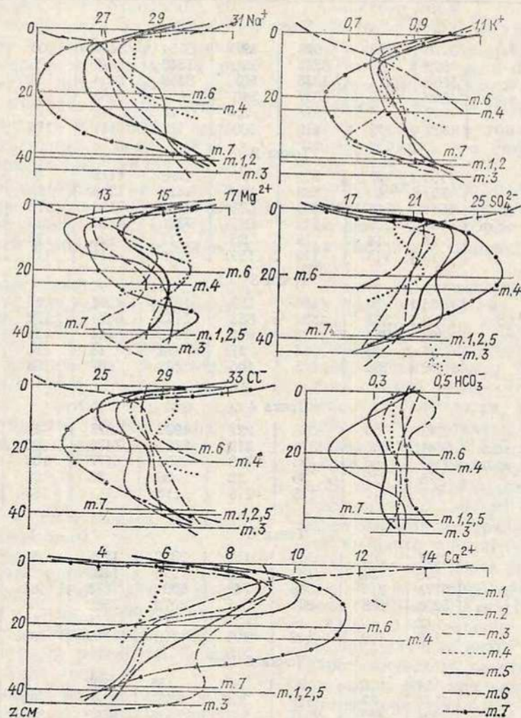
Рис. 17.1. Вертикальное распределение главных ионов солевого состава в системе снег—лед—вода, %.
