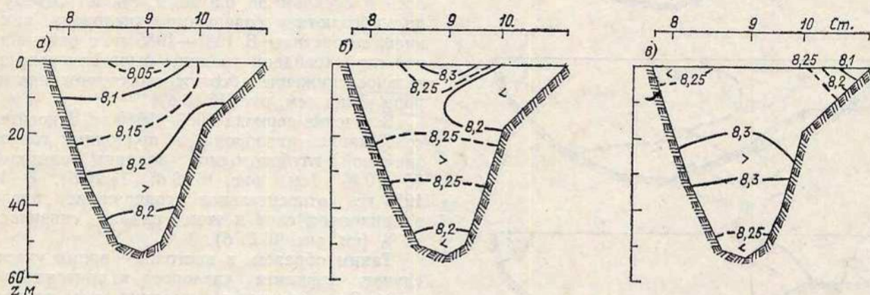
Рис. 16.27. Среднее многолетнее (1981—1985) распределение рН на разрезе Б весной (а), летом (б) и осенью (в).
