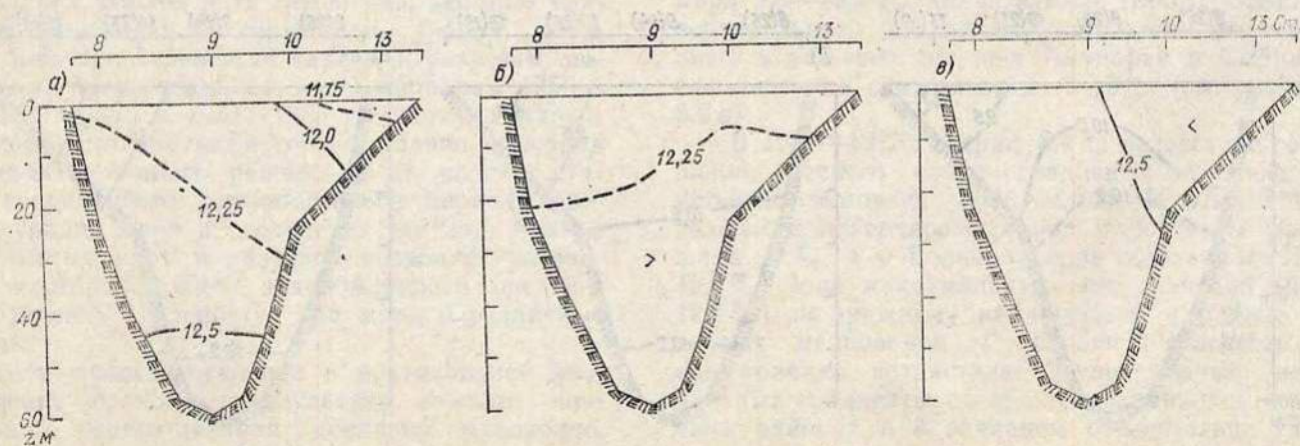
Рис. 8.6. Среднее многолетнее (1971—1975) распределение солености на разрезе Б весной (а), летом (б) и осенью (в), ‰.
