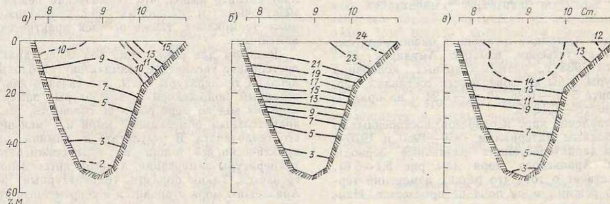
Рис. 5.6. Среднее многолетнее (1976—1985) распределение температуры воды на разрезе В весной (а), летом (б) и осенью (в), °С.
