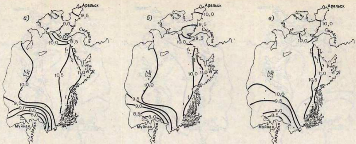
Рис. 8.1. Среднее многолетнее (1956—1960) распределение солёности на поверхности моря весной (а), летом (б) и осенью (в), ‰.
