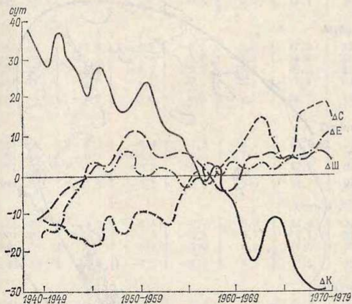
Рис. 2.1. Многолетние изменения 10-летних скользящих средних отклонений от нормы типов циркуляции по М. Х. Байдалу.
