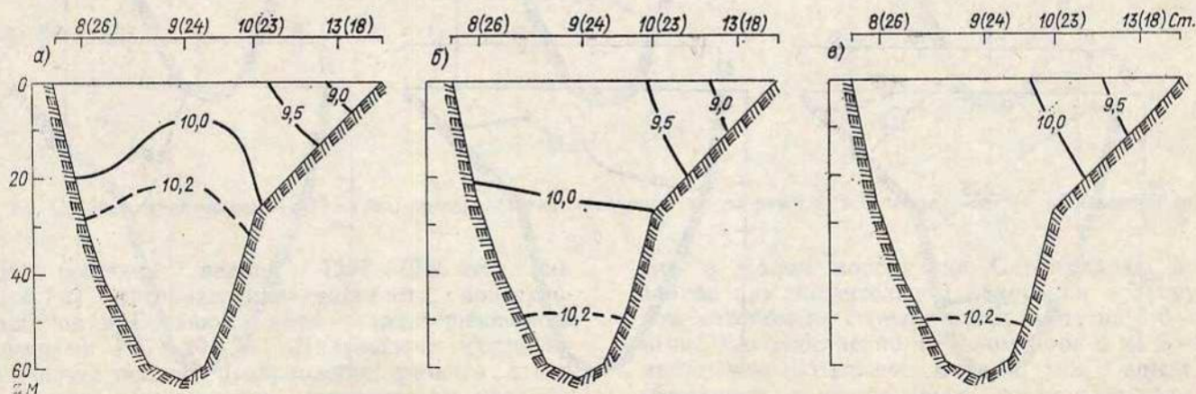
Рис. 8.3. Среднее многолетнее (1956—1960) распределение солёности на разрезе Б весной (а), летом (б) и осенью (в), ‰.
