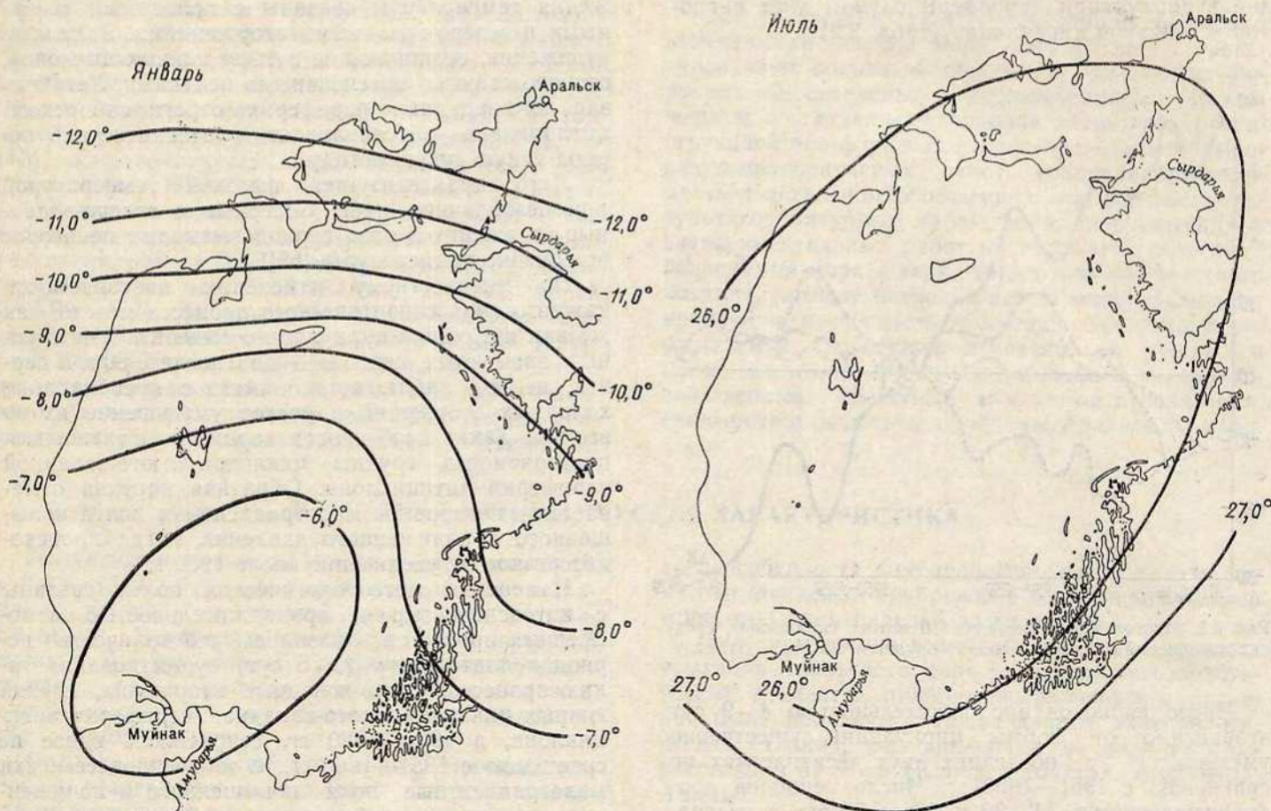
Рис. 2.2. Среднее многолетнее распределение температуры воздуха в январе и июле, ^{\circ}\text{C} .
