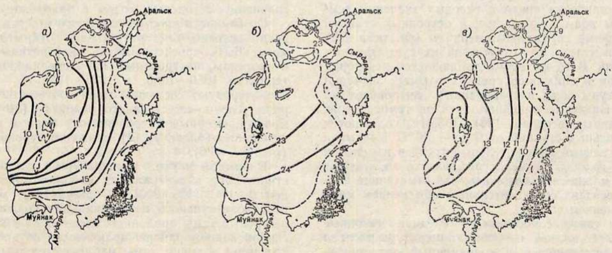
Рис. 5.4. Среднее многолетнее (1976—1985) распределение температуры поверхности моря весной (а), летом (б) и осенью (в), ^{\circ}\text{C} .
