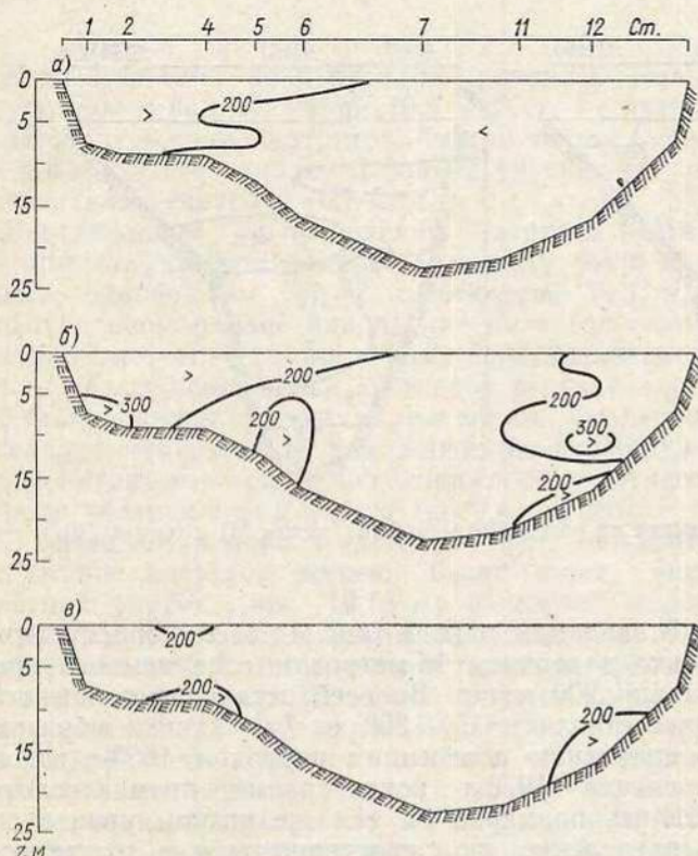
Рис. 14.23. Среднее многолетнее (1971—1975) распределение кремния на разрезе А весной (а), летом (б) и осенью (в), мкг/л.
