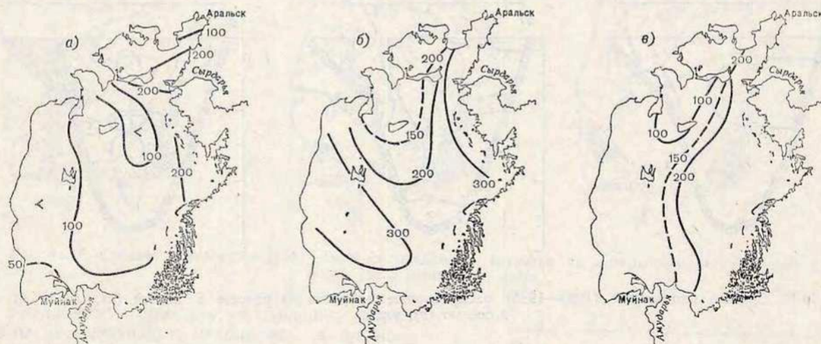
Рис. 14.19. Среднее многолетнее (1961—1965) распределение кремния на поверхности моря весной (а), летом (б) и осенью (в), мкг/л.
