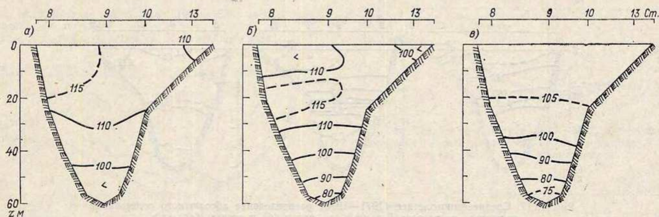
Рис. 16.20. Среднее многолетнее распределение относительного содержания кислорода на разрезе Б весной (а), в 1971—1975 гг., летом (б) 1976—1980 гг. и осенью (в) в 1971—1975 гг., %.
