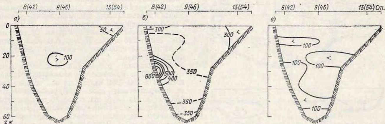
Рис. 14.21. Среднее многолетнее (1961—1965) распределение кремния на разрезе Б весной (а), летом (б) и осенью (в), мкг/л.
