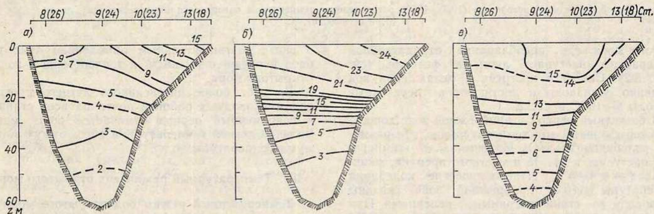
Рис. 5.3. Среднее многолетнее (1950—1960) распределение температуры воды на разрезе Б весной (а), летом (б), осенью (в), ^{\circ}\text{C} .
