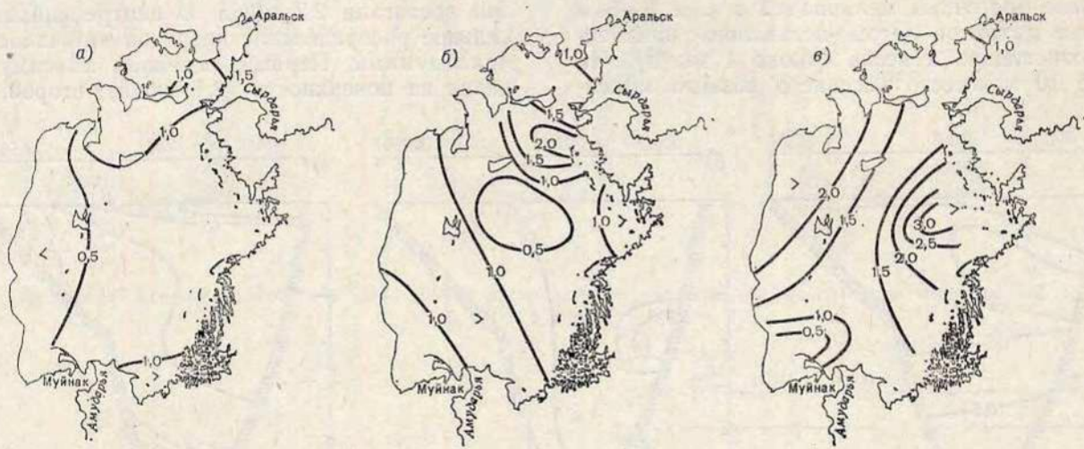
Рис. 14.10. Среднее многолетнее (1961—1965) распределение нитритов на поверхности моря весной (а), летом (б) и осенью (в), мкг/л.
