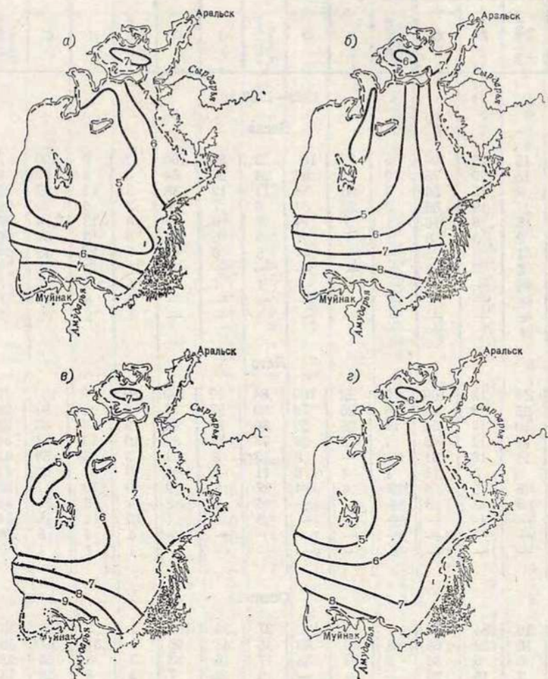
Рис. 11.2. Среднее многолетнее (1961—1985) пространственное распределение цвета морских вод весной (а), летом (б), осенью (в) и в среднем за год (г), балл.
