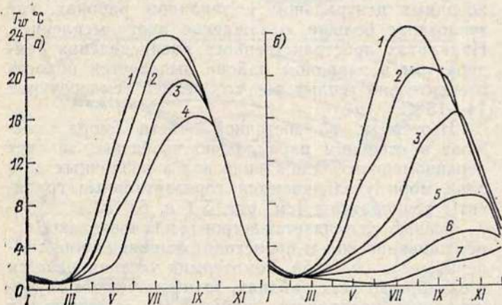
Рис. 5.7. Внутригодовая изменчивость температуры воды на различных глубинах в центральном (а) и западном (б) гидрологических районах.
