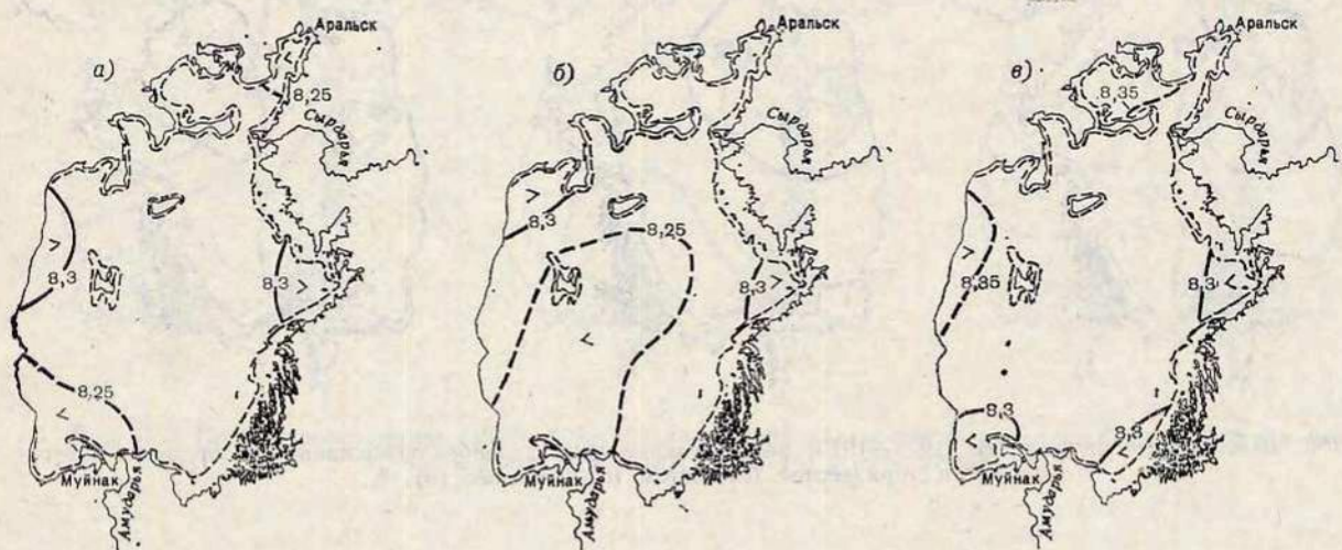
Рис. 16.8. Среднее многолетнее (1971—1975) распределение рН на поверхности моря весной (а), летом (б) и осенью (в).
