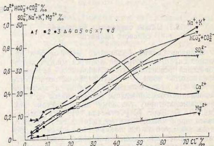
Рис. 12.1. Изменение содержания главных солеобразующих ионов в зависимости от хлорности воды.
