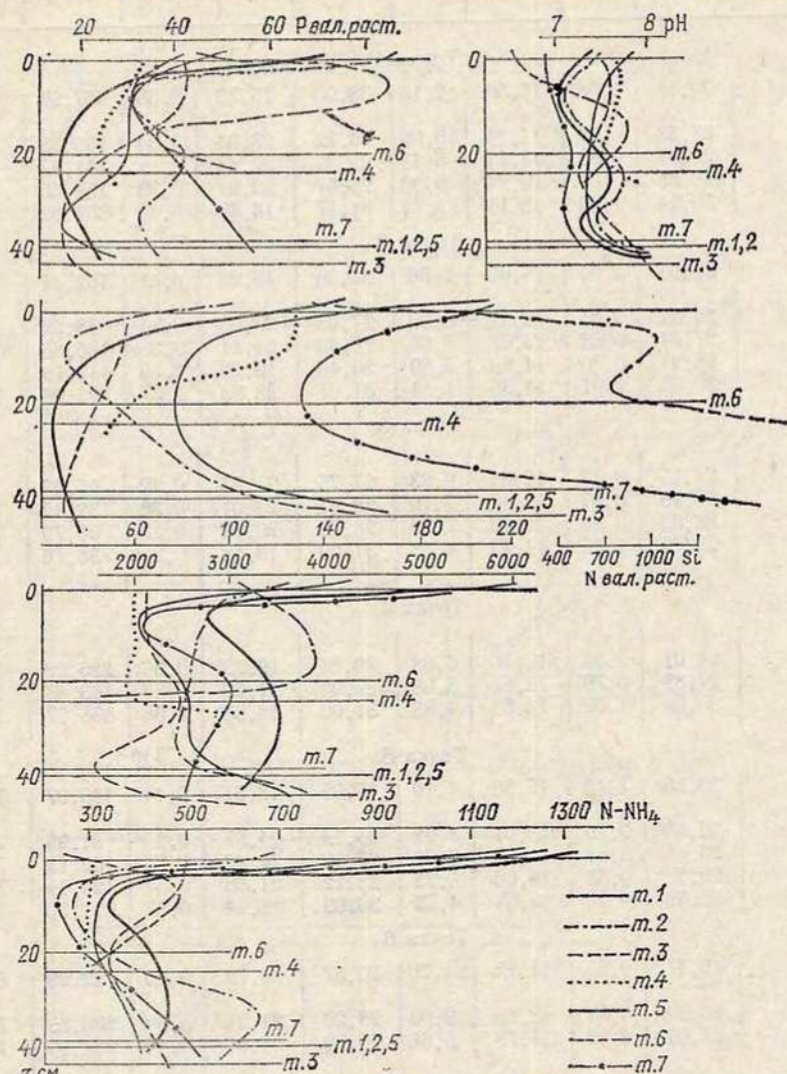
Рис. 17.2. Вертикальное распределение рН и биогенных элементов в системе снег—лед—вода, мкг/л.
