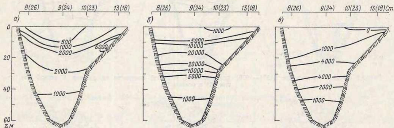
Рис. 9.7. Среднее многолетнее (1956—1960) распределение устойчивости вод ( E \cdot 10^8 ) на разрезе Б весной (а), летом (б) и осенью (в).
