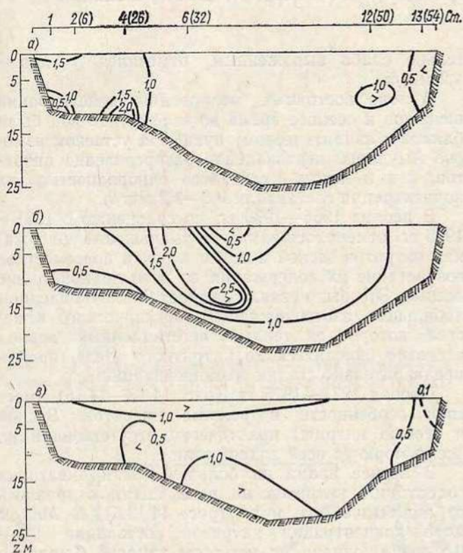
Рис. 14.11. Среднее многолетнее (1961—1965) распределение нитритов на разрезе А весной (а), летом (б) и осенью (в), мкг/л.
