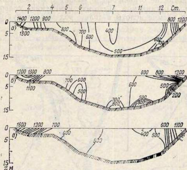
Рис. 14.26 Среднее многолетнее (1981—1985) распределение кремния на разрезе А весной (а), летом (б) и осенью (в), мкг/л.
