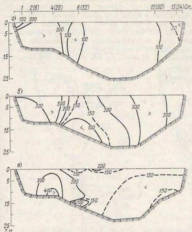
Рис. 14.20. Среднее многолетнее (1961—1965) распределение кремния на разрезе А весной (а), летом (б) и осенью (в), мкг/л.
