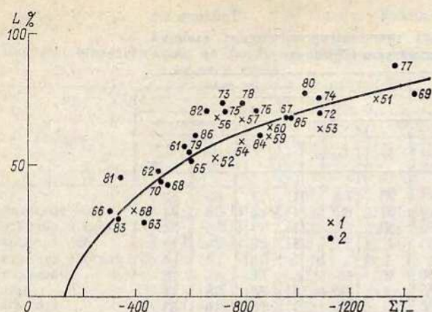
Рис. 6.1. Связь ледовитости моря ( L\% ) с суммой градусо-дней мороза ( \Sigma T_- ).
