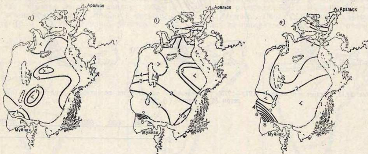
Рис. 14.16. Среднее многолетнее (1981—1985) распределение нитритов на поверхности моря весной (а), летом (б) и осенью (в), мкг/л.
