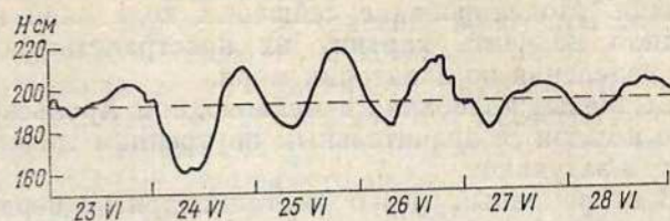
Рис. 3.5. Приливные колебания уровня моря в районе ст. Аральское Море. Июнь 1961 г.
