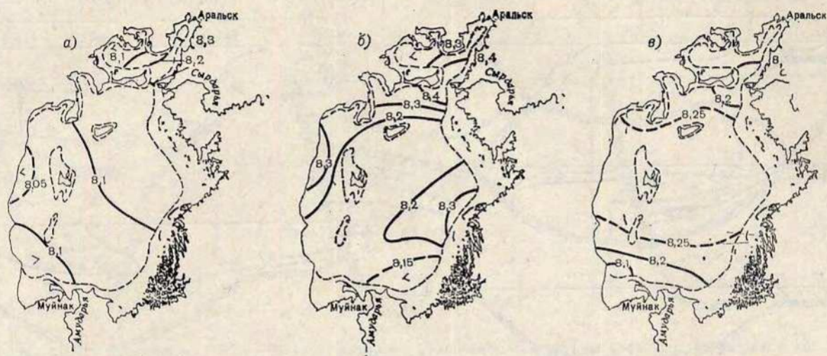
Рис. 16.9. Среднее многолетнее (1981—1985) распределение рН на поверхности моря весной (а), летом (б) и осенью (в).
