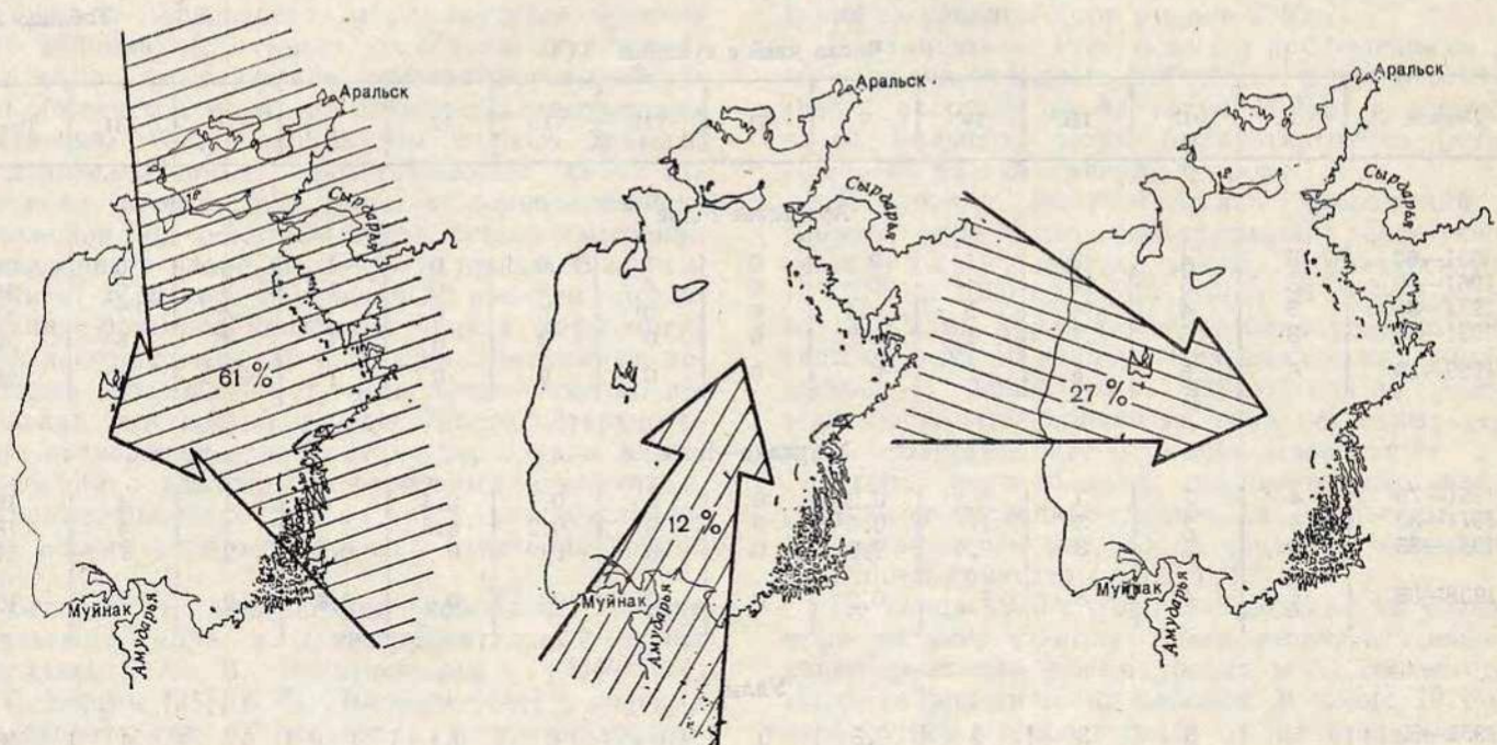
Рис. 2.7. Повторяемость различных направлений ветра во время пыльных бурь и пыльного поземка.
