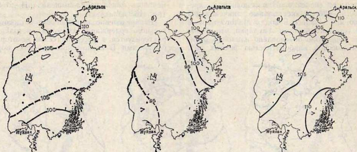
Рис. 16.4. Среднее многолетнее распределение относительного содержания кислорода на поверхности моря весной (а), летом (б) в 1961—1965 гг. и осенью (в) в 1966—1970 гг., %.
