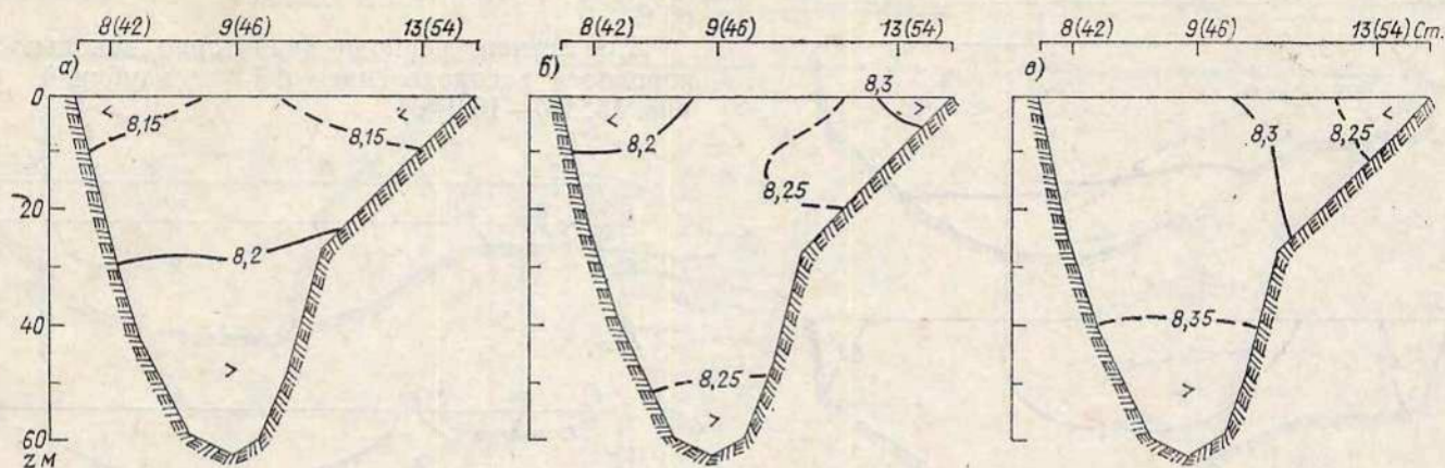
Рис. 16.25. Среднее многолетнее (1961—1965) распределение рН на разрезе Б весной (а), летом (б) и осенью (в).
