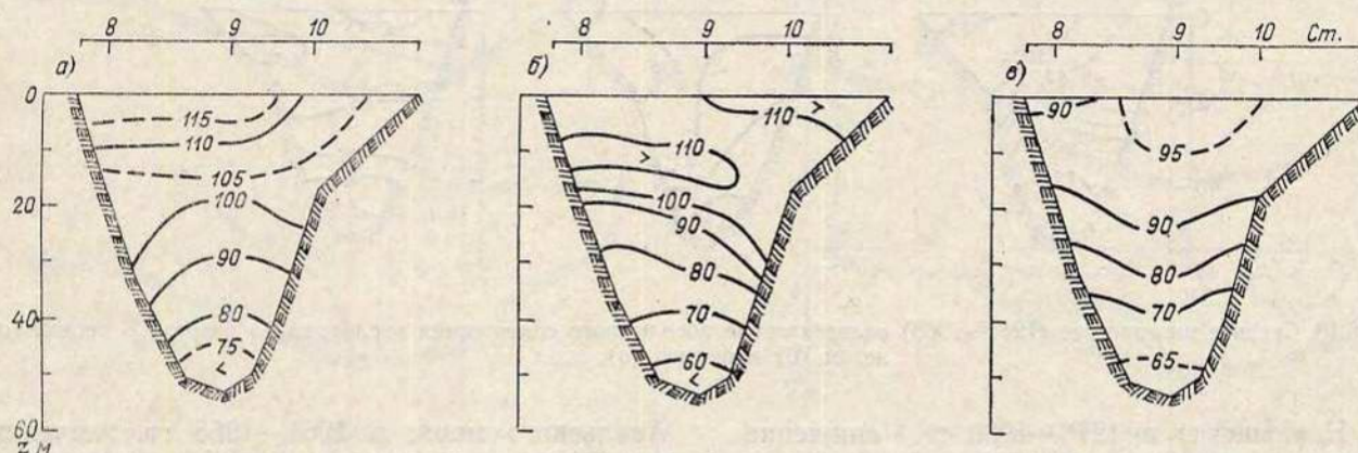
Рис. 16.21. Среднее многолетнее (1981—1985) распределение относительного содержания кислорода на разрезе Б весной (а), летом (б) и осенью (в), %.
