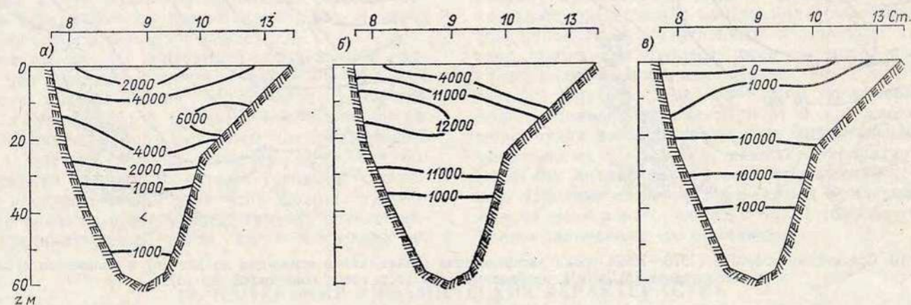
Рис. 9.9. Среднее многолетнее (1976—1980) распределение устойчивости вод ( E \cdot 10^8 ) на разрезе Б весной (а), летом (б) и осенью (в).
