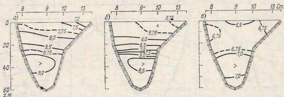
Рис. 16.17. Среднее многолетнее (1971—1975) распределение абсолютного содержания кислорода на разрезе Б весной (а), летом (б) и осенью (в), мл/л.
