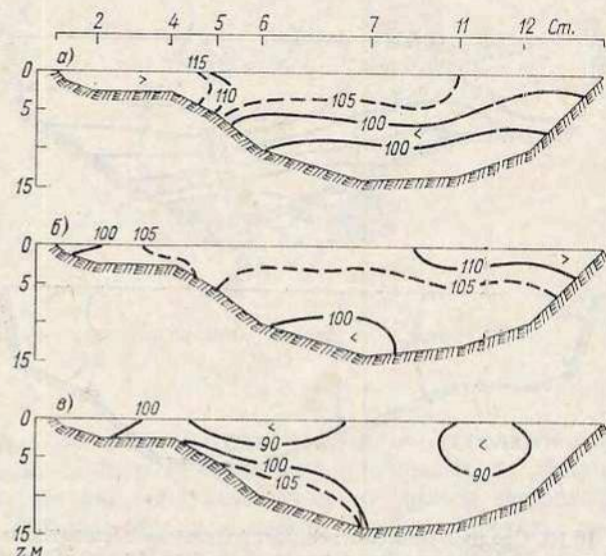
Рис. 16.15. Среднее многолетнее (1981—1985) распределение относительного содержания кислорода на разрезе А весной (а), летом (б) и осенью (в), %.
