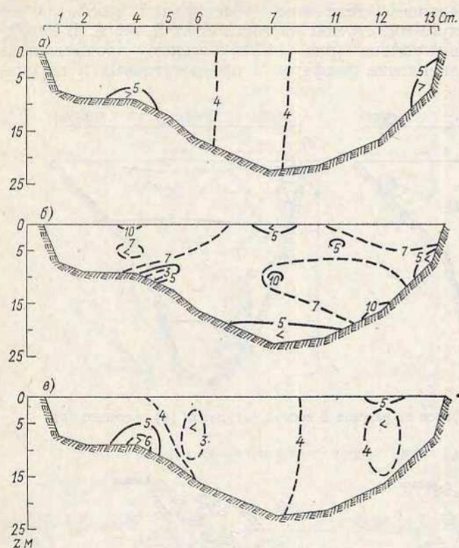
Рис. 14.5. Среднее многолетнее (1971—1975) распределение фосфатов на разрезе А весной (а), летом (б) и осенью (в), мкг/л.
