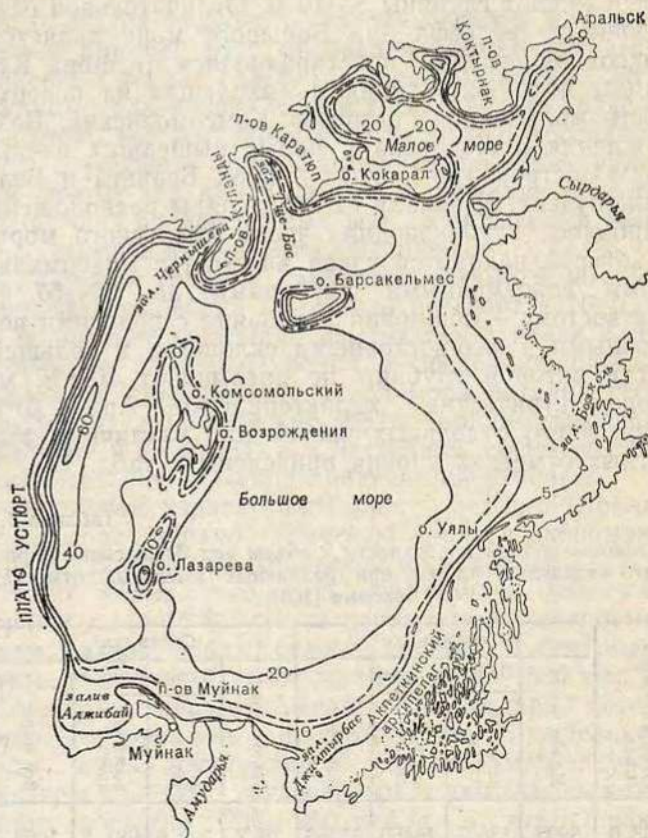
Рис. 1.1. Распределение глубин в Аральском море при отметке уровня 53 м абс.
