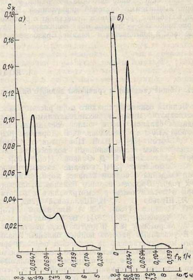
Рис. 3.6. Спектры ежечасных уровней моря в районе станций Аральское Море (а) и Тигровый (б). Июнь 1961 г.
