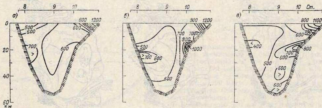
Рис. 14.27. Среднее многолетнее (1981—1985) распределение кремния на разрезе Б весной (а), летом (б) и осенью (в), мкг/л.
