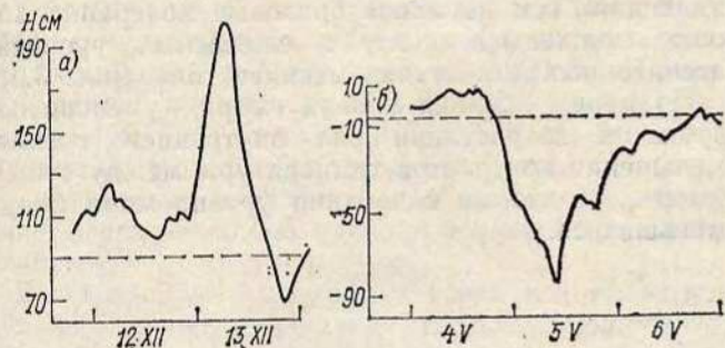
Рис. 3.4. Сгонно-нагонные колебания уровня моря в районе ст. Аральское Море.
