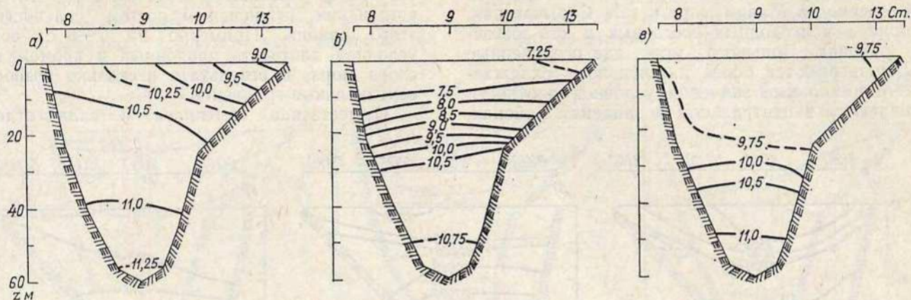
Рис. 9.4. Среднее многолетнее (1971—1975) распределение условной плотности на разрезе Б весной (а), летом (б) и осенью (в).
