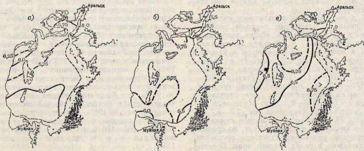
Рис. 16.3. Среднее многолетнее (1981—1985) распределение абсолютного содержания кислорода на поверхности моря весной (а), летом (б) и осенью (в), мл/л.
