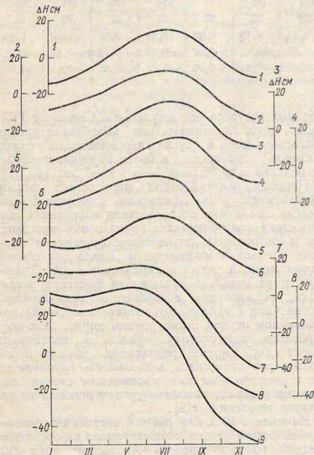
Рис. 3.3. Кривые сезонных колебаний уровня Аральского моря для отдельных пятилеток.
