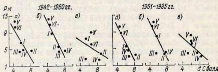
Рис. 11.7. Зависимости средних сезонных значений прозрачности морской воды от ее цвета для характерных периодов.
