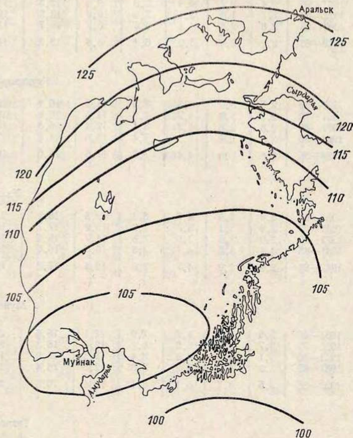
Рис. 2.5. Среднее многолетнее распределение годового количества осадков, мм.
