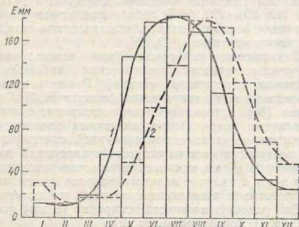
Рис. 4.2. Среднее многолетнее внутригодовое распределение испарения.
