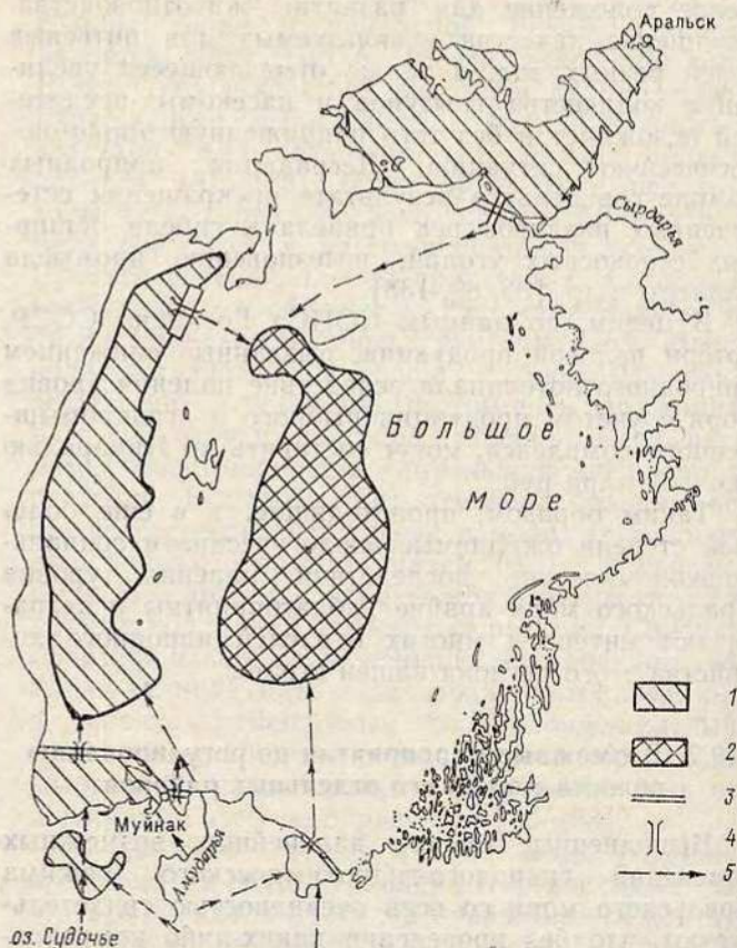
Рис. 19.2. Схема возможной реконструкции Аральского моря.
