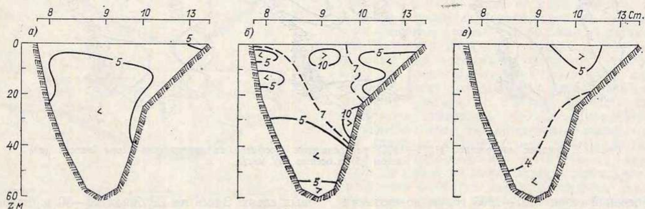
Рис. 14.6. Среднее многолетнее (1971—1975) распределение фосфатов на разрезе Б весной (а), летом (б) и осенью (в), мкг/л.
