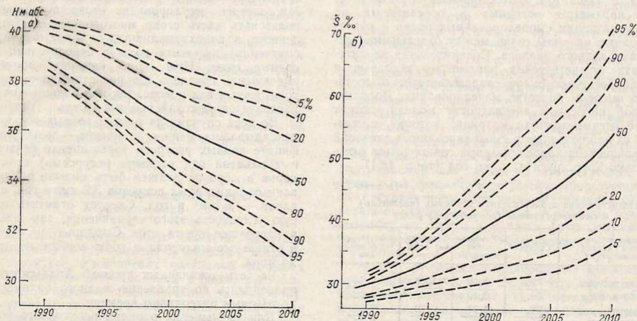
Рис. 18.1. Возможные изменения уровня (а) и солёности (б) Аральского моря при осуществлении одного из вариантов безвозвратных изъятий стока в его бассейне.
