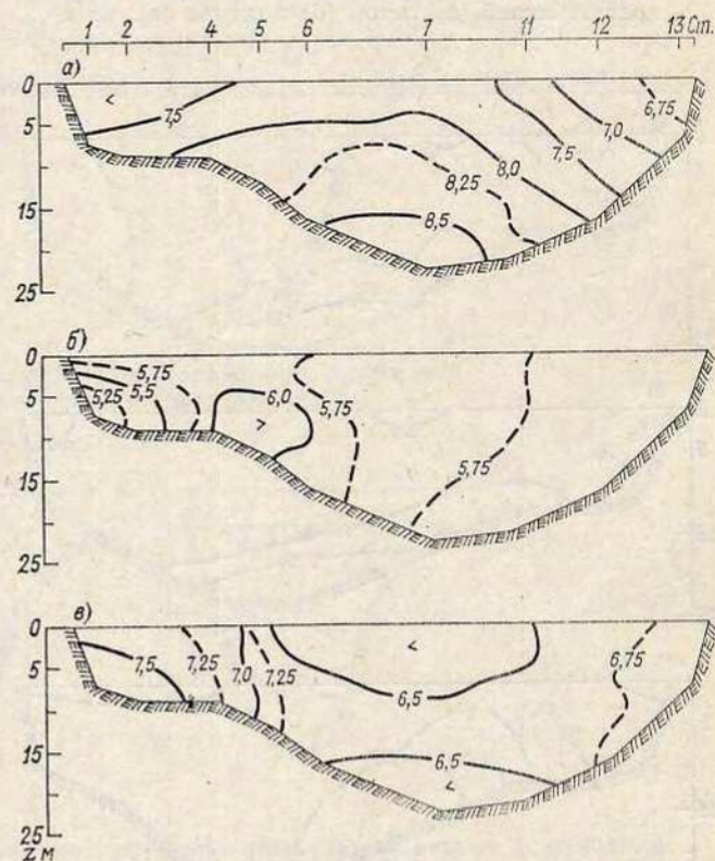
Рис. 16.11. Среднее многолетнее (1971—1975) распределение абсолютного содержания кислорода на разрезе А весной (а), летом (б) и осенью (в), мл/л.
