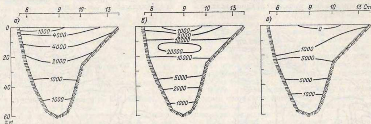
Рис. 9.8. Среднее многолетнее (1971—1975) распределение устойчивости вод ( E \cdot 10^8 ) на разрезе Б весной (а), летом (б) и осенью (в).
