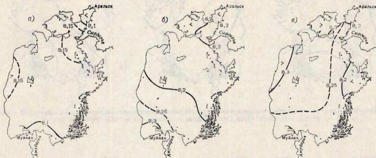
Рис. 16.7. Среднее многолетнее (1961—1965) распределение рН на поверхности моря весной (а), летом (б) и осенью (в).
