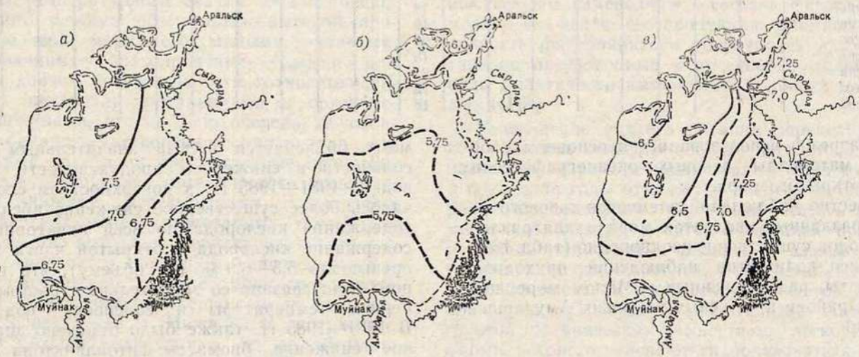
Рис. 16.2. Среднее многолетнее (1971—1975) распределение абсолютного содержания кислорода на поверхности моря весной (а), летом (б) и осенью (в), мл/л.
