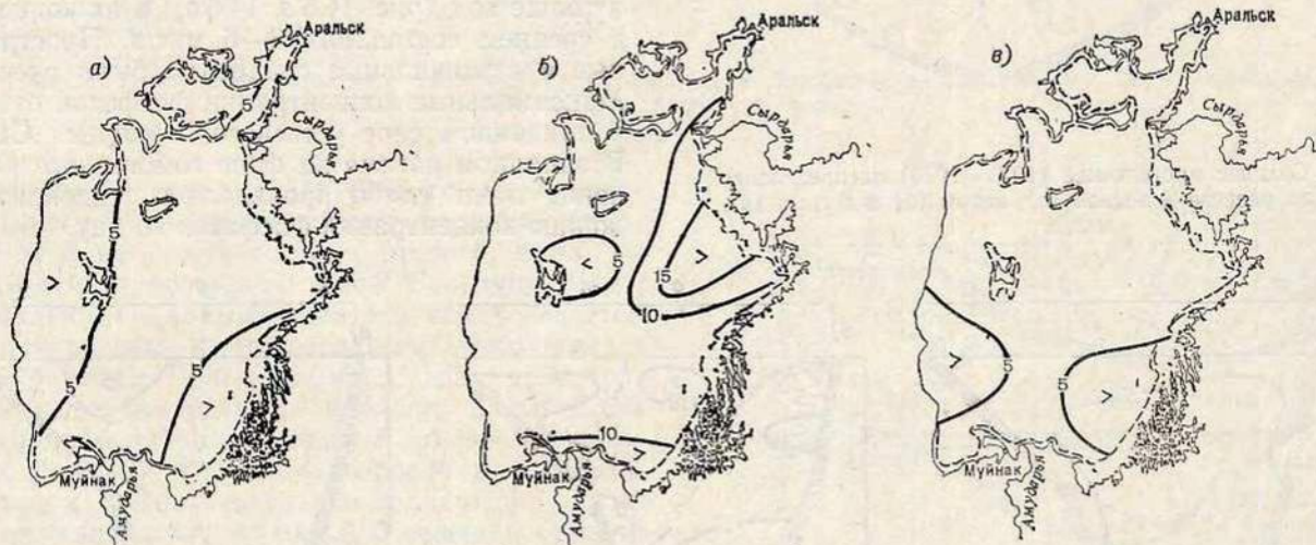
Рис. 14.4. Среднее многолетнее (1971—1975) распределение фосфатов на поверхности моря весной (а), летом (б) и осенью (в), мкг/л.
