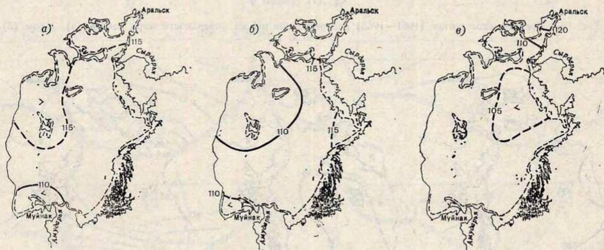
Рис. 16.5. Среднее многолетнее (1971—1975) распределение относительного содержания кислорода на поверхности моря весной (а), летом (б) и осенью (в), %.
