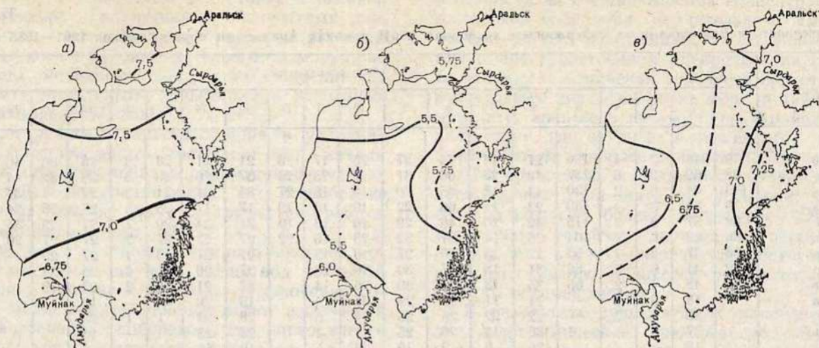
Рис. 16.1. Среднее многолетнее распределение абсолютного содержания кислорода на поверхности моря весной (а), летом (б) в 1961—1965 гг. и осенью (в) в 1966—1970 гг., мл/л (‰ по объему).
