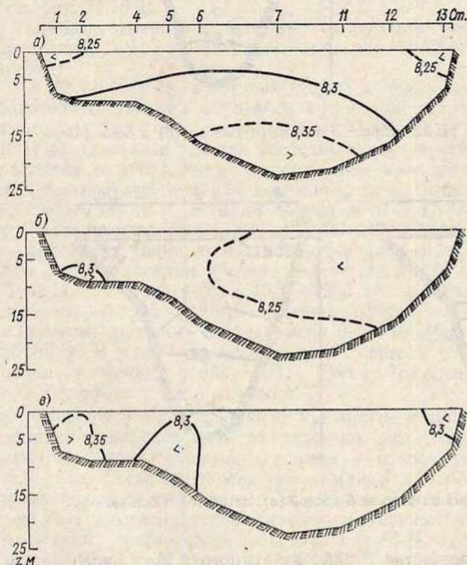
Рис. 16.23. Среднее многолетнее (1971—1975) распределение pH на разрезе А весной (а), летом (б) и осенью (в).
