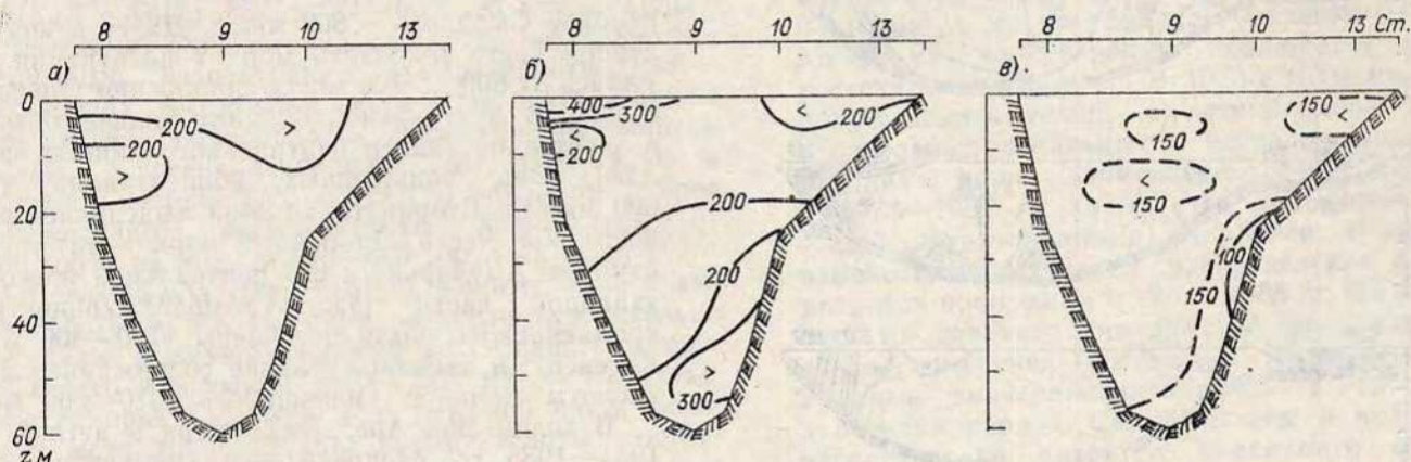
Рис. 14.24. Среднее многолетнее (1971—1975) распределение кремния на разрезе Б весной (а), летом (б) и осенью (в), мкг/л.
