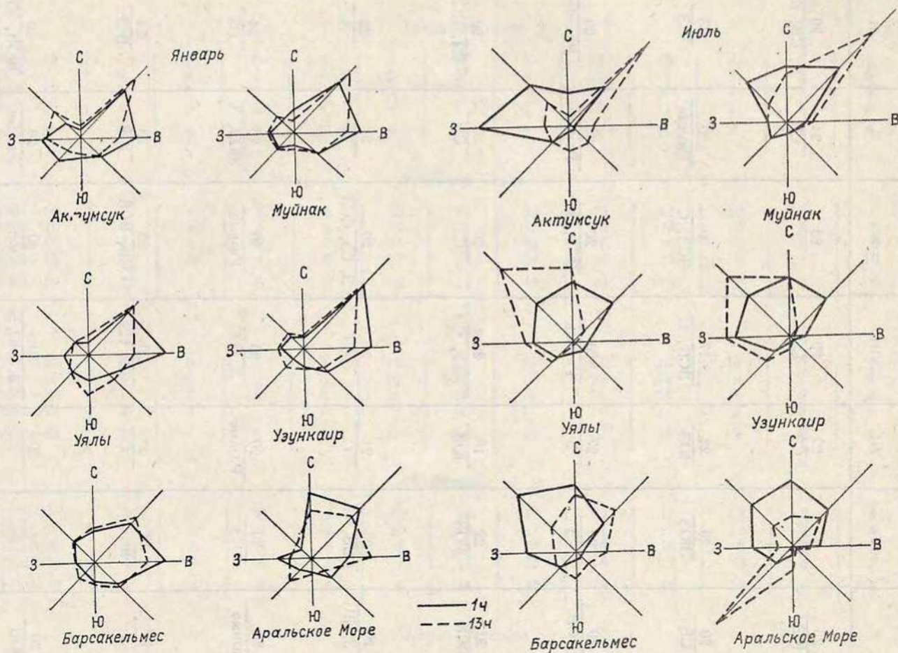
Рис. 2.6. Средние многолетние розы ветра.
