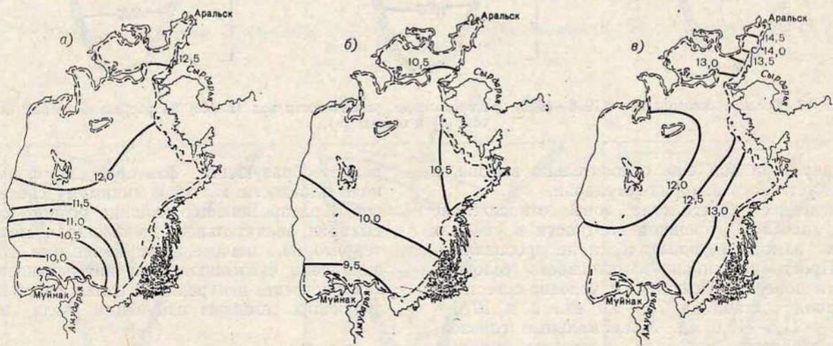
Рис. 9.5. Среднее многолетнее (1976—1980) распределение условной плотности на поверхности моря весной (а), летом (б) и осенью (в).
