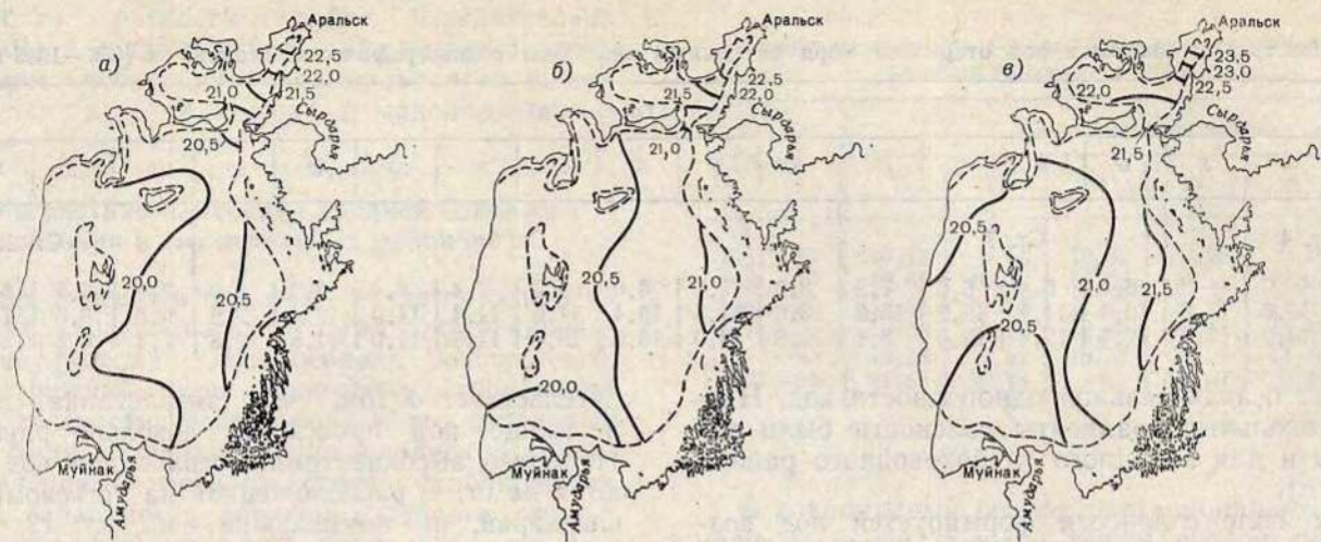
Рис. 8.7. Среднее многолетнее (1981—1985) распределение солености на поверхности моря весной (а), летом (б) и осенью (в), ‰.
