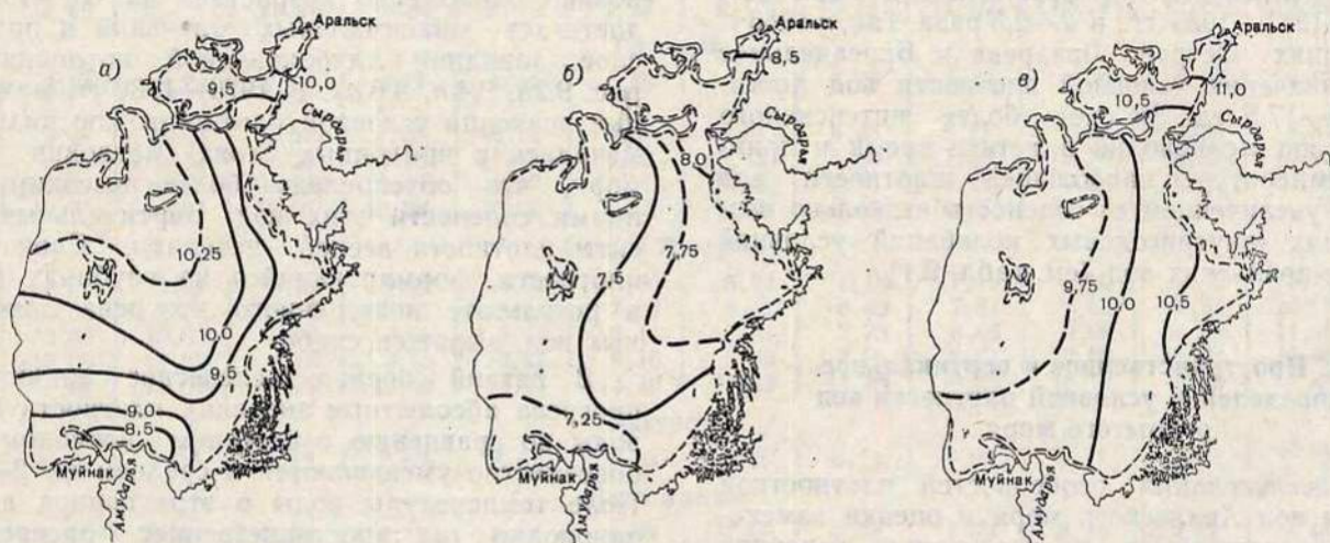
Рис. 9.3. Среднее многолетнее (1971—1975) распределение условной плотности на поверхности моря весной (а), летом (б) и осенью (в).
