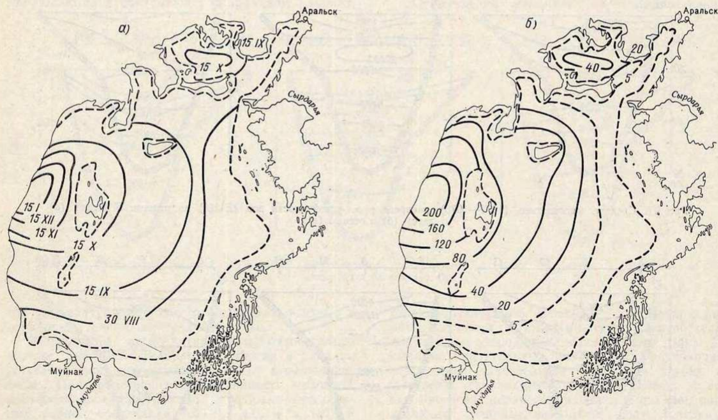
Рис. 9.10. Средние многолетние (1976—1982) сроки распределения осенне-зимней конвекции до дна (а) и количество суммарной теплоотдачи (МДж/м²), необходимой для достижения конвекцией дна (б).
