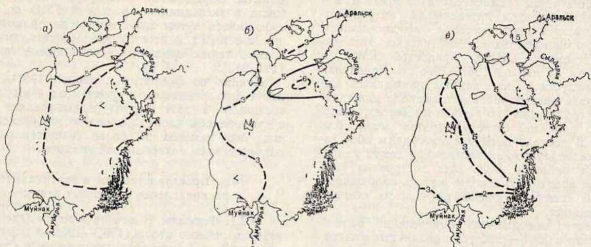
Рис. 14.1. Среднее многолетнее (1961—1965) распределение фосфатов на поверхности моря весной (а), летом (б) и осенью (в), мкг/л.
