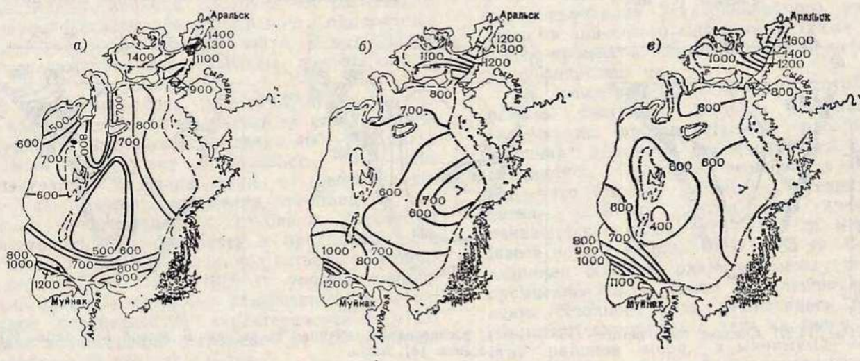
Рис. 14.25. Среднее многолетнее (1981—1985) распределение кремния на поверхности моря весной (а), летом (б) и осенью (в), мкг/л.
