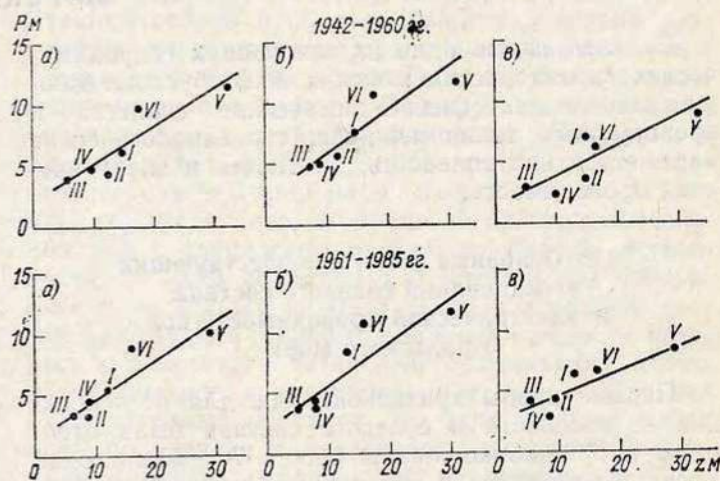
Рис. 11.6. Зависимости средних сезонных значений прозрачности морской воды от глубины моря для характерных периодов.
