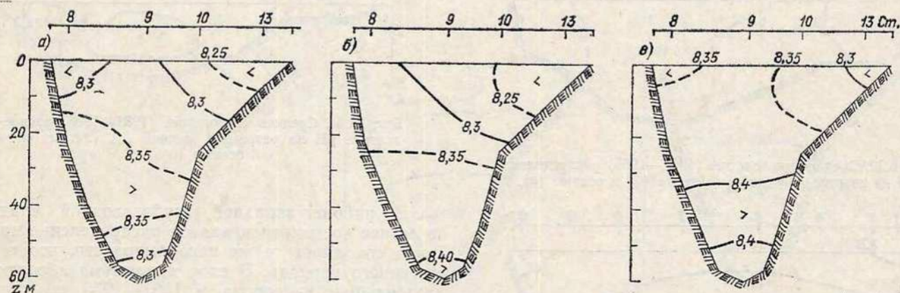
Рис. 16.26. Среднее многолетнее (1971—1975) распределение рН на разрезе Б весной (а), летом (б) и осенью (в).
