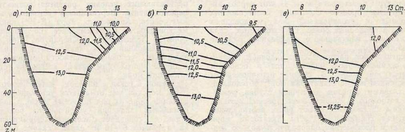
Рис. 9.6. Среднее многолетнее (1976—1980) распределение условной плотности на разрезе Б весной (а), летом (б) и осенью (в).
