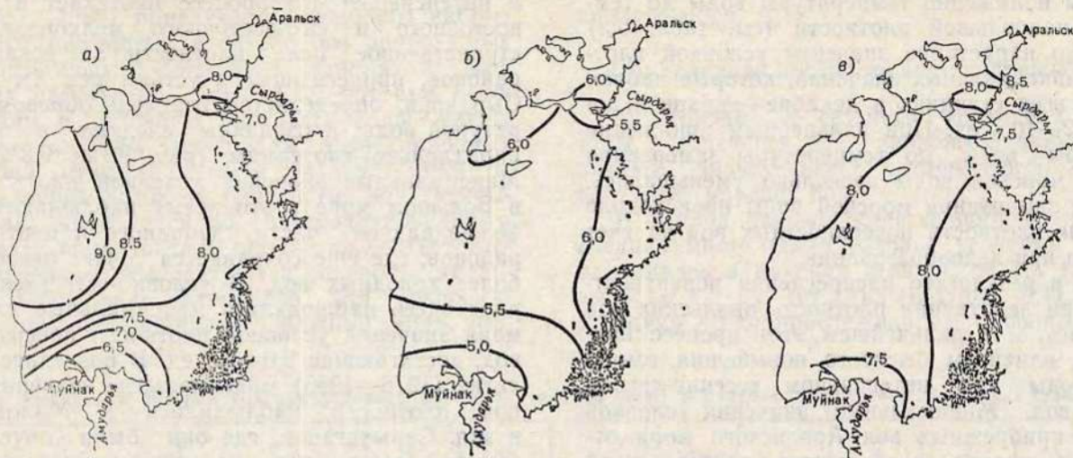
Рис. 9.1. Среднее многолетнее (1956—1960) распределение условной плотности на поверхности моря весной (а), летом (б) и осенью (в).
