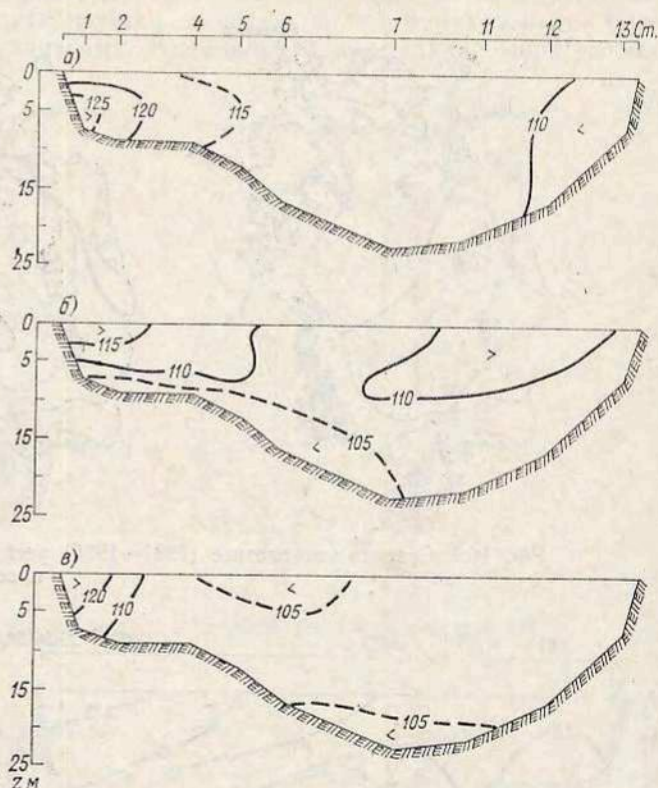
Рис. 16.14. Среднее многолетнее (1971—1975) распределение относительного содержания кислорода на разрезе А весной (а), летом (б) и осенью (в), %.
