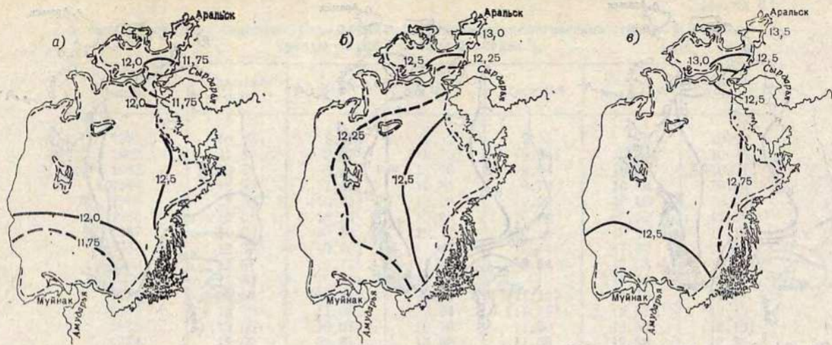
Рис. 8.4. Среднее многолетнее (1971—1975) распределение солености на поверхности моря весной (а), летом (б) и осенью (в), ‰.
