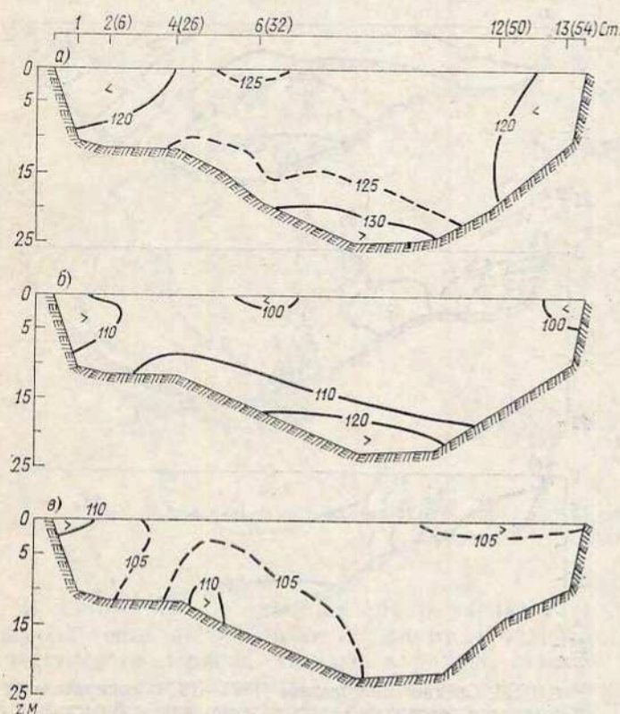
Рис. 16.13. Среднее многолетнее (1966—1970) распределение относительного содержания кислорода на разрезе А весной (а), летом (б) и осенью (в), %.
