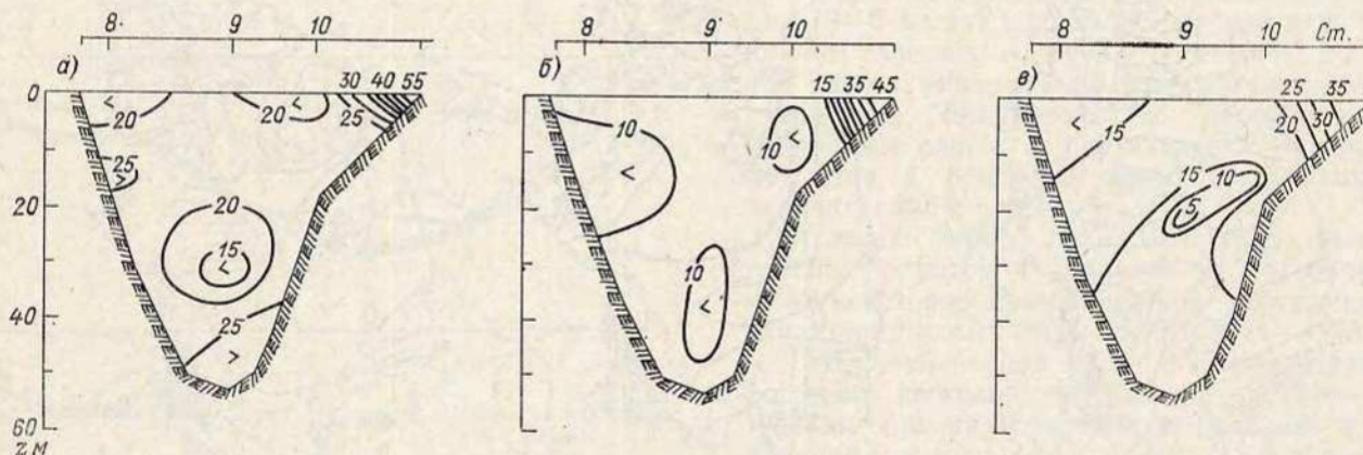
Рис. 14.9. Среднее многолетнее (1981—1985) распределение фосфатов на разрезе Б весной (а), летом (б) и осенью (в), мкг/л.
