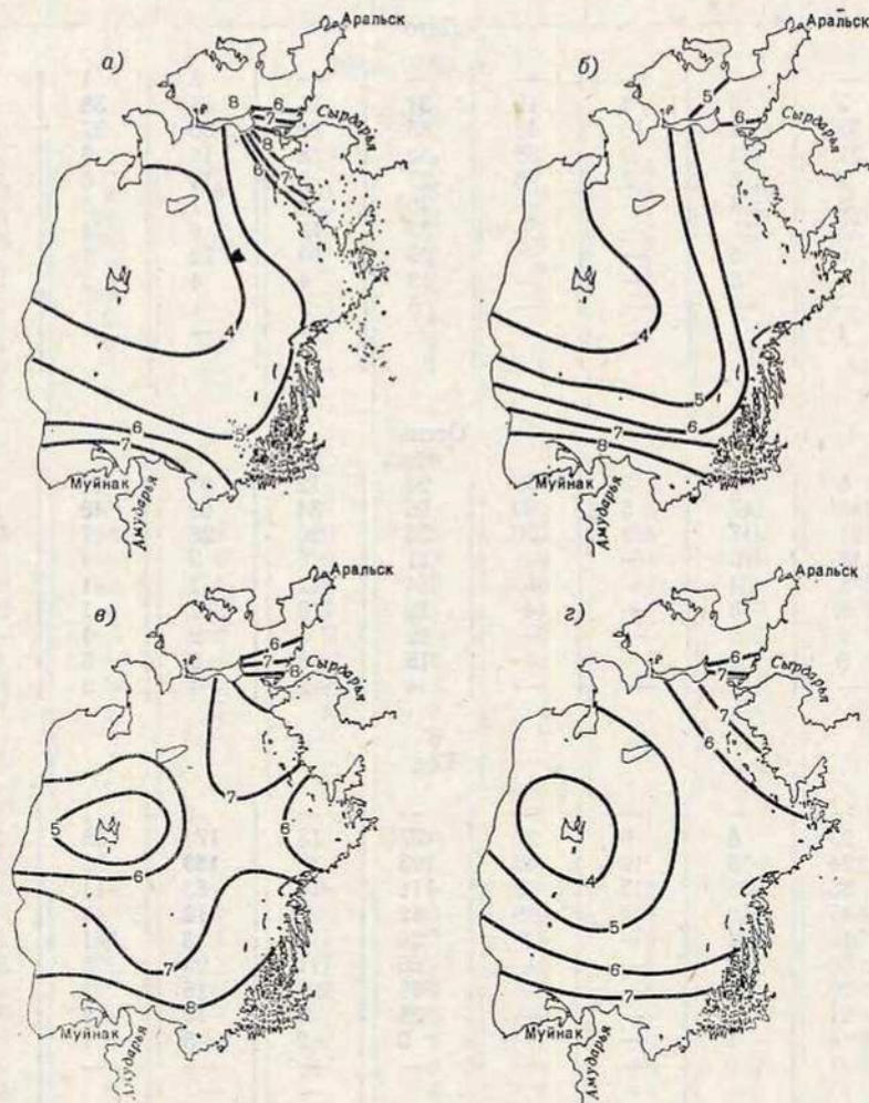
Рис. 11.1. Среднее многолетнее (1942—1960) пространственное распределение цвета морских вод весной (а), летом (б), осенью (в) и в среднем за год (г), балл.
