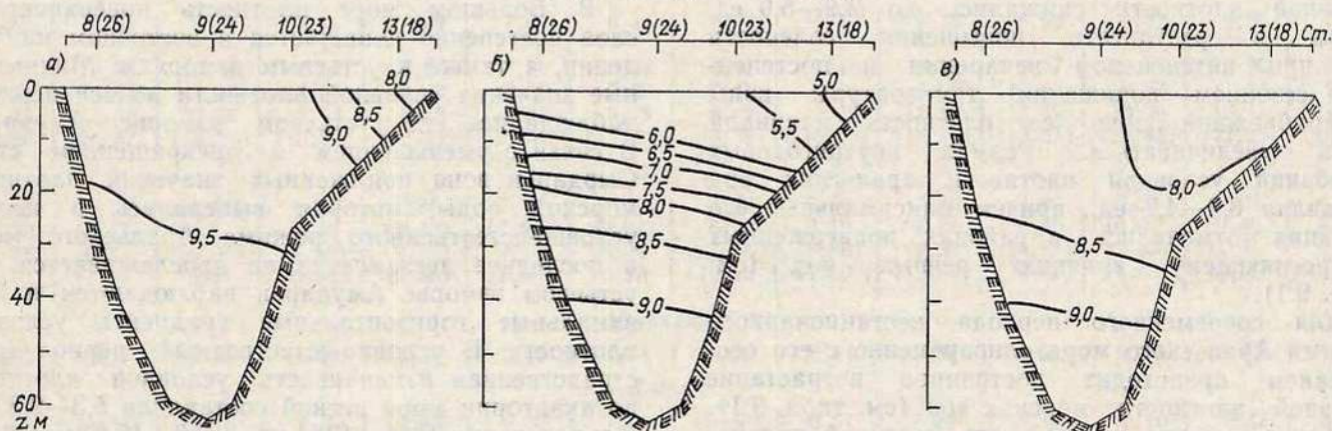
Рис. 9.2. Среднее многолетнее (1956—1960) распределение условной плотности на разрезе Б весной (а), летом (б) и осенью (в).
