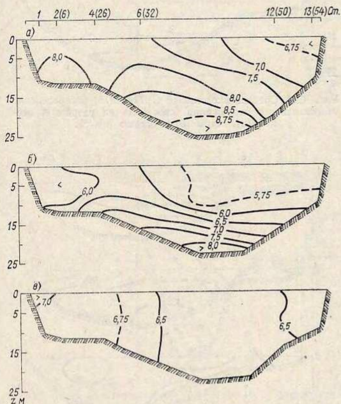
Рис. 16.10. Среднее многолетнее распределение абсолютного содержания кислорода на разрезе А весной (а) в 1961—1966 гг., летом (б) и осенью (в) в 1966—1970 гг., мл/л.
