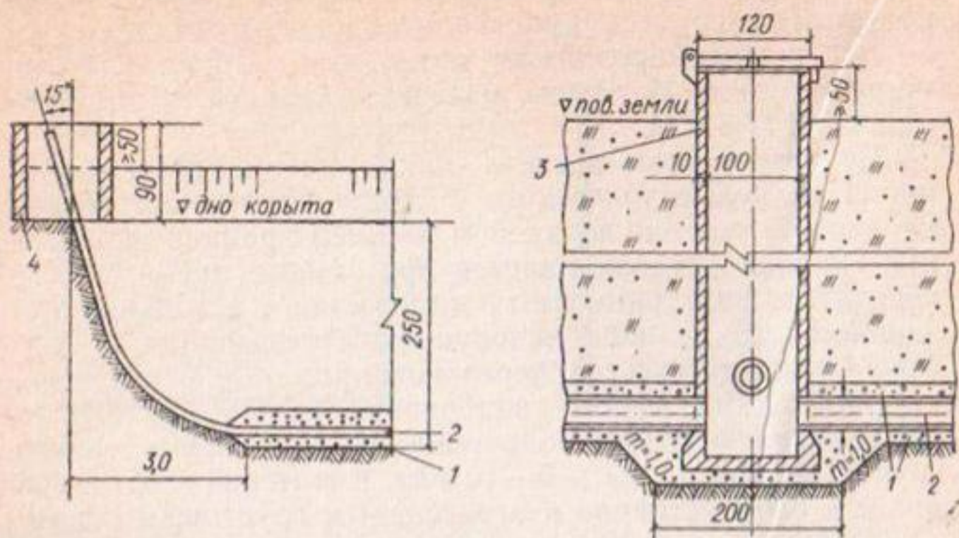
Рис. 7. Дренажные колодцы:
