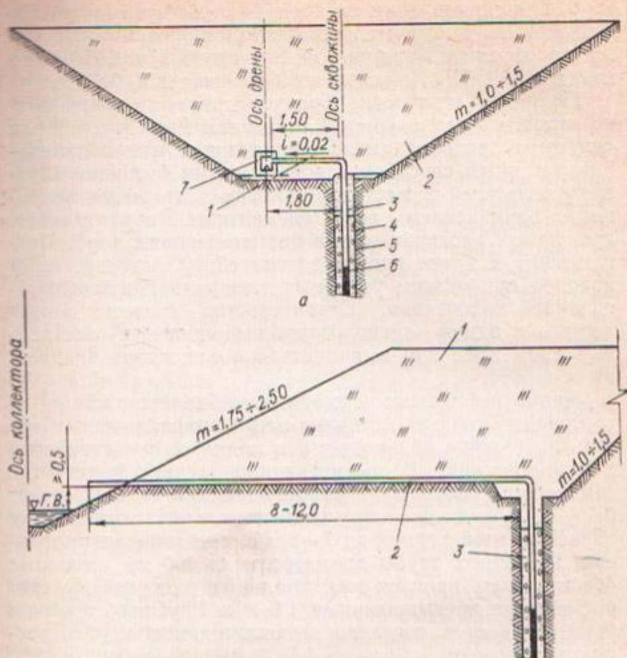
Рис. 10. Подключение скважины-усилителя:
