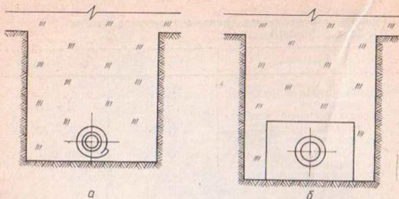
Рис. 6. Рекомендуемые конструкции дрена для бесстраншейного способа строительства закрытого дренажа (по Е. Д. Томину):
