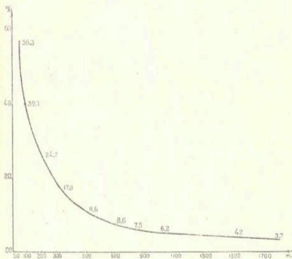
Рис. 1. Потери времени на повороты при вспашке на различную длину гона.
