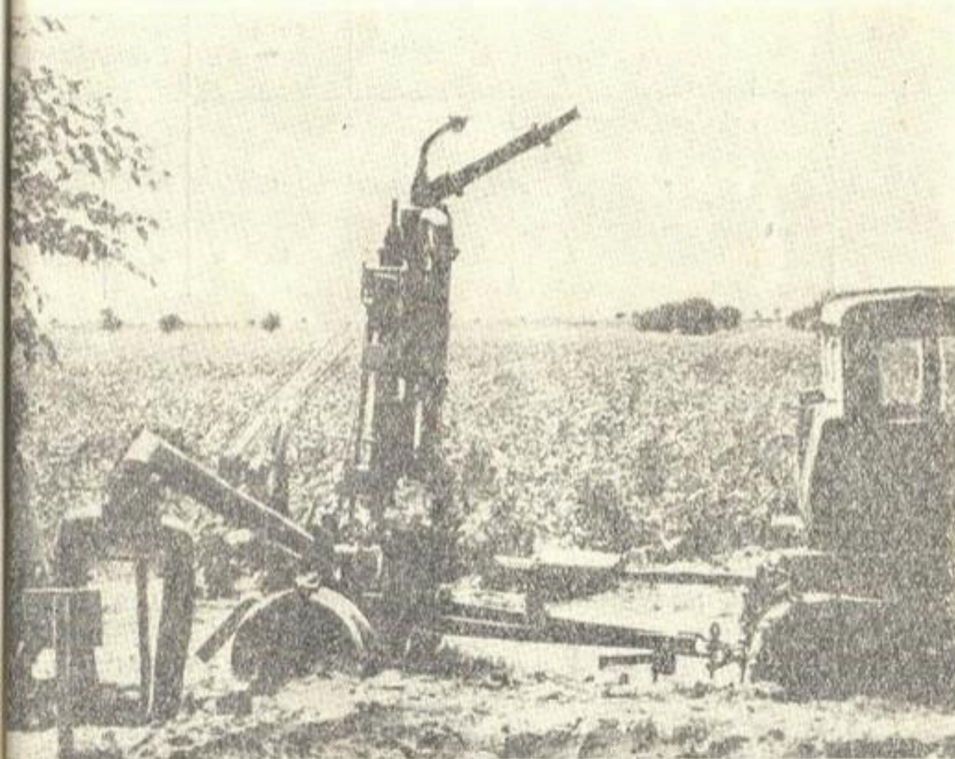
Рис. 5. Дальнеиструйная дождевальная прицепная машина ДДП-ЗОС.
