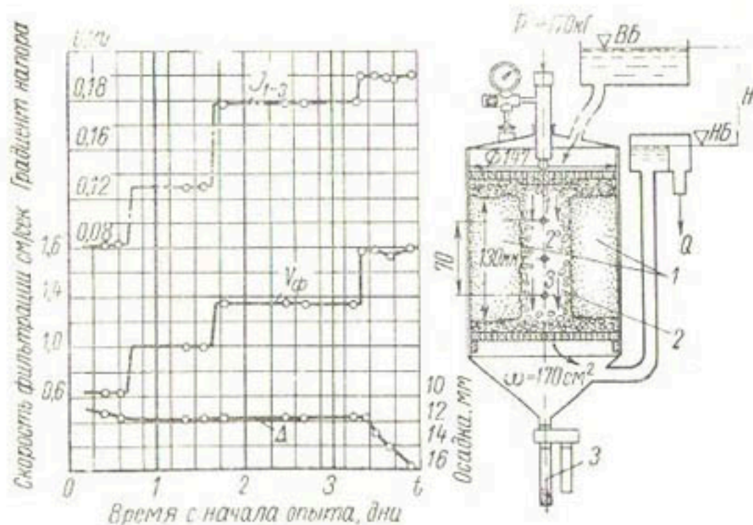
Рис. 22. Схема и результаты опыта по определению сопротивляемости суглинка размыву продольным вертикальным фильтрационным потоком в слое гравия 1—суглинок \gamma_{c,н} = 1,31 \text{ г/см}^3 ; W_n = 18,7\% ; 2—гравий; 3—песколовка.
