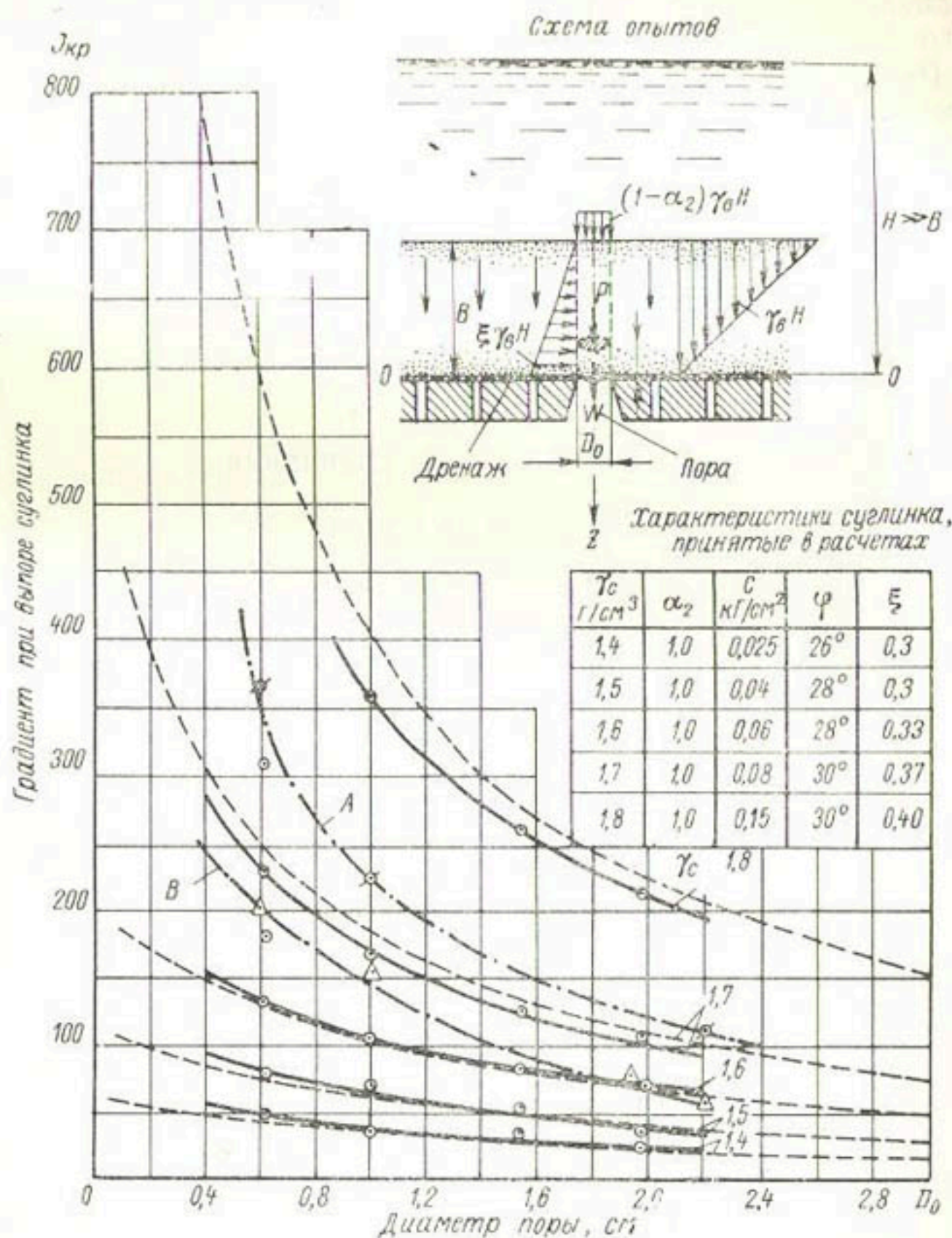
Рис. 18. Графики зависимостей между критическим градиентом фильтрационного потока и диаметром отверстия при контактом выпоре лессового суглинка с оптимальной начальной влажностью W_H = 16-18\% :
