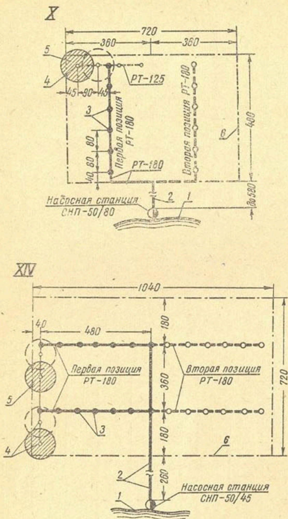
Рис. 9. Схемы орошения участков с помощью дождевальной машины ДДН-45:
