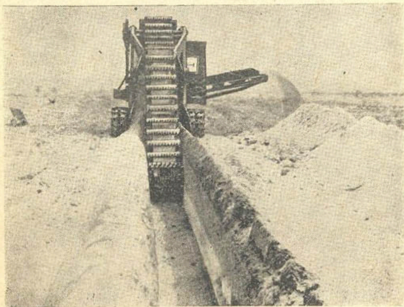
Рис. 73. Рытье траншеи для трубопровода закрытой оросительной сети многоковшовым экскаватором.
