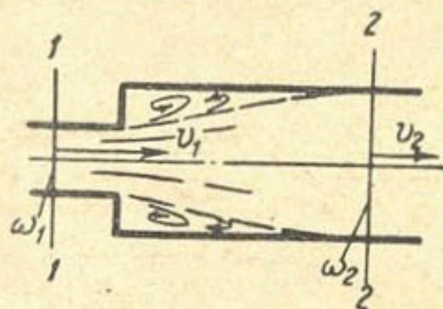
Рис. 35. Внезапное расширение.
