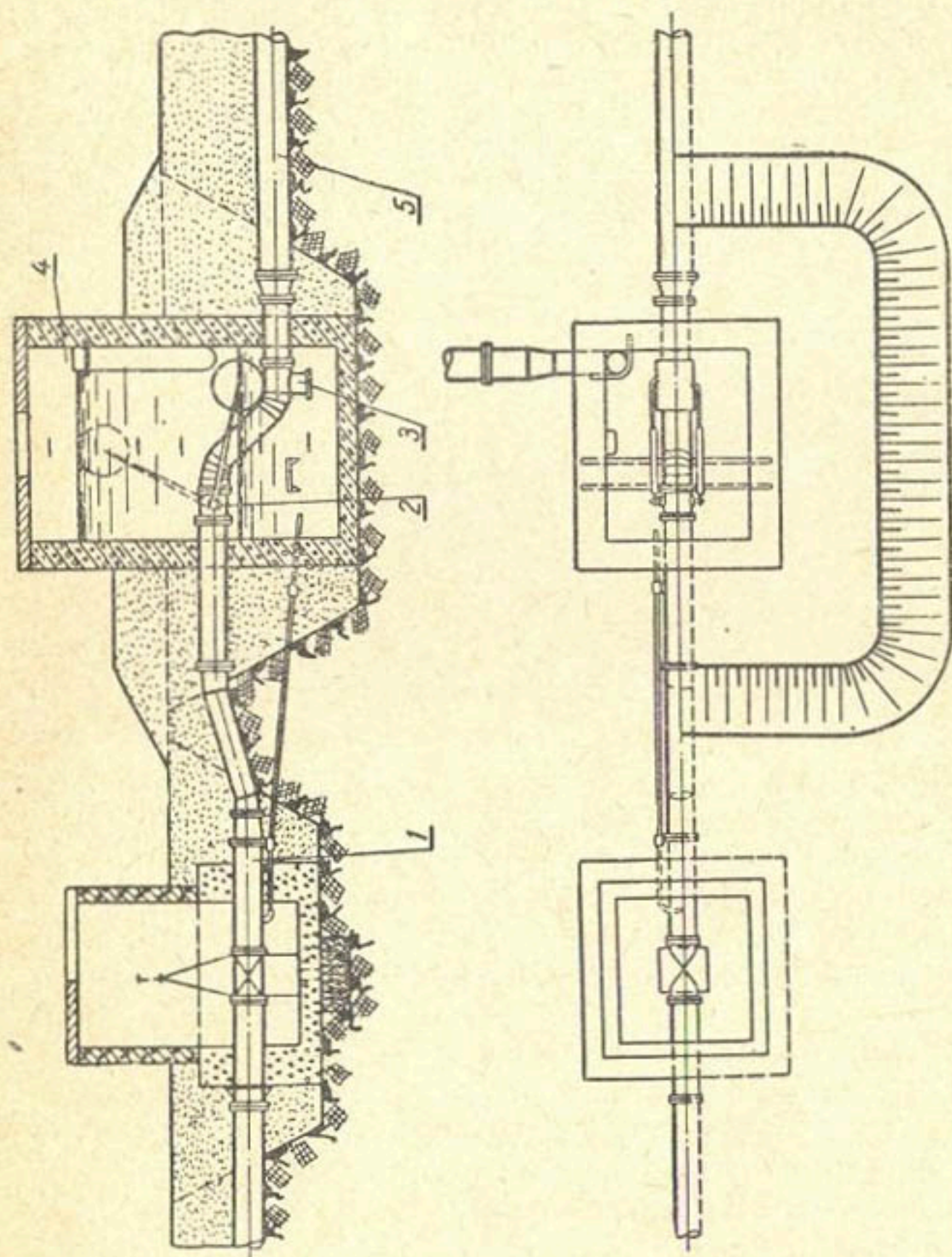
Рис. 67. Гаситель напора с патрубок-отводом: 1 — вышерасположенный трубопровод; 2 — дроссельный клапан; 3 — патрубок-отвод; 4 — ко- лодец; 5 — нижерасположенный трубопровод.
