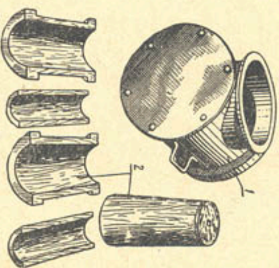
Рис. 55. Разборная опалубка: 1 — металлическая разъемная форма; 2 — деревянные сердечники.
