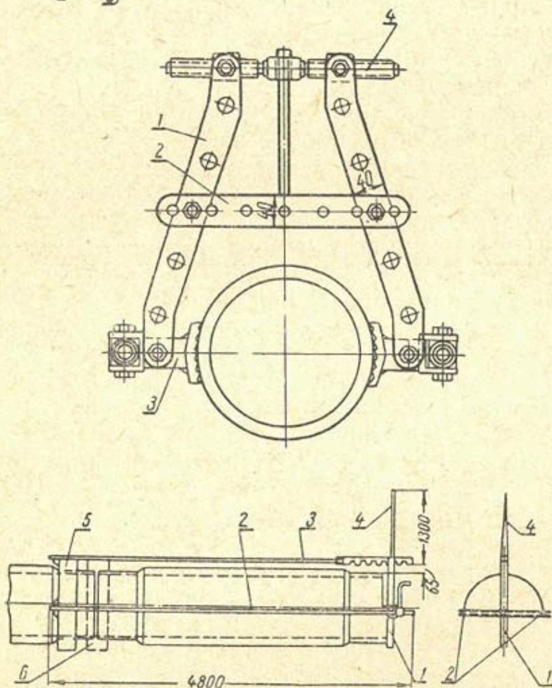
Рис. 77. Соединение труб больших диаметров винтовым домкратом:
