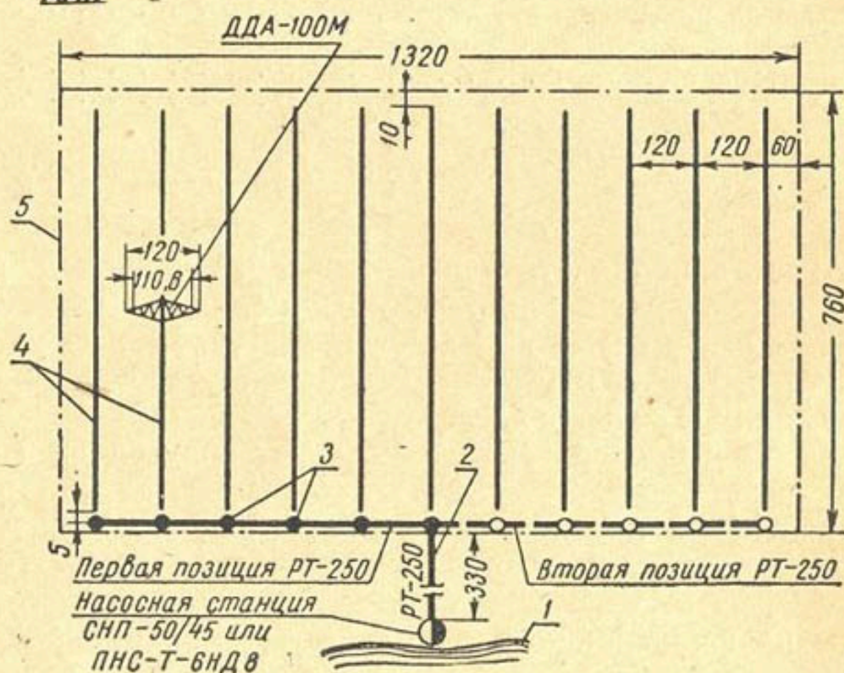
Рис. 10. Схемы орошения участков с помощью дождевального агрегата ДДА-100М: XXI—XXII — площадь орошения за сезон 100 га; 1 — водоем; 2 — подводящая часть трубопровода; 3 — труба-гидрант 250×180; 4 — открытые оросители; 5 — граница орошаемой площади.
