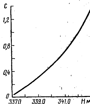
Рис. 3. Зависимость коэффициента C от уровня оз. Балхаш
