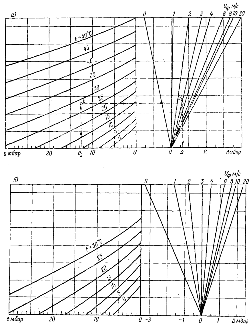
Рис. 3. Номограмма для определения поправки \Delta к влажности воздуха e_2 , вычисленной для стационарного психметра: а — P=1000 мбар, б — P=600 мбар
