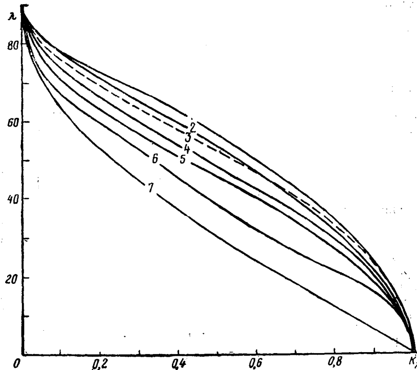
Рис. 3. Зависимость коэффициента уменьшения рассеянной солнечной радиации ( K_{\lambda} ) от угла закрытости горизонта \lambda и высоты солнца h_{\odot} : 1 — h_{\odot} = 16,5^{\circ} ; 2 — h_{\odot} = 15^{\circ} ; 3 — h_{\odot} = 20,5^{\circ} ; 4 — h_{\odot} = 30^{\circ} ; 5 — h_{\odot} = 50^{\circ} ; 6 — пасмурно; 7 — теоретическая кривая K_{\lambda} , вычисленная в предположении изотропного излучения всего небосвода
