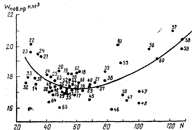
Рис. 1. Связь поверхностного притока (выше дельты) в оз. Балхаш с осредненными по семилеткам значениями чисел Вольфа ( N ) за 1911—1969 гг.
