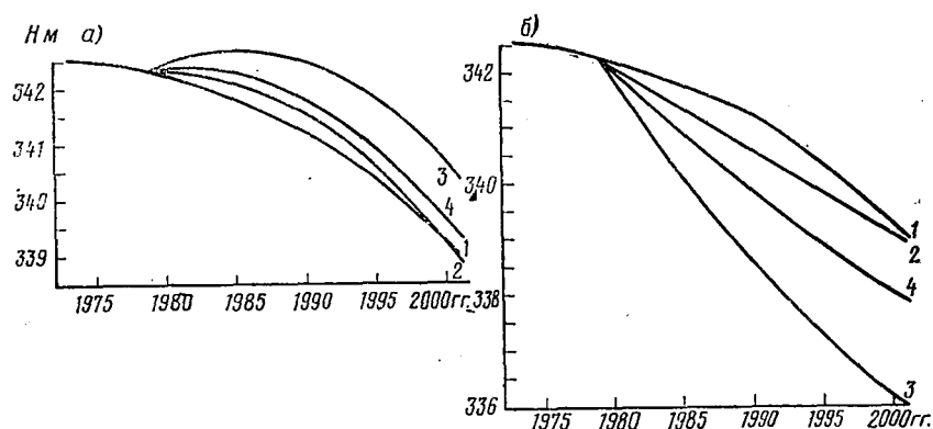
Рис. 4. Влияние на уровень Западного (а) и Восточного (б) Балхаша (прогноз с учетом климатического и хозяйственного факторов, вариант III с приостановкой наполнения Капчагайского водохранилища в 1974—1979 гг.) плотины в прол. Узун-Арал и переброски стока р. Каратал:
