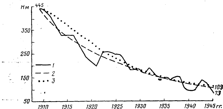
Рис. 3. Отклонения уровня оз. Балхаш, обусловленные коротко-периодными многолетними колебаниями водного баланса от фоновых значений уровня озера за фазу спада внутривекового цикла: 1 — фактические значения уровня, 2 — фоновые значения, 3 — кривая фоновых значений, рассчитанная воднобалансовым методом по фоновым значениям элементов водного баланса, аппроксимированных прямыми линиями; цифры у кривых — уровни к концу расчетного периода
