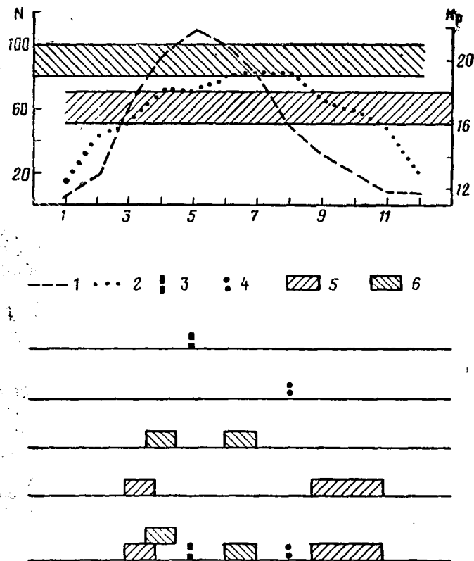
Рис. 1. Средние циклические кривые чисел Вольфа ( N ) и планетарного индекса геомагнитной возмущенности K_p (2) за 1888—1964 гг. и диаграмма максимумов различных видов солнечных воздействий:
