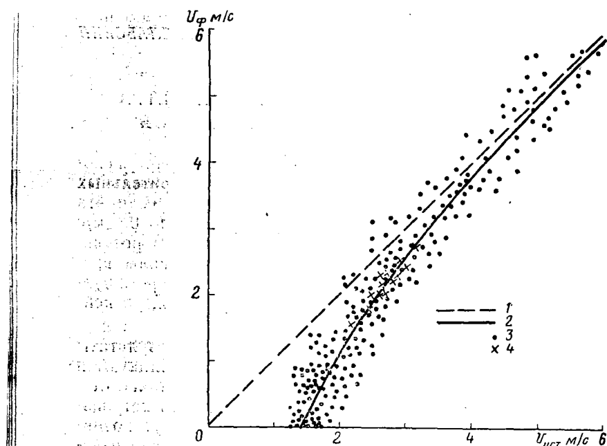
Рис. 1. Сопоставление измеренной флюгером (2) и истинной (1) скоростей ветра по материалам наблюдений 1969—1971 гг. на ст. Селезневка: 3, 4 — соответственно среднесуточная и среднемесячная скорости ветра
