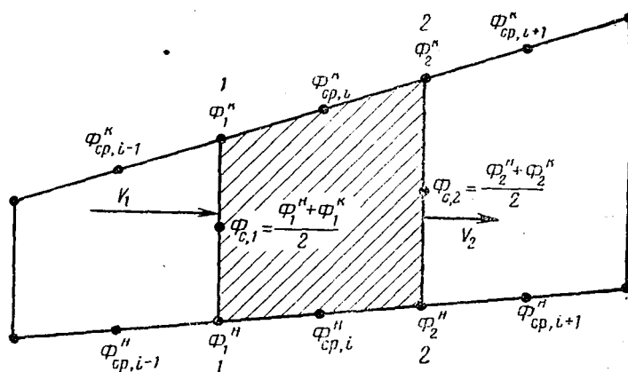
Рис. 1. Схема распределения величин минерализации воды во времени и по длине участка водоема
