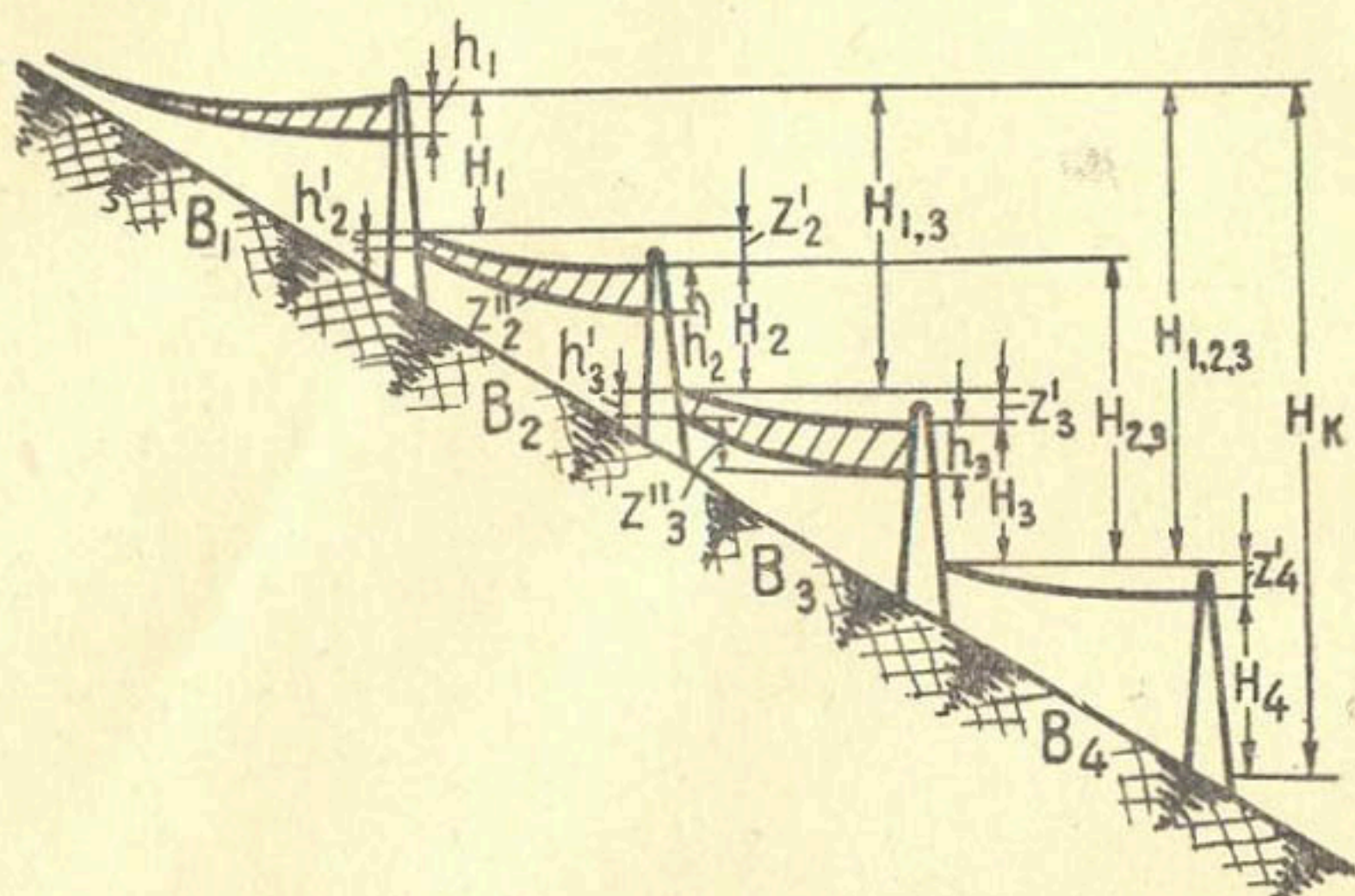
Рис. 17. Схема каскада ГЭС к выбору очередности сработки водохранилищ.
