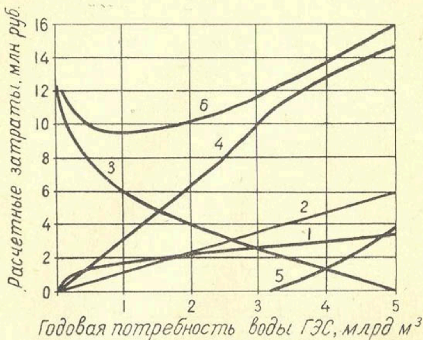
Рис. 44. Среднегодовые расчетные затраты в ГЭС 1, сэкономленное топливо 2, заменяющую КЭС 3, бассейн перерегулирования 4, компенсацию дефицита электроэнергии в системе 5 и их сумма 6 в зависимости от величины годовой потребности воды ГЭС для покрытия задачного графика нагрузки (схема IV).
