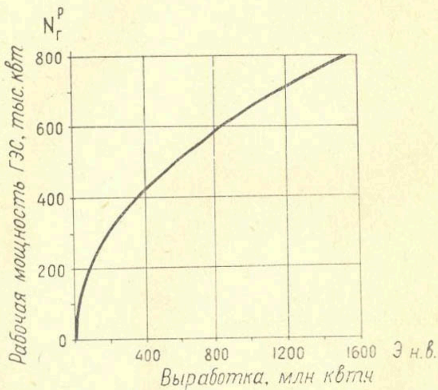
Рис. 55. Зависимость минимально необходимой выработки энергии проектируемой ГЭС в течение невегетационного периода \mathcal{E}_{\text{н.в.}} от ее рабочей мощности N_r^p
