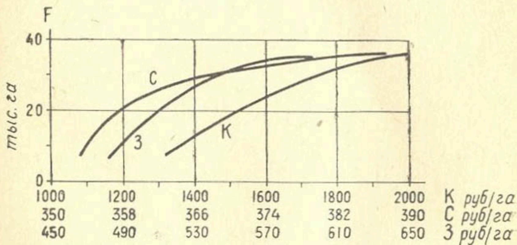
Рис. 12. Величины удельных капитальных вложений K , ежегодных эксплуатационных издержек C и среднегодовых расчетных затрат Z на дополнительный гектар в зависимости от площади орошения F при увеличении емкости регулирующего водохранилища.
