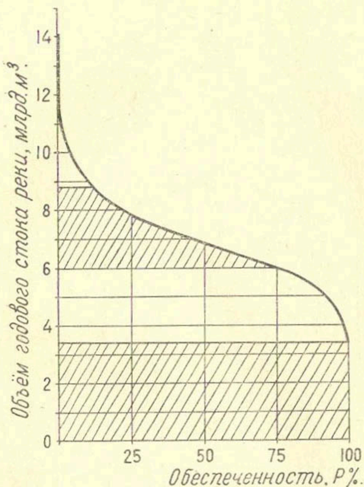
Рис. 34. Кривая обеспеченности годовых объемов стока реки в створе проектируемого комплексного гидроузла. C_v = 0,22 ; \bar{V}_{\text{год}} = 7,0 млрд \text{м}^3 .
