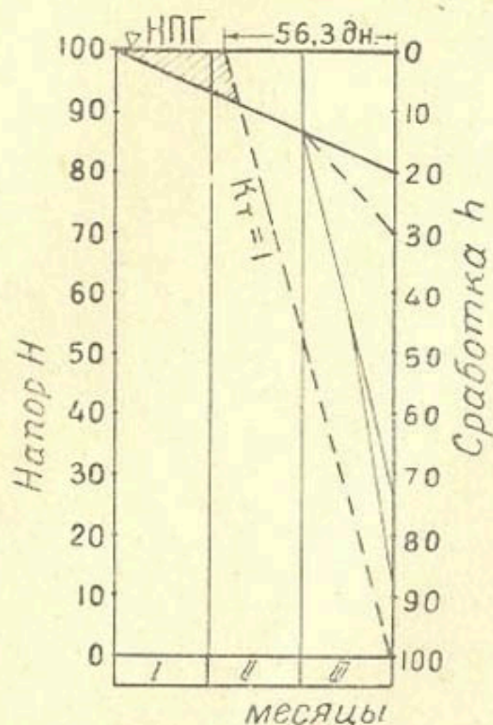
Рис. 22. Режим сработки водохранилища
