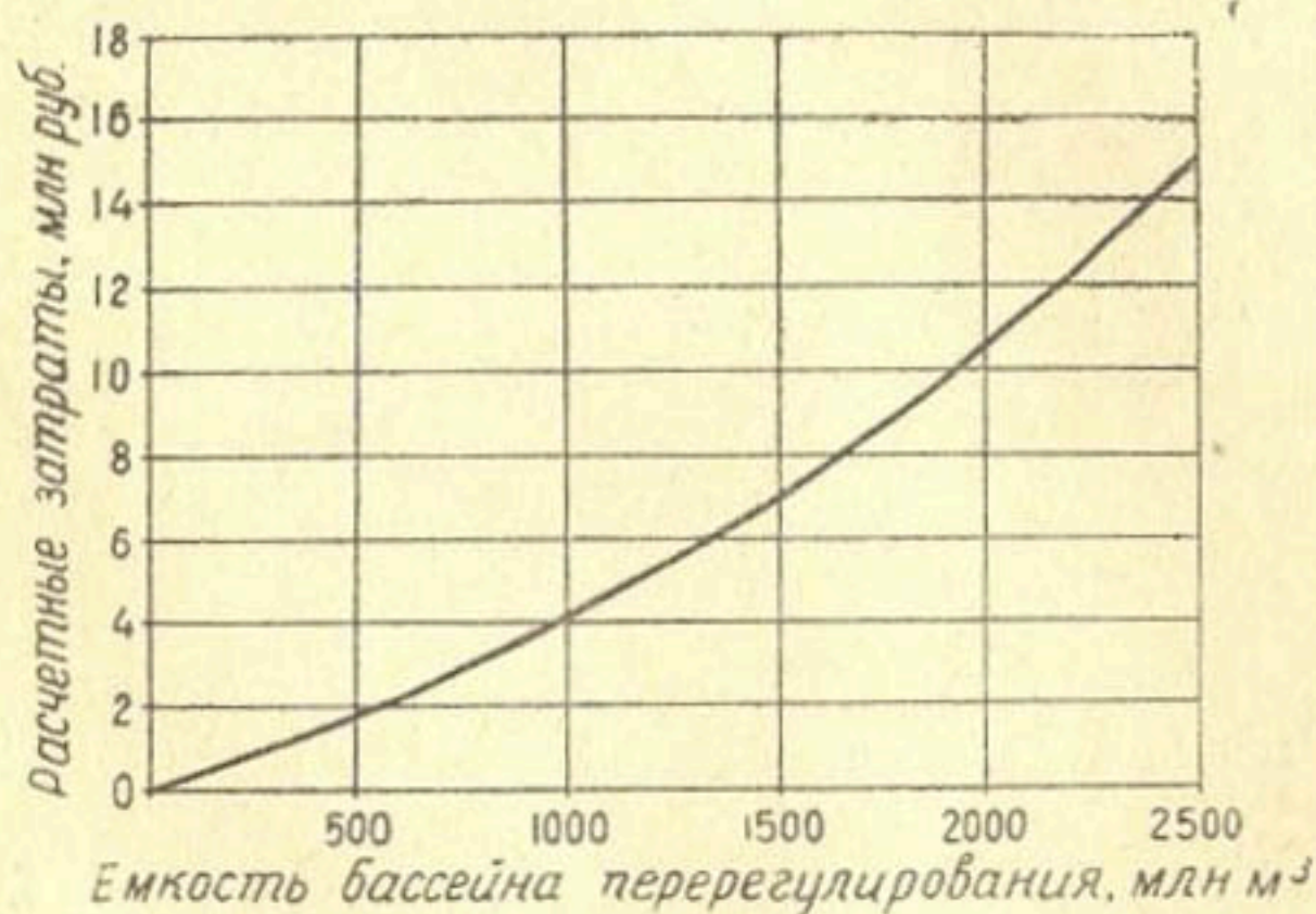
Рис. 43. Зависимость среднегодовых расчетных затрат по бассейну перерегулирования от его полезной емкости.
