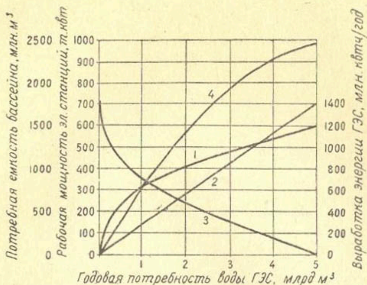
Рис. 42. Зависимости рабочей мощности 1 и выработки энергии 2 проектируемой ГЭС, мощности заменяющей КЭС 3 и необходимой емкости бассейна перерегулирования 4 от величины годовой потребности воды ГЭС (схема IV).
