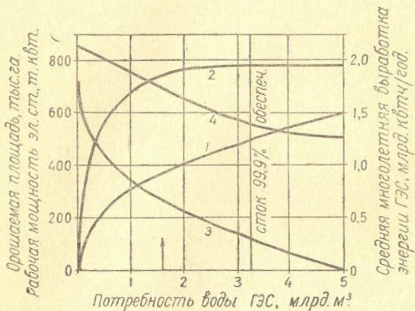
Рис. 35. Зависимости рабочей мощности проектируемой ГЭС 1, ее средней многолетней выработки энергии 2, мощности заменяющей КЭС 3 и площади орошения 4 от годовой потребности воды ГЭС для покрытия гарантируемой зоны графика нагрузки энергосистемы (схема II-а).
