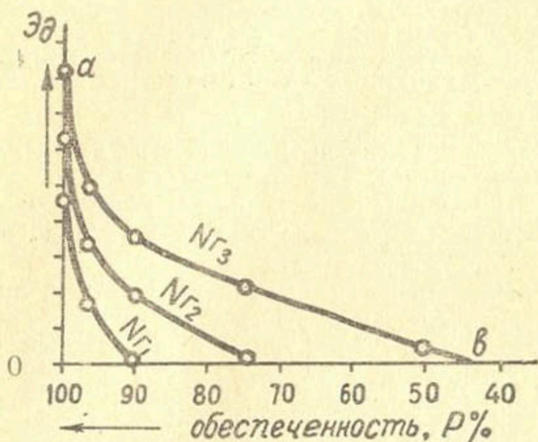
Рис. 32. Зависимости величины годового дефицита энергии в системе \mathcal{E}_d от обеспеченности годового стока p при трех значениях мощности проектируемой ГЭС.
