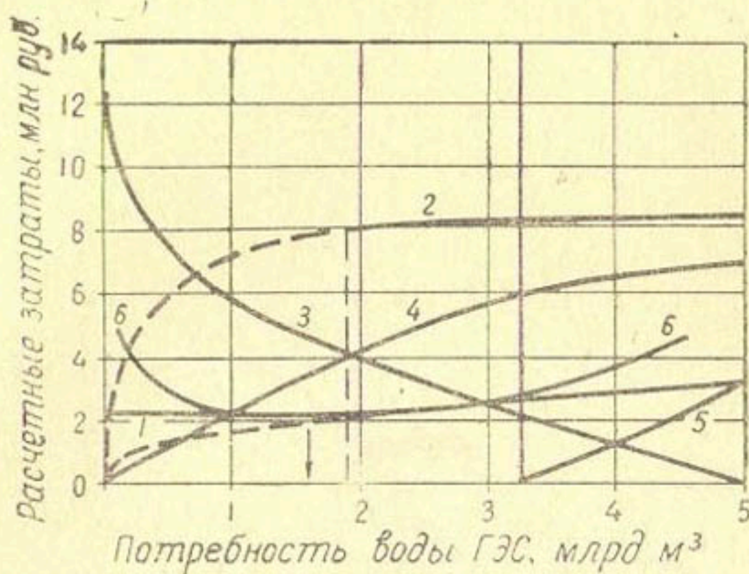
Рис. 36. Среднегодовые расчетные затраты в GES 1, сэкономленное топливо 2, в заменяющую КЭС 3, дополнительные затраты в сельское хозяйство 4, компенсацию дефицита электроэнергии в системе 5 и сумма 6 в зависимости от годовой потребности воды GES для покрытия гарантируемой зоны графика нагрузки энергосистемы (схема II-а).
