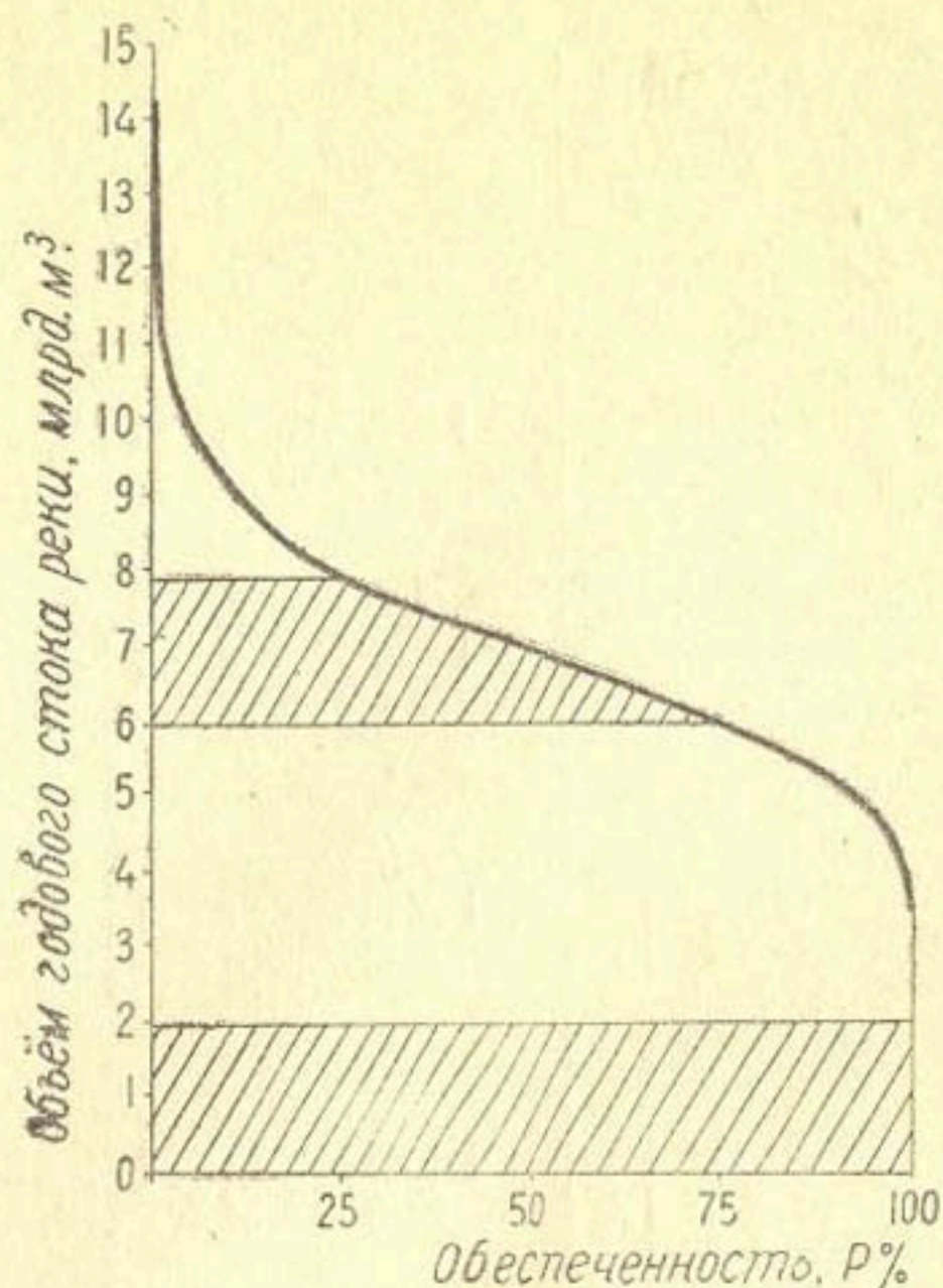
Рис. 52. Кривая обеспеченности годовых объемов стока реки в створе проектируемой ГЭС.
