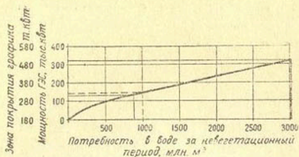
Рис. 49. Потребности в воде ГЭС-3 за невегетационный период в зависимости от ее мощности.
