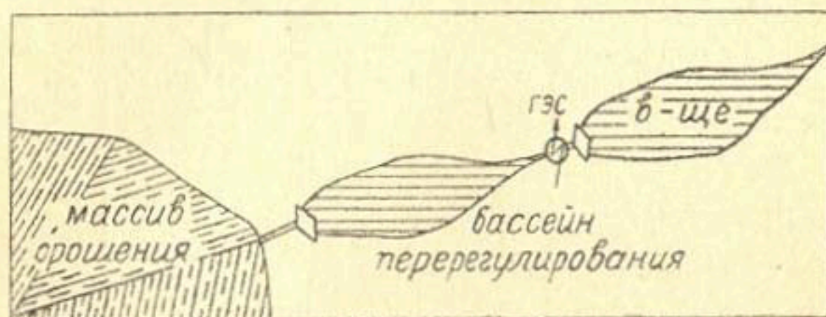
Рис. 41. Четвертая расчетная схема использования ресурсов реки.
