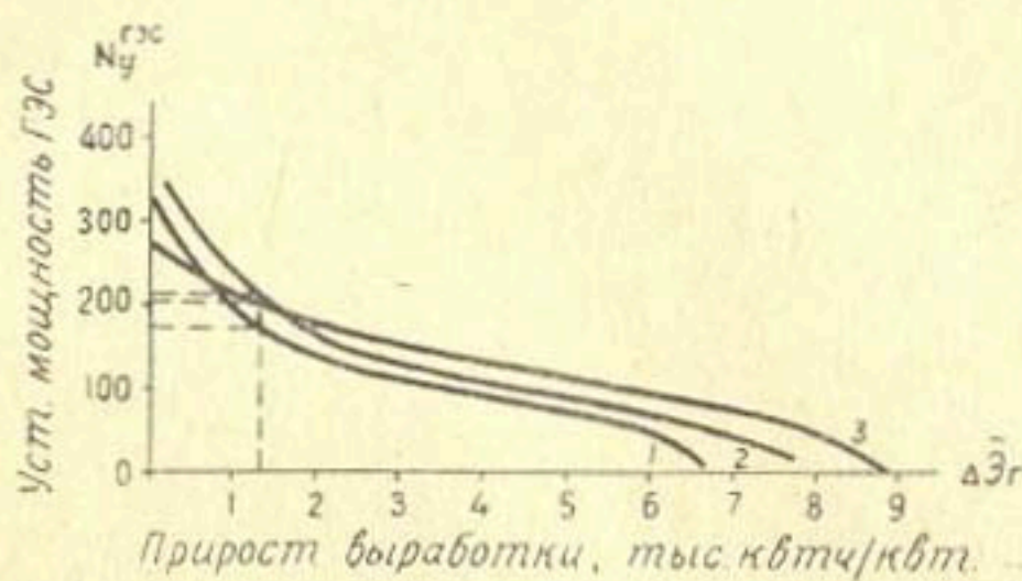
Рис. 53. Зависимости прироста средней многолетней выработки энергии дополнительного киловатта от установленной мощности ГЭС—1, 2, 3.
