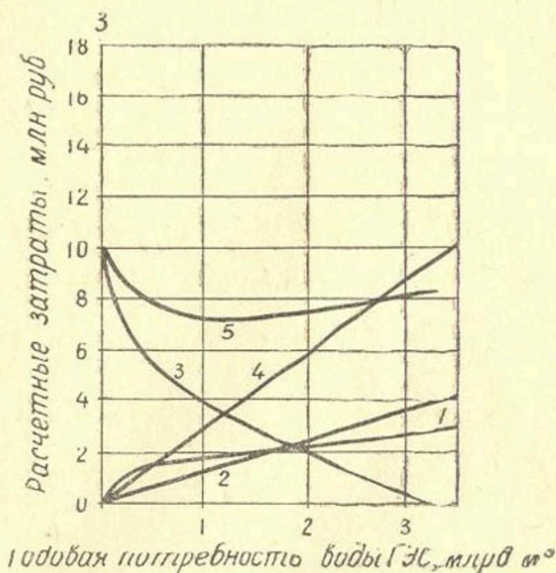
Рис. 27. Зависимости среднегодовых расчетных затрат в ГЭС 1, сэкономленное топливо 2, заменяющую КЭС 3, дополнительных затрат в сельское хозяйство 4 и их суммы 5 от годовой потребности воды ГЭС (для схемы I)
