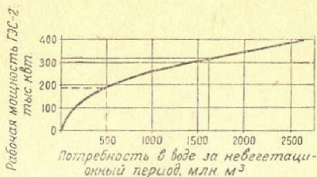
Рис. 48. Потребности в воде ГЭС-2 за невегетационный период в зависимости от ее рабочей мощности
