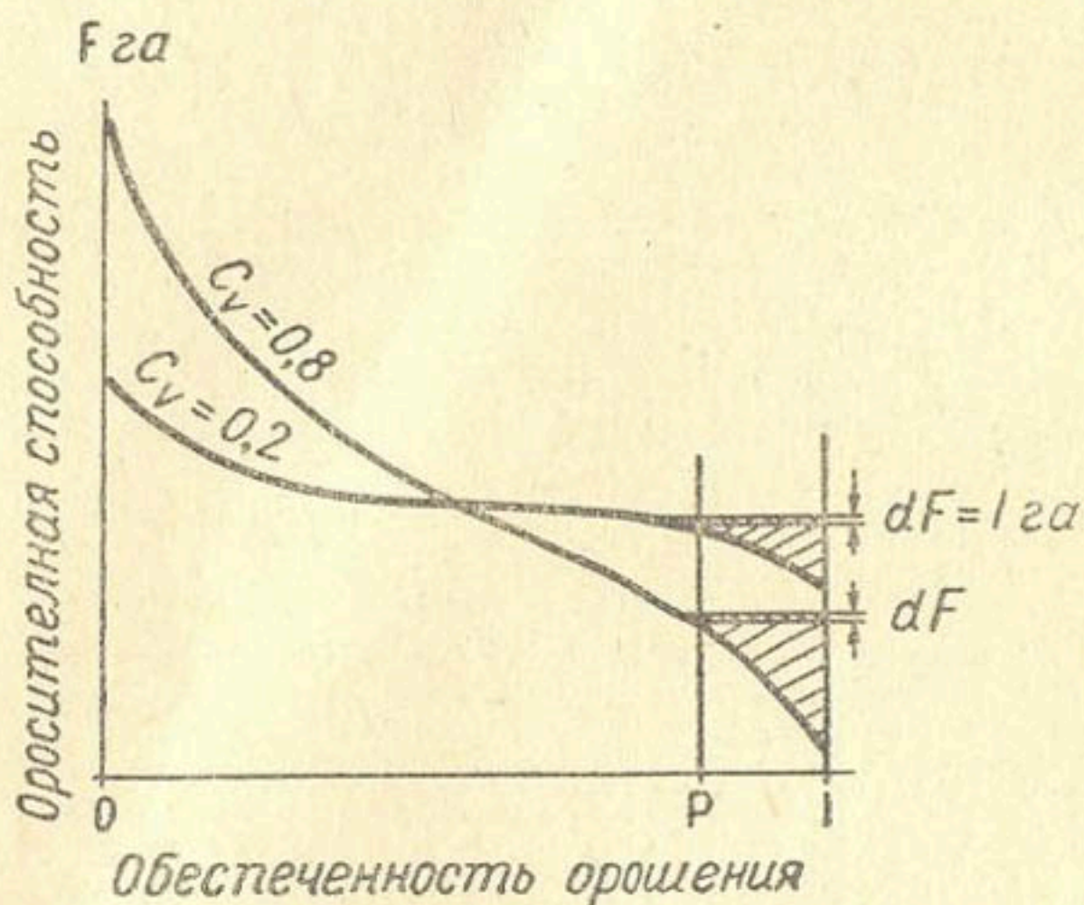
Рис. 9. Кривые зависимости оросительной способности систем от их обеспеченности. Штриховкой показана суммарная величина недополивов в критические маловодные годы; двойной штриховкой — ее прирост на дополнительный гектар.
