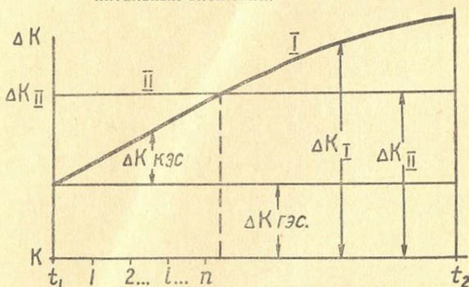
Рис. 5. Динамика изменений капитальных вложений по вариантам: I — на ГЭС к первому расчетному уровню t_1 устанавливается полная мощность N'_r с последующей компенсацией ее снижения, наращиванием тепловой мощности; II — на уровне t_1 устанавливается мощность ГЭС, равная N_r , и дополнительная мощность ГЭС — \alpha_N \Delta N_r
