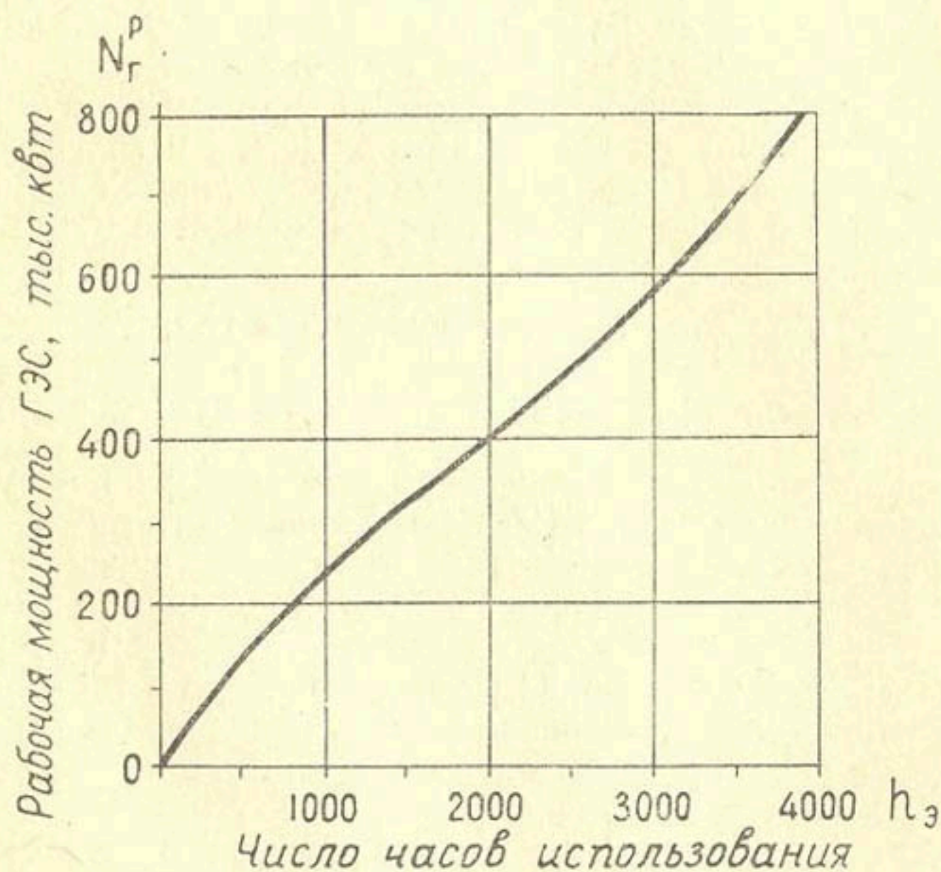
Рис. 56. Зависимость числа часов использования дополнительного киловатта проектируемой ГЭС в графике нагрузки энергосистемы за невегетационный период года h_g от величины ее рабочей мощности N_r^p
