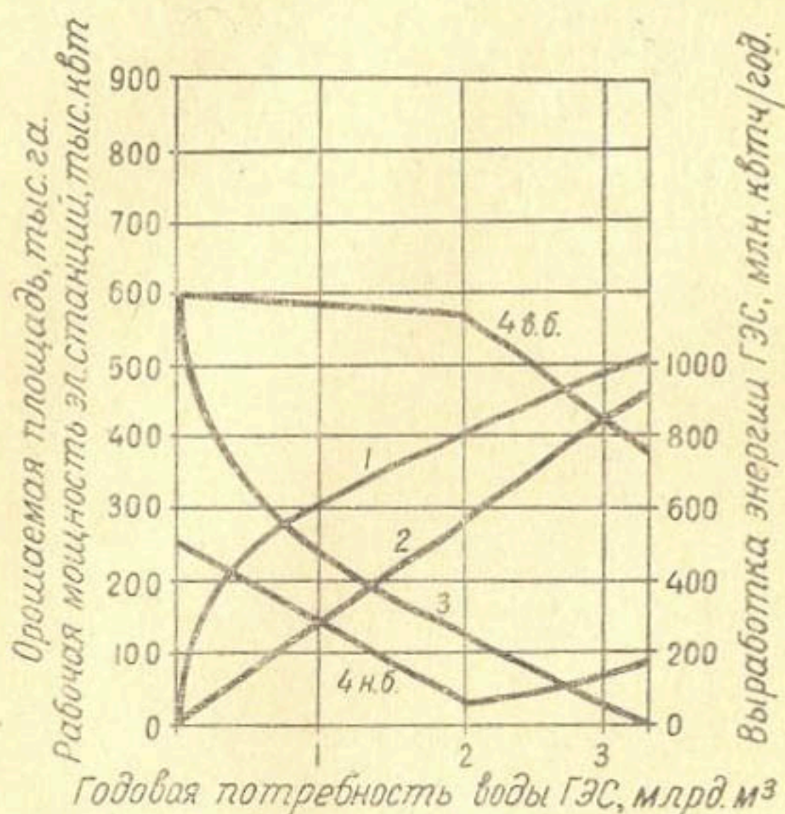
Рис. 39. Зависимости рабочей мощности 1 и выработки энергии 2 проектируемой ГЭС, мощности заменяющей КЭС 3, площади орошения в верхнем (4 в. б.) и нижнем (4 н. б.) бьефах от годовой потребности воды ГЭС (схема III)
