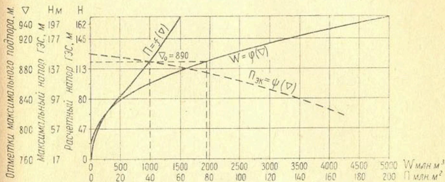
Рис. 54. Емкость W и площадь зеркала P проектируемого водохранилища сезонного регулирования стока в зависимости от отметки подпора
