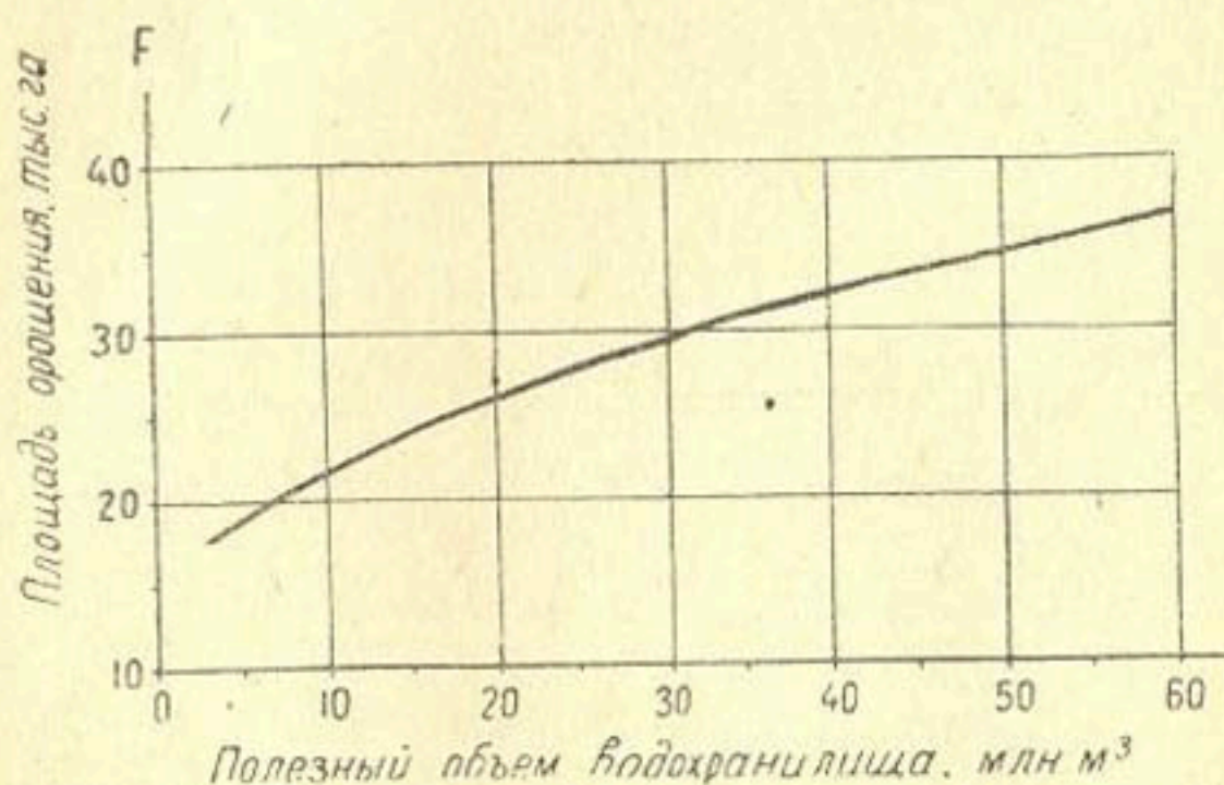
Рис. 10. Зависимость оросительной способности реки в году расчетной обеспеченности от величины полезной емкости регулирующего водохранилища.
