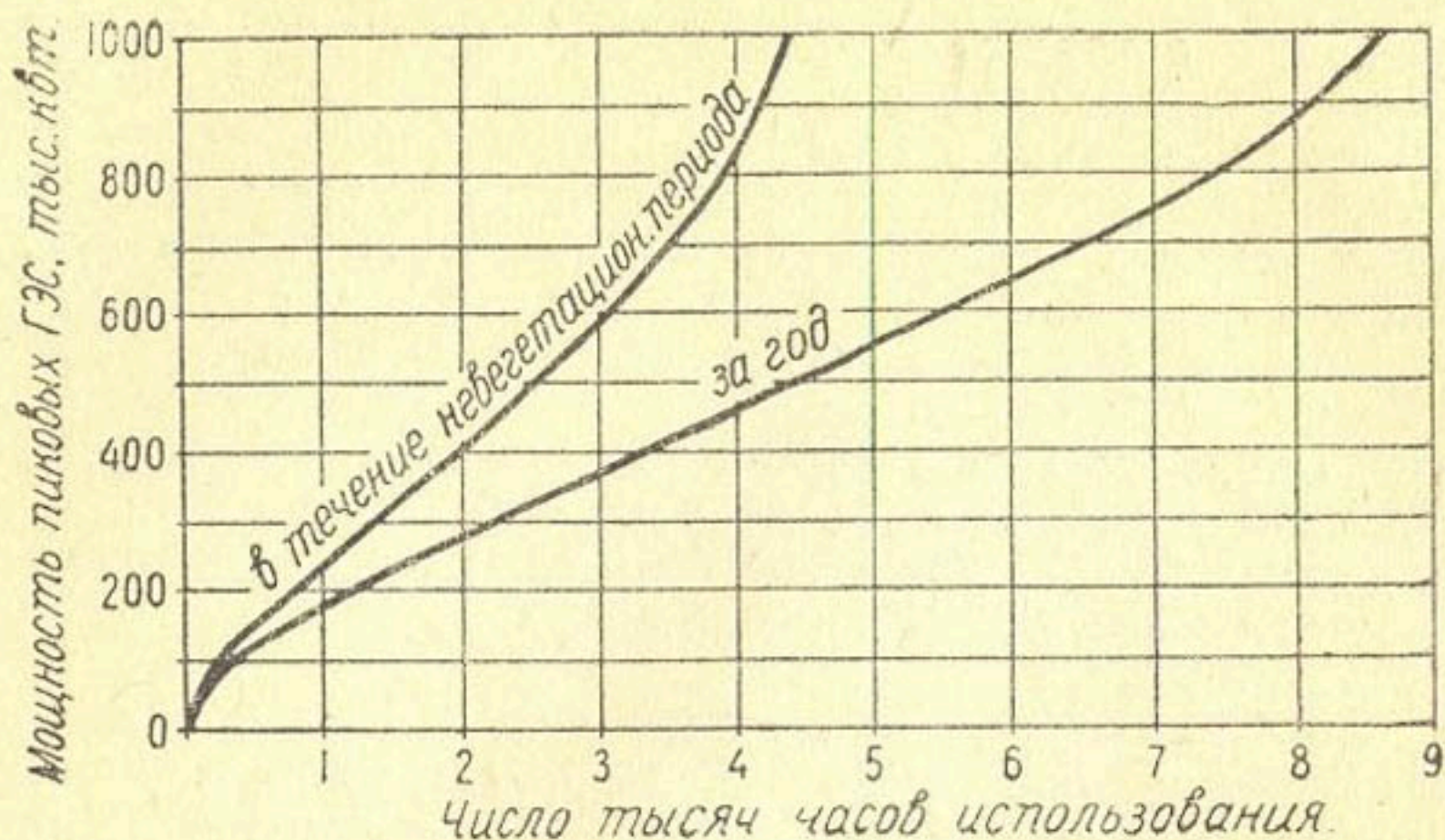
Рис. 45. Зависимости числа часов использования в графике нагрузки энергосистемы дополнительного киловатта на пиковых ГЭС от величины их рабочей мощности.
