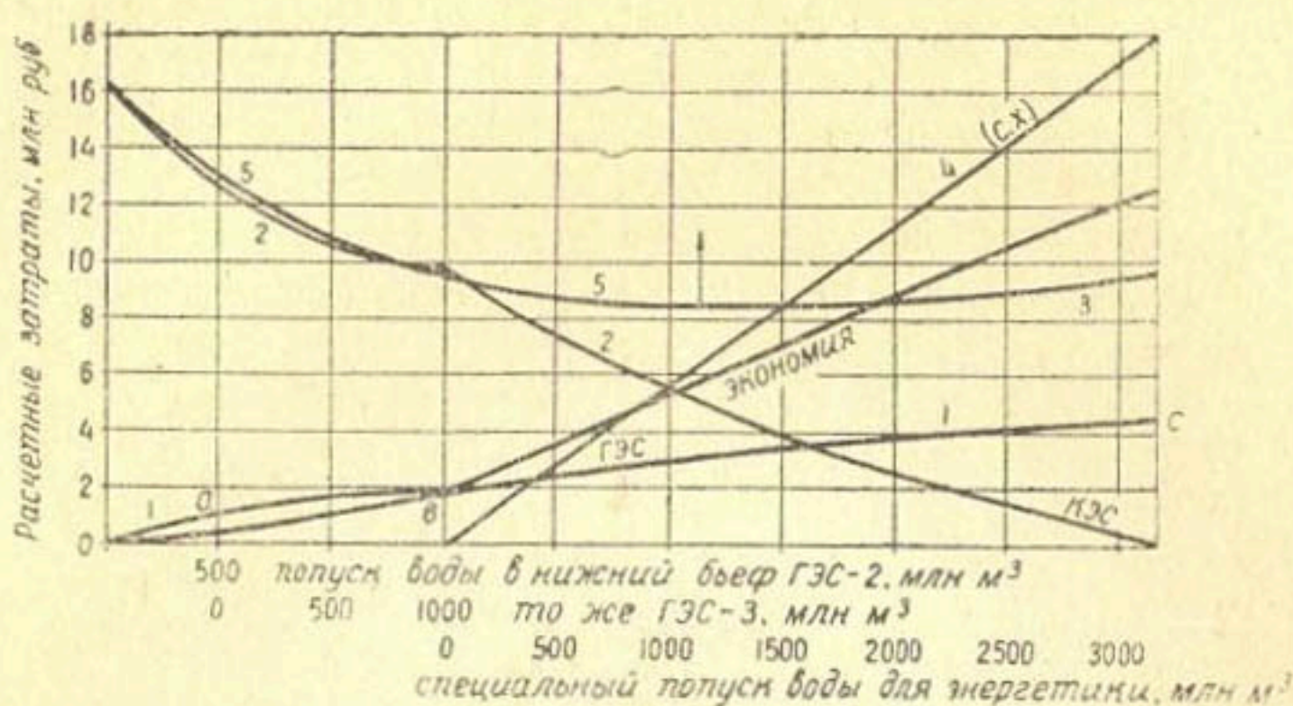
Рис. 51. Среднегодовые расчетные затраты в ГЭС 1, сэкономленное топливо 2, заменяющую КЭС 3 дополнительные затраты в сельское хозяйство 4 и их сумма 5 в зависимости от величины используемого гидроэлектростанциями количества воды за вегетационный период года.
