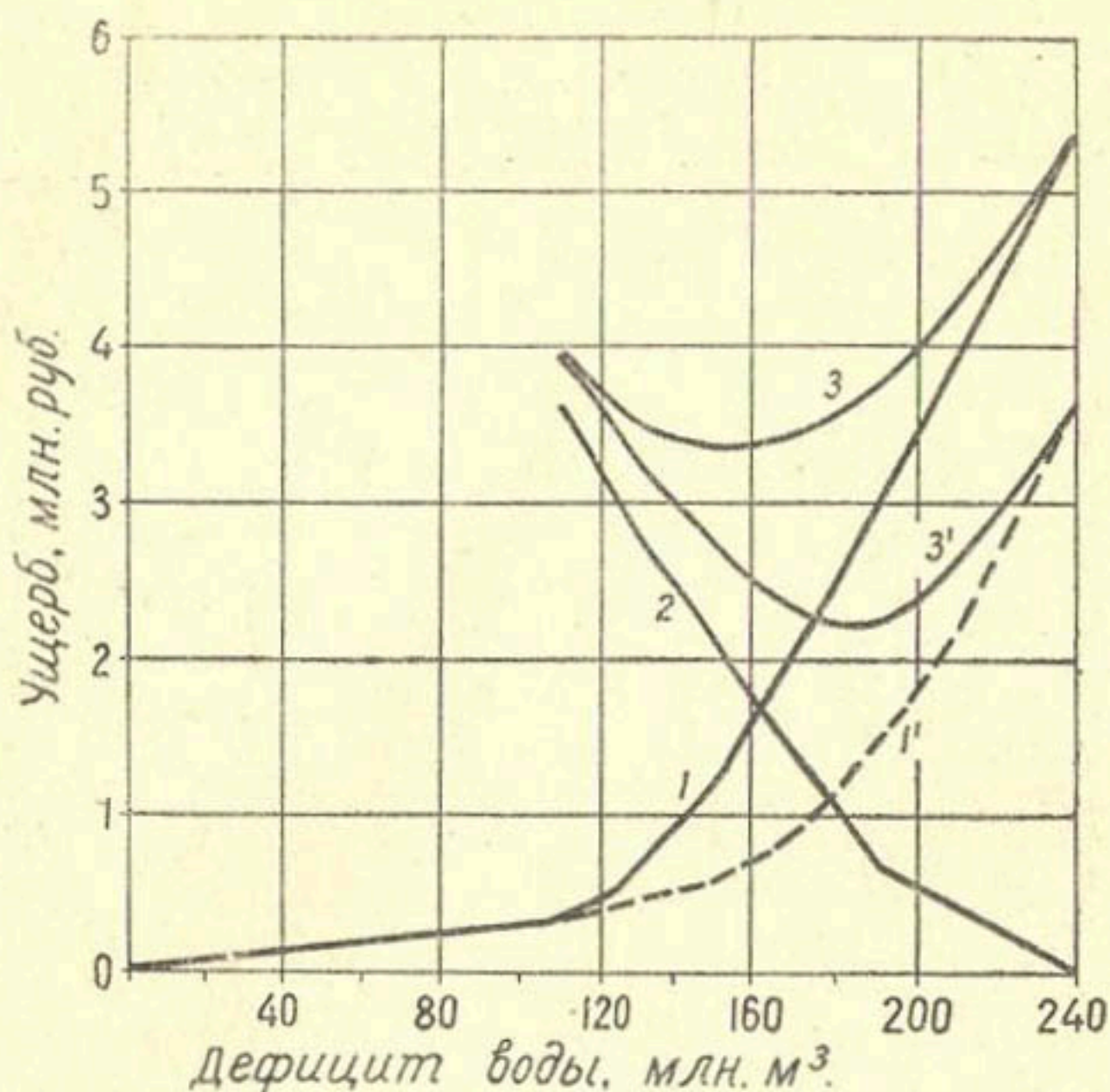
Рис. 61. Зависимости ущербов от ограничений в воде: 1—производственно-энергетической системы (без ограничения коммунально-бытовой нагрузки системы); 1'—то же с учетом ограничения коммунально-бытовой нагрузки; 2—сельскохозяйственных потребителей; 3—суммарные государственные ущербы от ограничений в воде без учета ограничений коммунально-бытовой нагрузки энергосистемы; 3' — то же с учетом этих ограничений.
