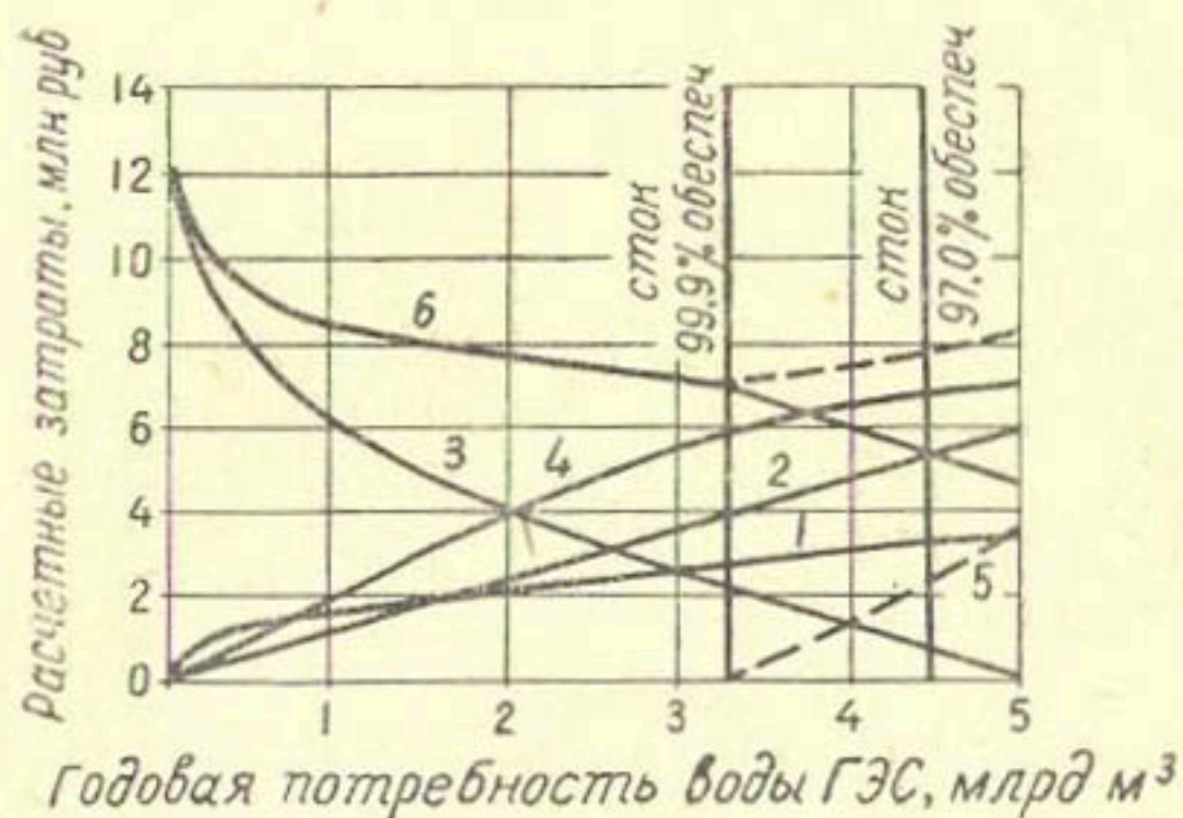
Рис. 31. Зависимости среднегодовых расчетных затрат в ГЭС 1, сэкономленное топливо 2, заменяющую КЭС 3, дополнительных затрат в сельское хозяйство 4, компенсацию дефицита электроэнергии в системе 5 и их суммы 6 от годовой потребности воды ГЭС (для схемы II)
