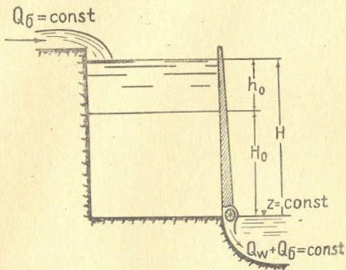
Рис. 21. Схема ГЭС к анализу методов выбора глубины сработки водохранилища.
