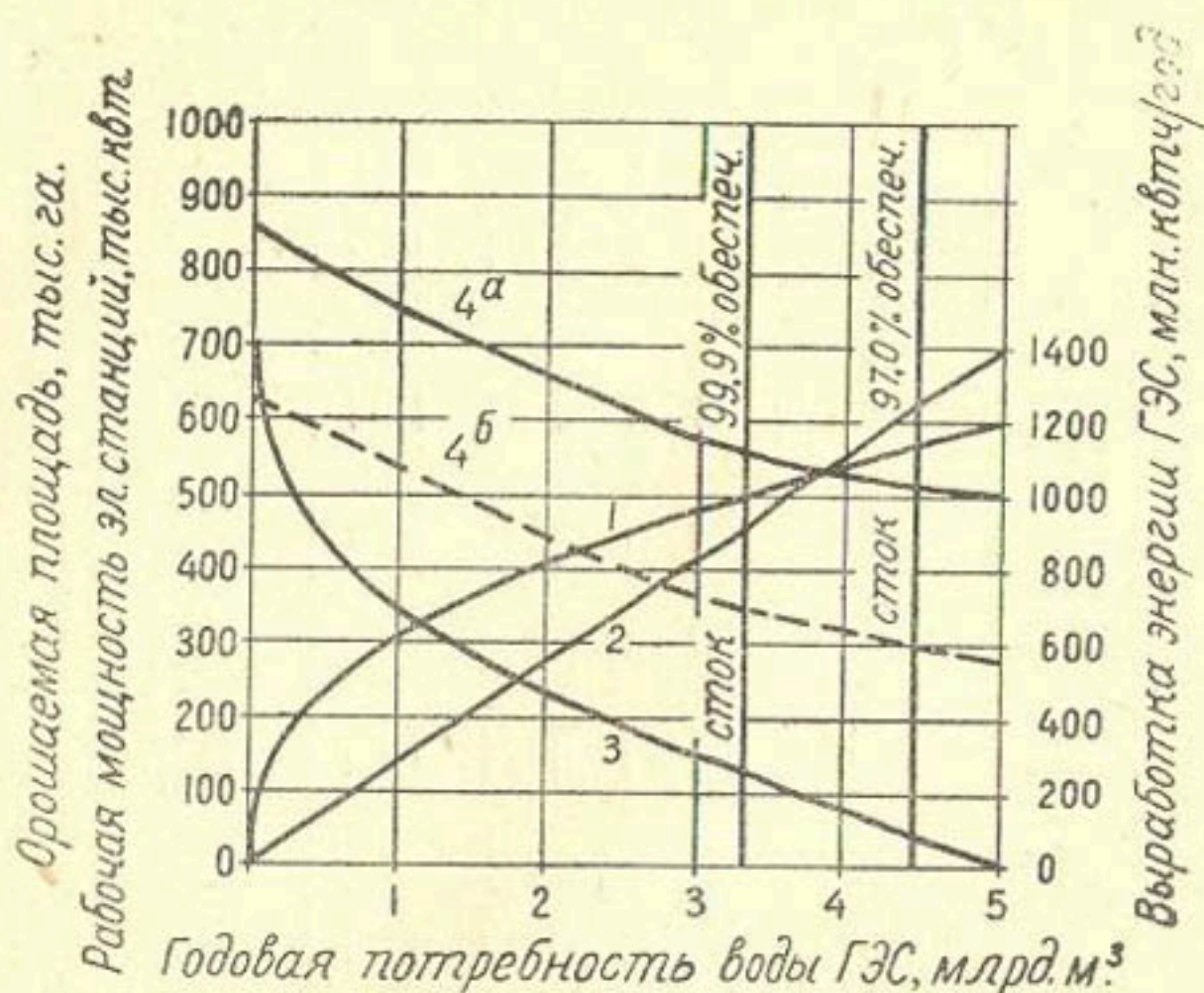
Рис. 30. Зависимости рабочей мощности 1 и выработки энергии 2 проектируемой ГЭС, мощности заменяющей КЭС 3 и площади орошения 4 от годовой потребности ГЭС для покрытия заданного графика нагрузки (для схемы II)
