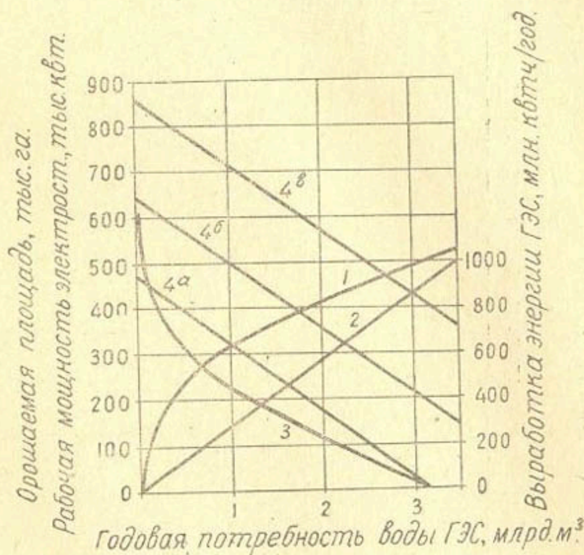
Рис. 26. Зависимости рабочей мощности 1 и выработки энергии 2 проектируемой ГЭС, мощности заменяющей КЭС 3 и площади орошения 4 от годовой потребности воды ГЭС для покрытия заданного графика нагрузки (для схемы I)
