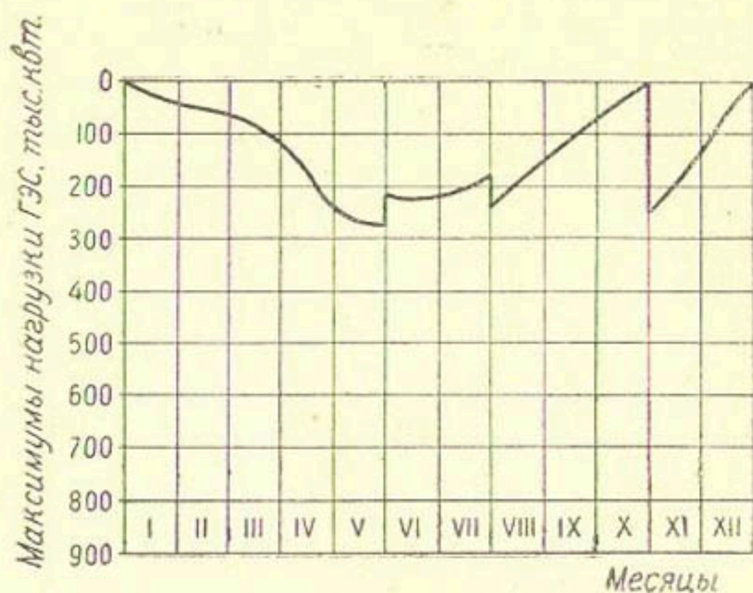
Рис. 15. Расчетный график нагрузки проектируемых ГЭС.
