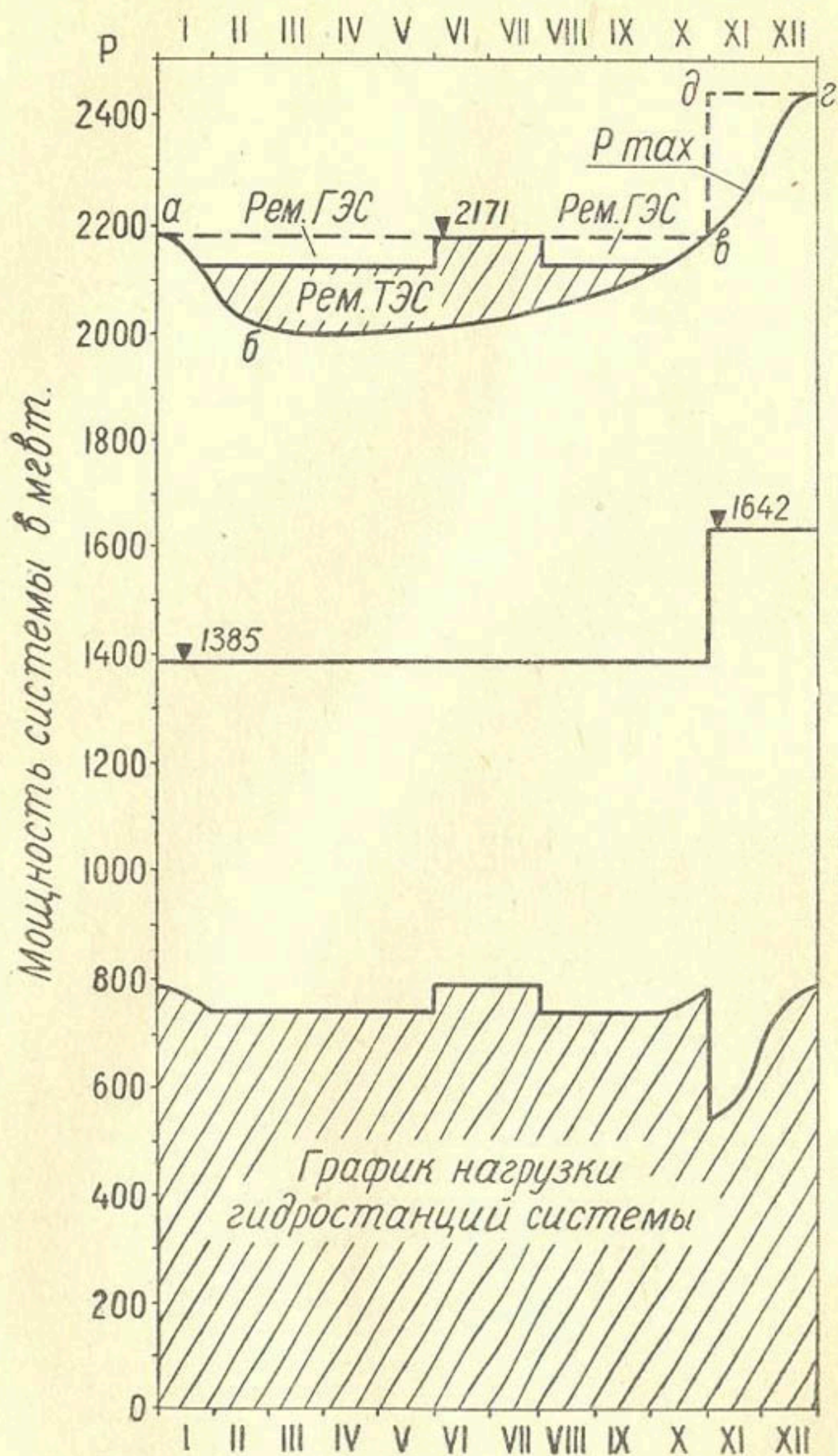
Рис. 14. Расчетный график нагрузки энергосистемы. При его построении принято, что вся тепловая мощность системы 4,5% времени в году находится в ремонте.
