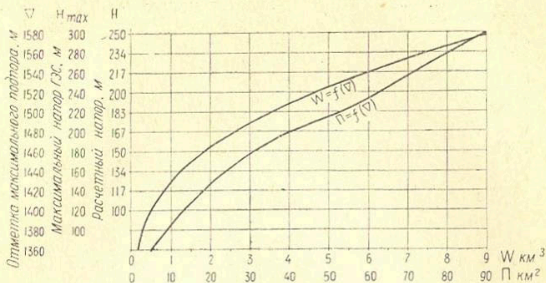
Рис. 58. Емкость W и площадь зеркала \Pi проектируемого водохранилища многолетнего регулирования стока в зависимости от отметки подпора
