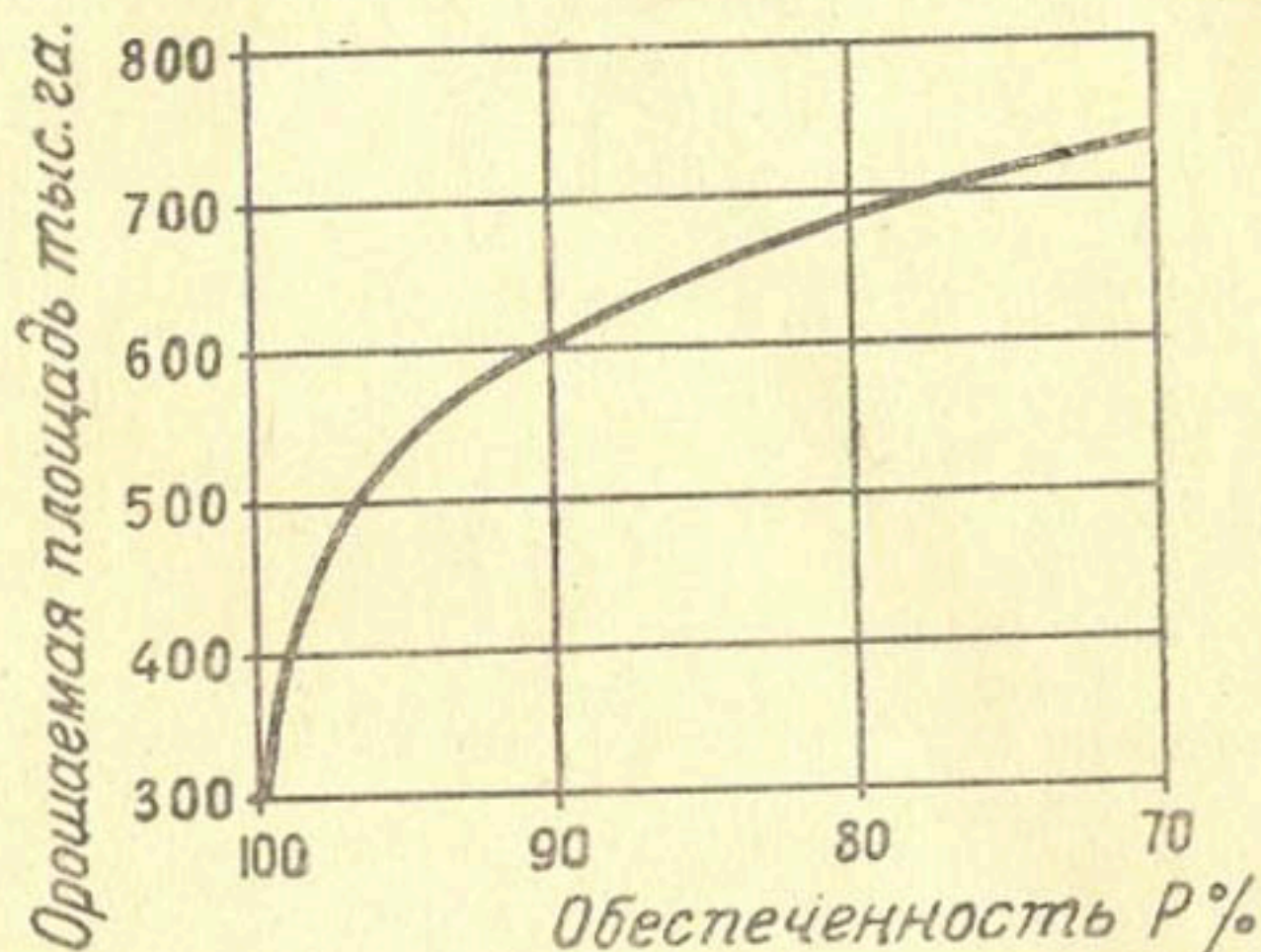
Рис. 28. Зависимость величины орошаемой площади от обеспеченности годового стока реки при мощности проектируемой ГЭС 320 тыс. квт
