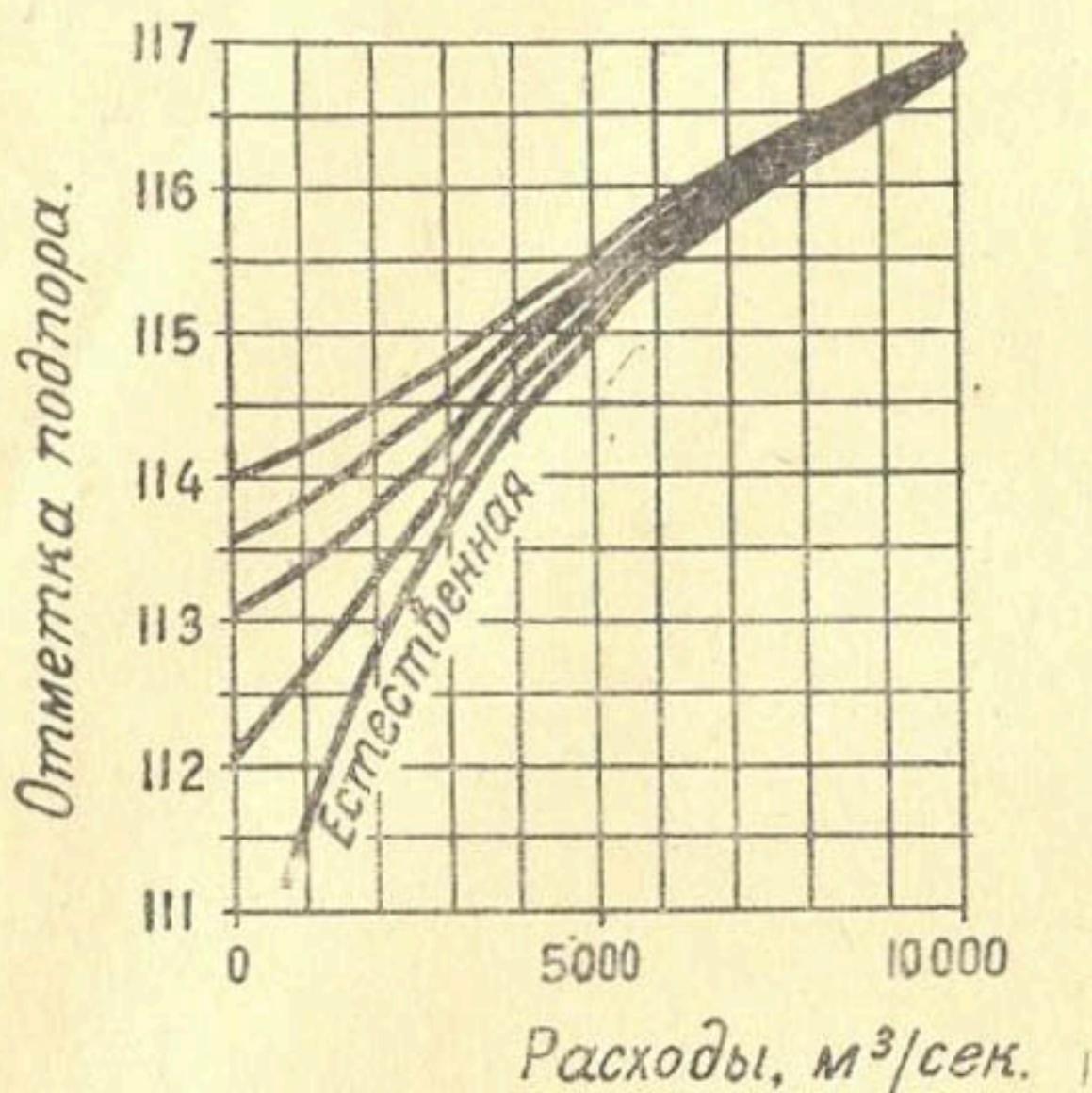
Рис. 19. Кривые расходов в створе ГЭС-I в естественных условиях и при подпоре ее водохранилищем ГЭС-II (летний режим).
