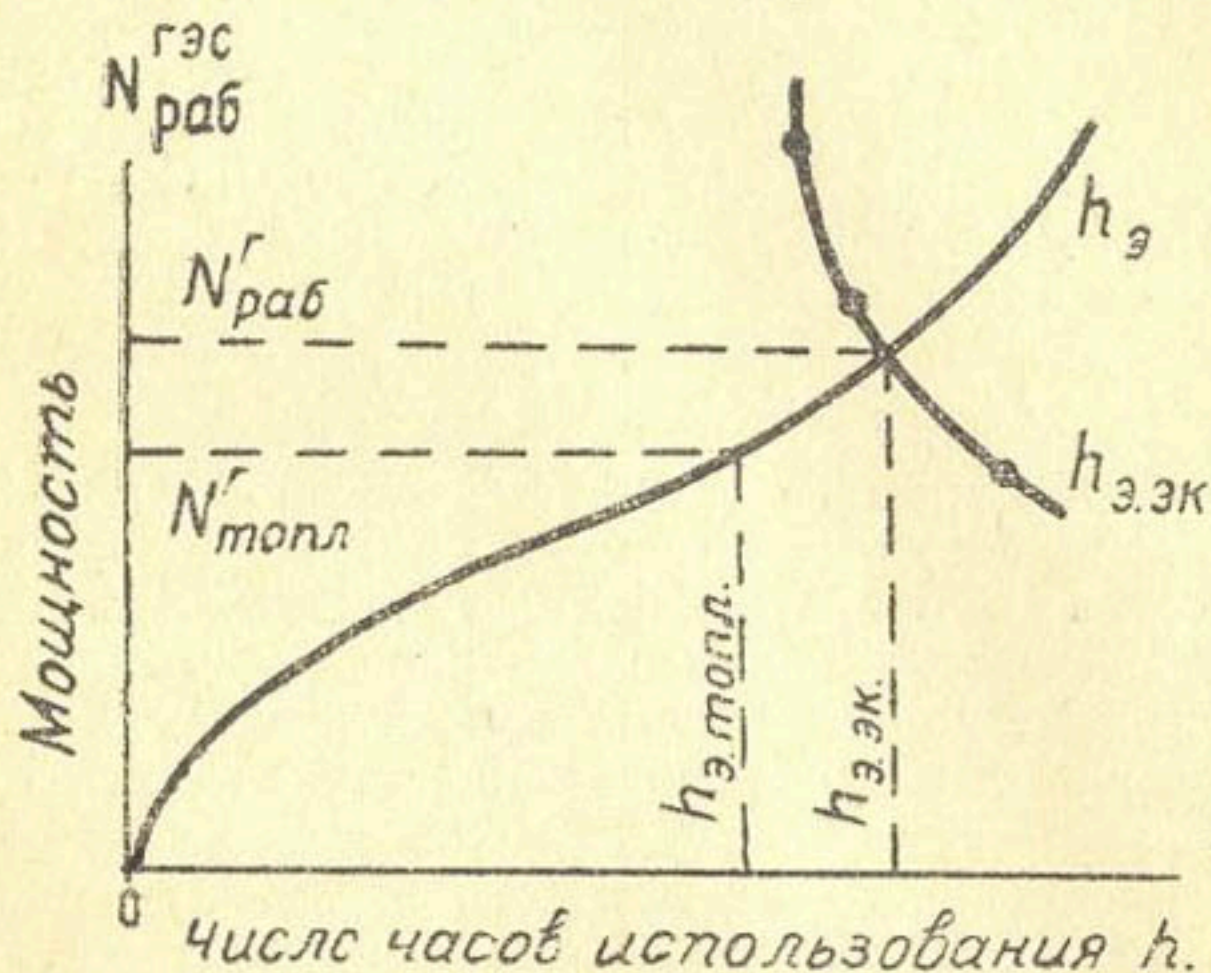
Рис. 46. Число часов использования дополнительного киловатта на специально пропускаемой для него воде в зависимости от величины рабочей мощности ГЭС.
