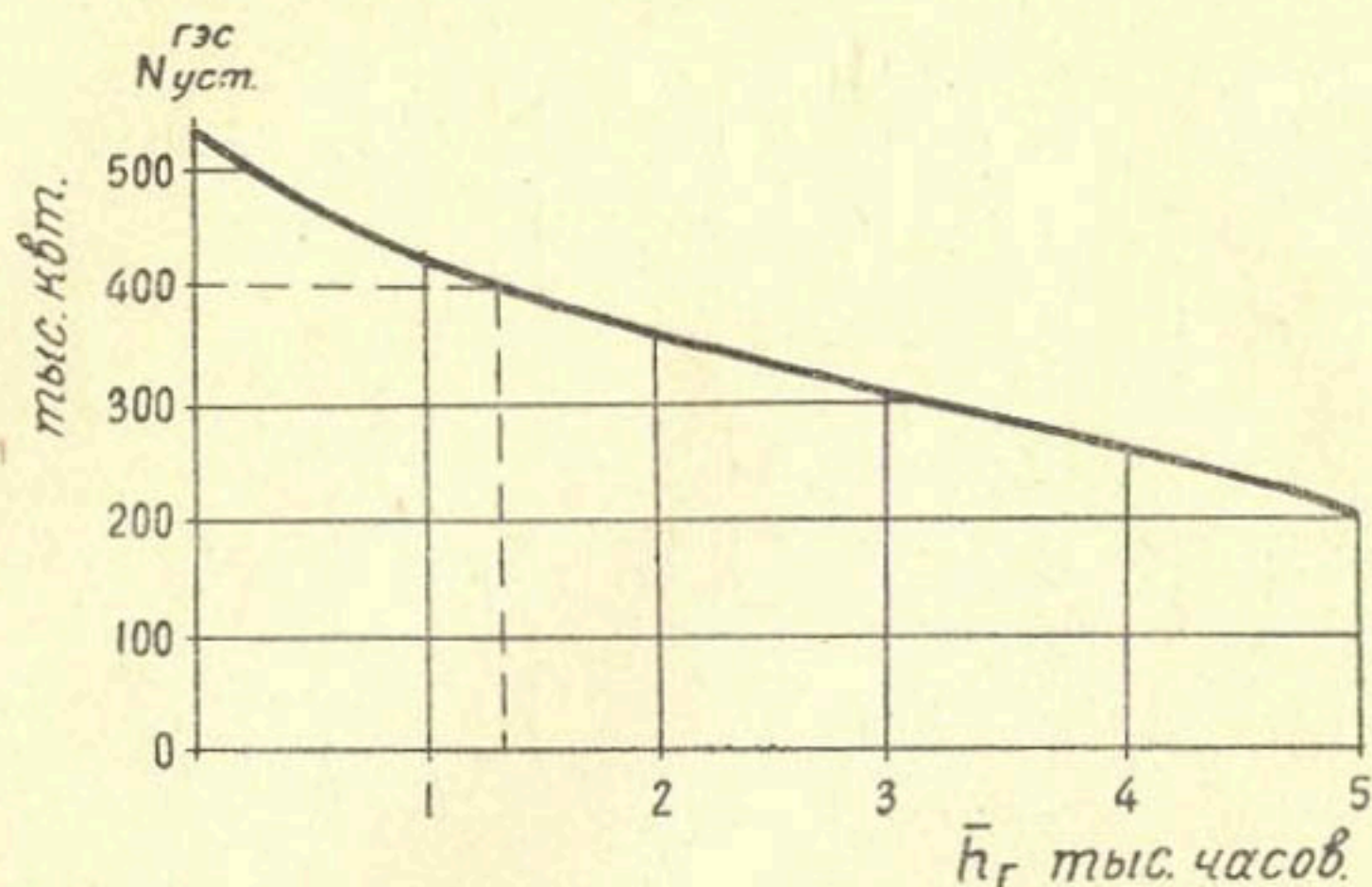
Рис. 37. Зависимость среднего многолетнего числа часов использования дополнительного киловатта \bar{h}_r от установленной мощности ГЭС N_{уст.}^{ГЭС}
