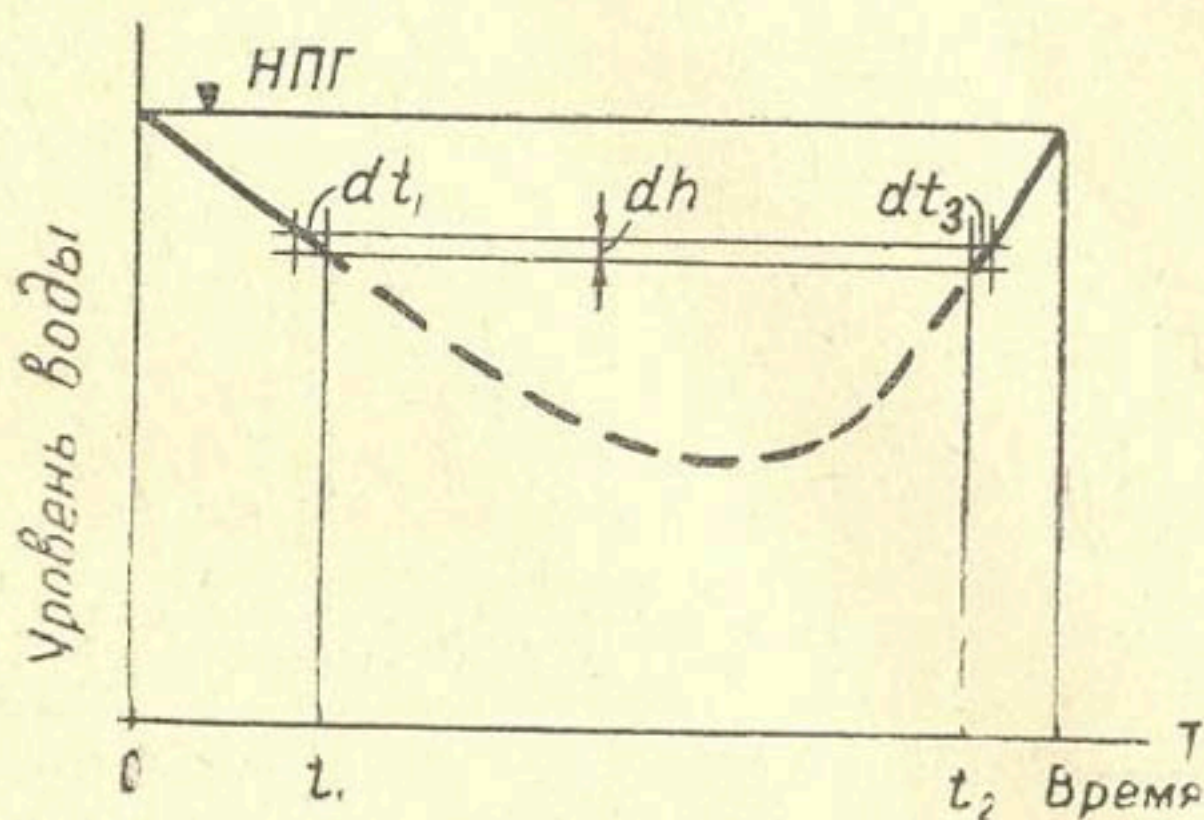
Рис. 23. К определению удельного прироста выработки энергии ГЭС при сработке ее водохранилища.
