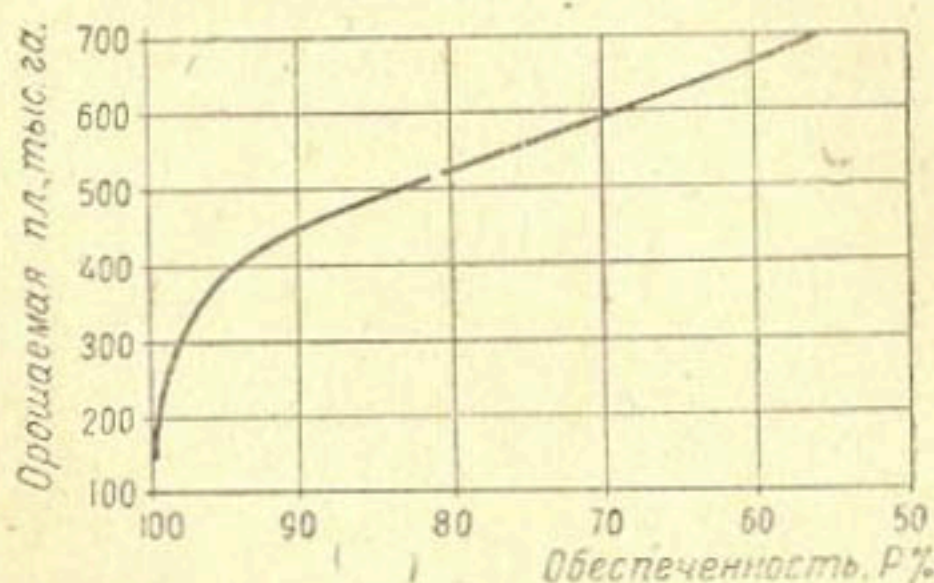
Рис. 33. Зависимость величины орошаемой площади от обеспеченности годового стока реки при оптимальной мощности проектируемой ГЭС (490 тыс. кВт).
