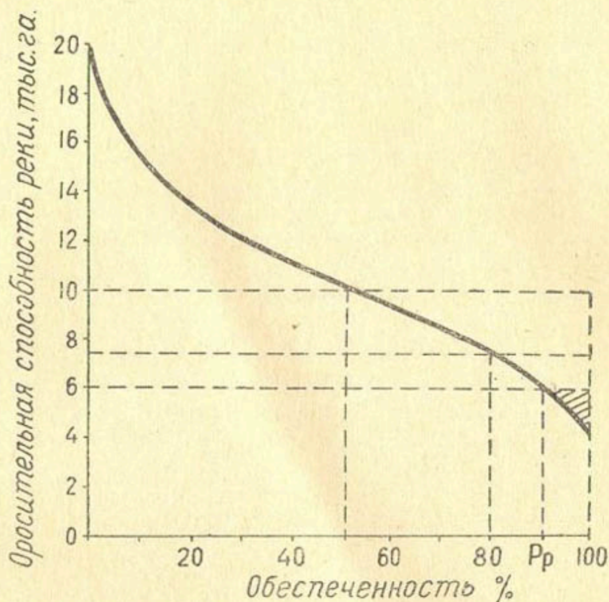
Рис. 8. Кривая обеспеченности площади орошения из проектируемого источника
