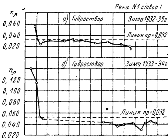
Рис. 123. График n_d = f(t) .
