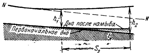
Рис. 58. Намыв на участке подпора.
