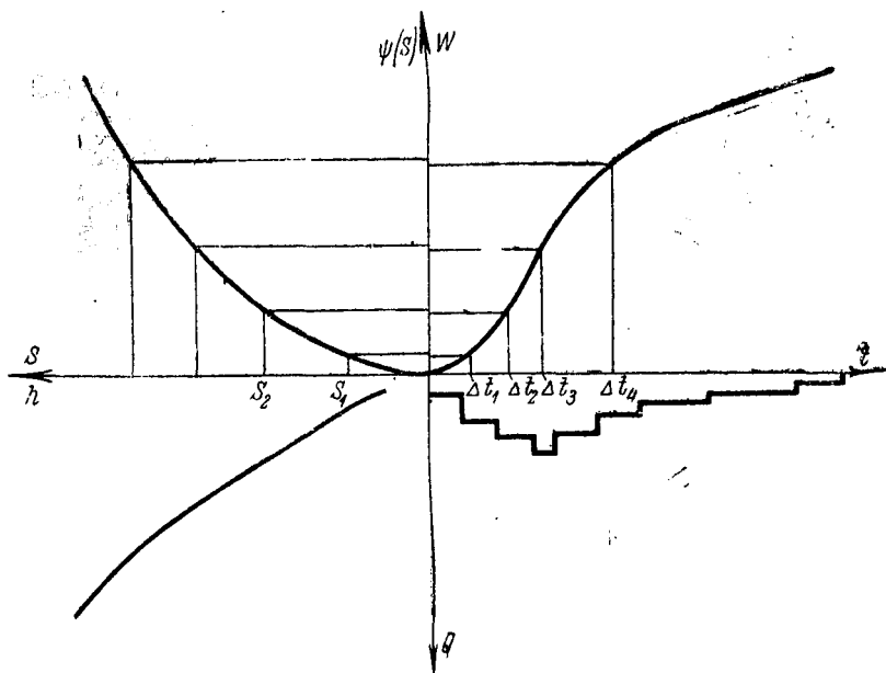
Рис. 102. Графический метод расчета продвижения гряды донных наносов при занесении подпертого бьефа.
