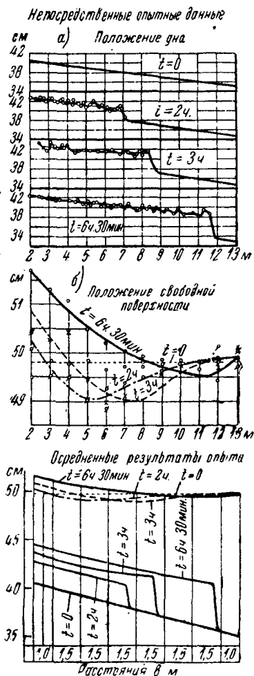
Рис. 98. Экспериментальное исследование занесения подпертого бьефа донными наносами.
