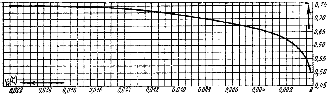
Рис. 86. \varphi_1(\zeta) .
