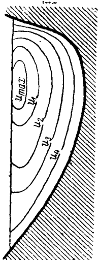
Рис. 49. Изотакхи скоростей в сечении водотока.
