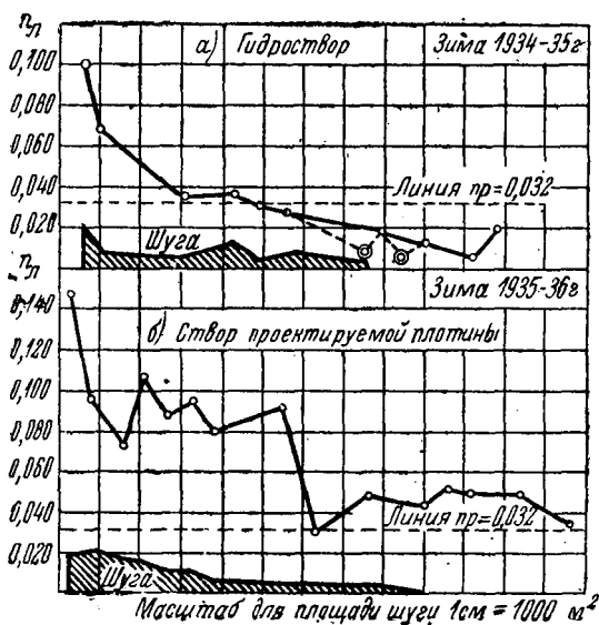
Рис. 125. График n_d = f(t) для шугоносного участка реки.
