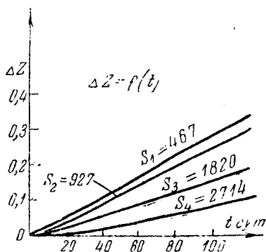
Рис. 90. График \Delta z = f(t, s) к примеру расчета заилиения дна водотока.
