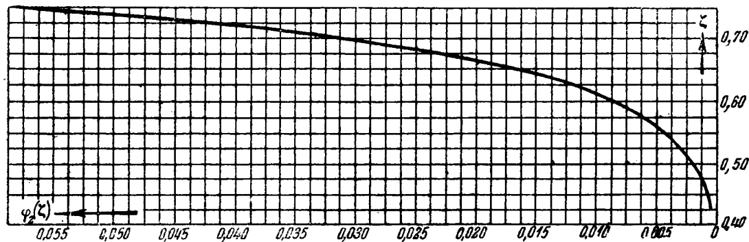
Рис. 87. \varphi_2(\zeta) .
