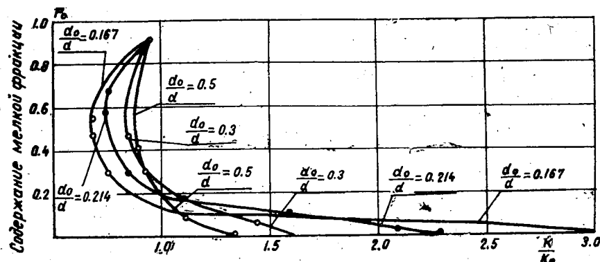
Рис. 2. Зависимость коэффициента фильтрации двухфракционной смеси от содержания мелкой фракции:
