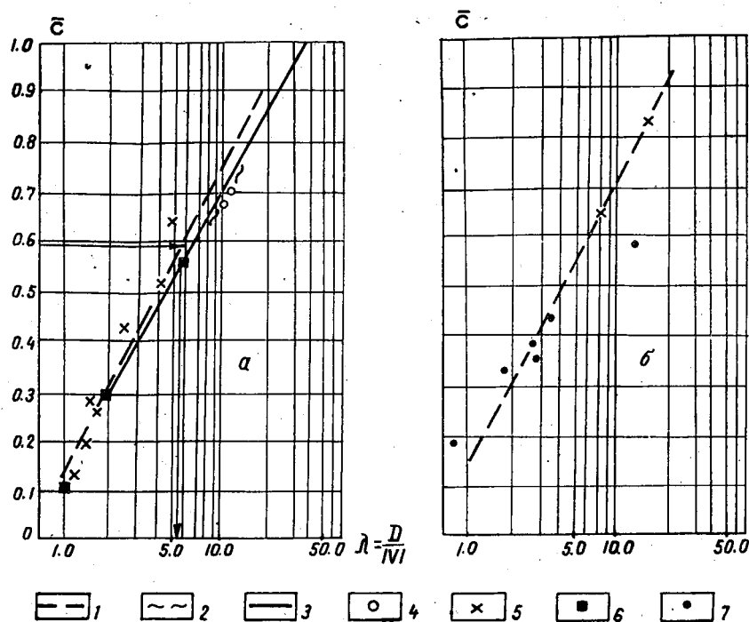
Рис. 2. Зависимость параметра среды \lambda от относительной концентрации \bar{C} :
