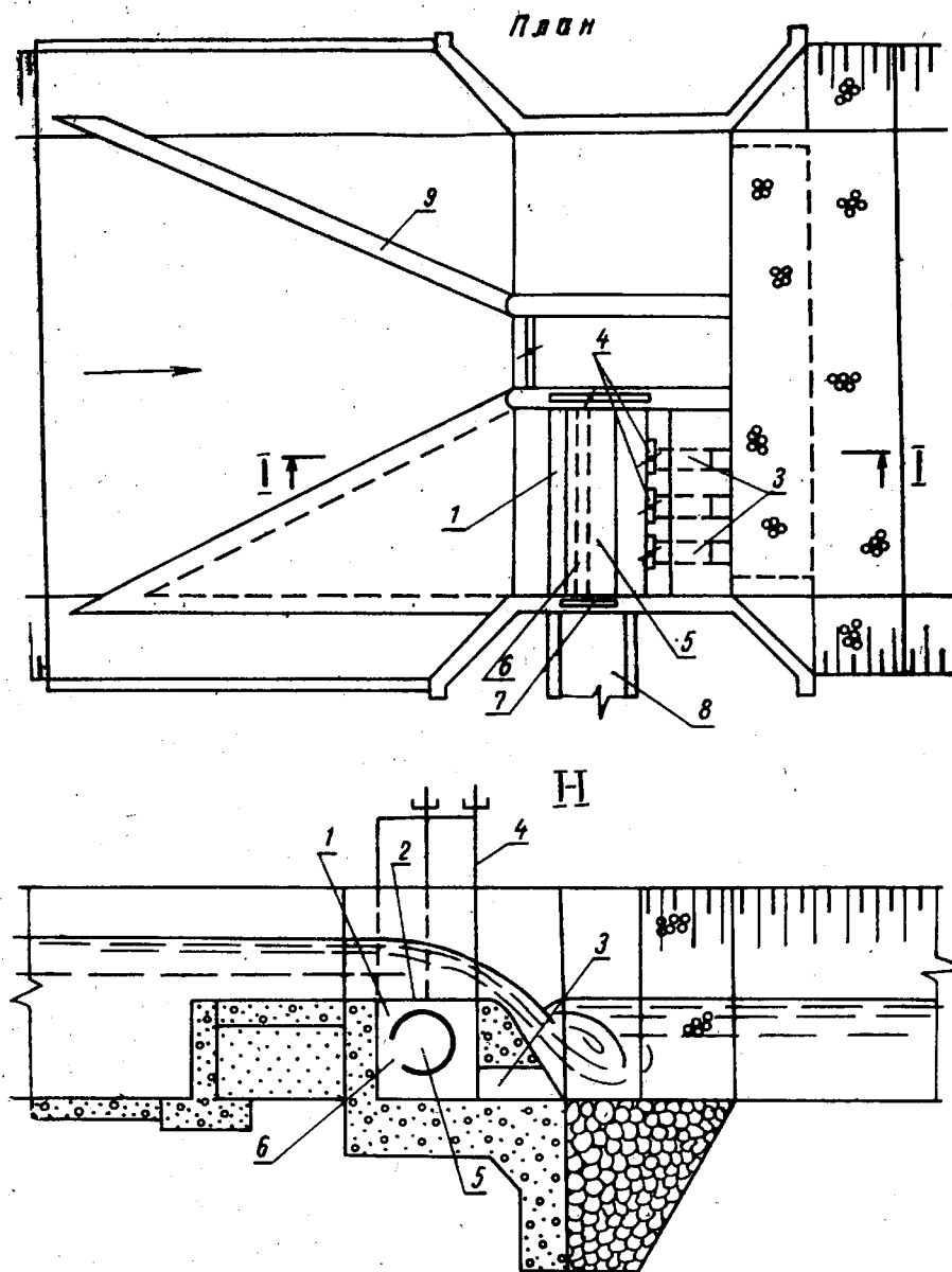
Рис. 3. Водозабор с совмещенным водоприемником — пескогравиеловкой:
