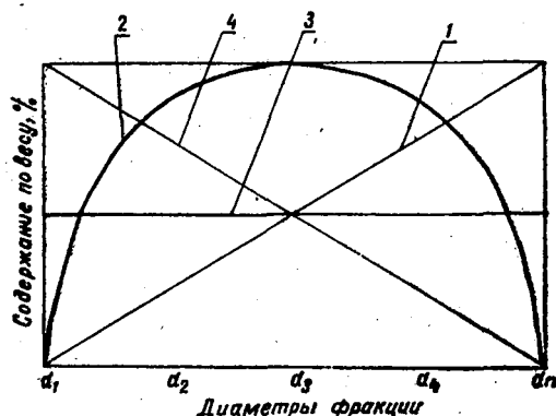
Рис. 5. Кривые распределения фракций: d_1, d_2, d_3, d_4 — диаметры отдельных фракций:
