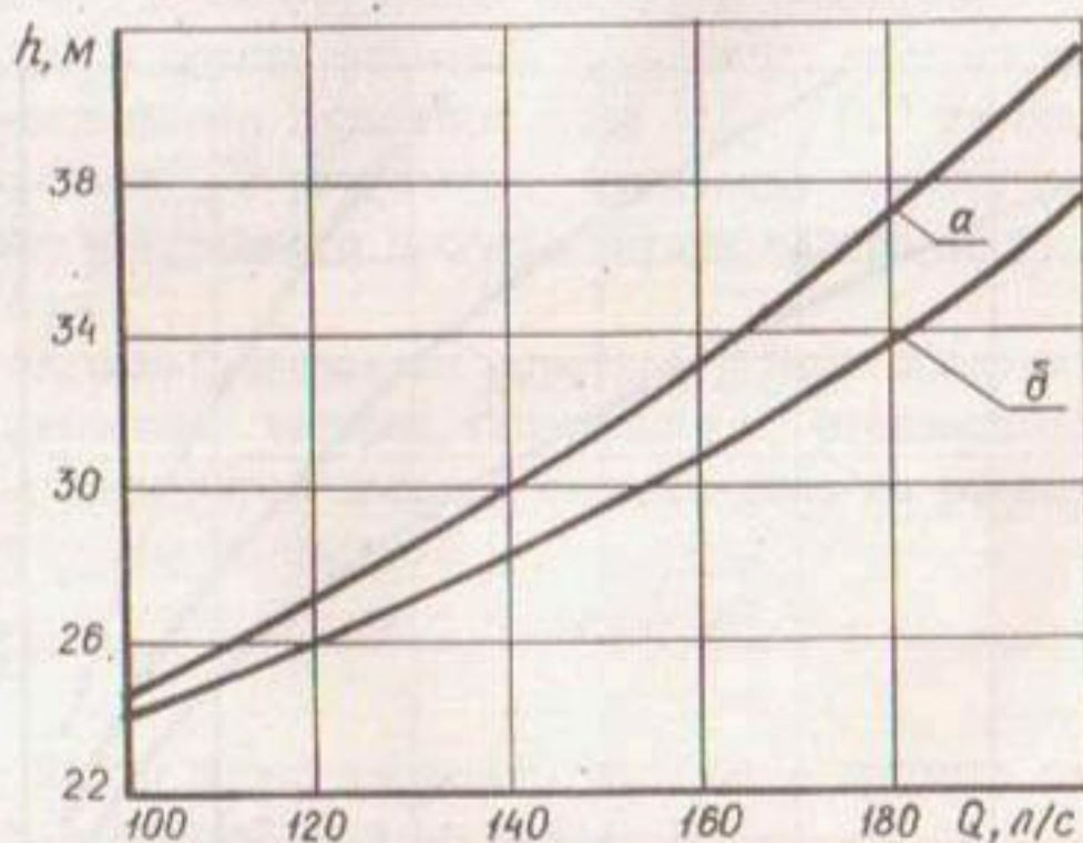
Рис.3. Характеристика напорного трубопровода машины: а, б - с внутренними диаметрами элементами трубопровода центрального пролета соответственно Ду 150 и 200 мм
