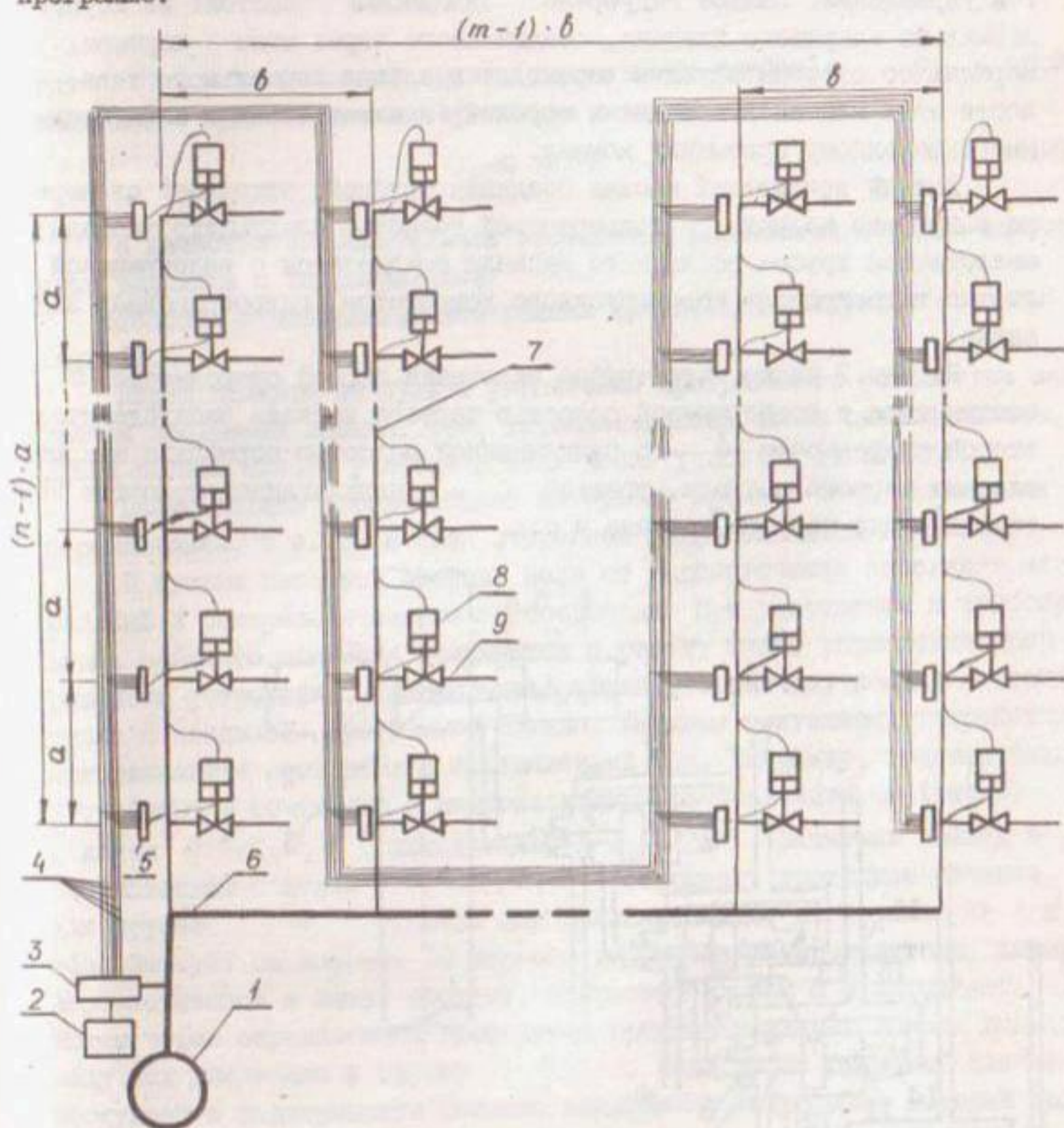
Рис. I. Многоканальная схема индивидуального управления запорными органами с гидроприводом: 1 - насосная станция; 2 - пульт управления; 3 - задатчик команд; 4 - управляющие трубки; 5 - многокаскадный приемник команд; 6 - магистральный трубопровод; 7 - распределительный трубопровод; 8 - гидроприводная задвижка; 9 - поливной трубопровод
