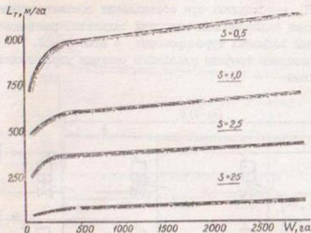
Рис. 3. Удельный расход управляющей трубки для многоканальной схемы индивидуального управления запорными органами с гидроприводом: — — — — при соотношении сторон 1:1; — — — — при соотношении сторон 1:2; — — — — при соотношении сторон 1:5; — — — — при соотношении сторон 1:10
