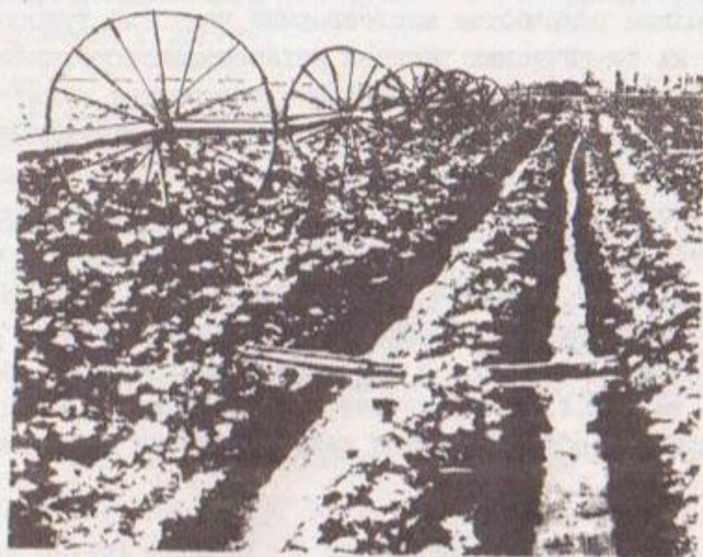
Рис.2. Колесный трубопровод ТКІ-90 в работе
