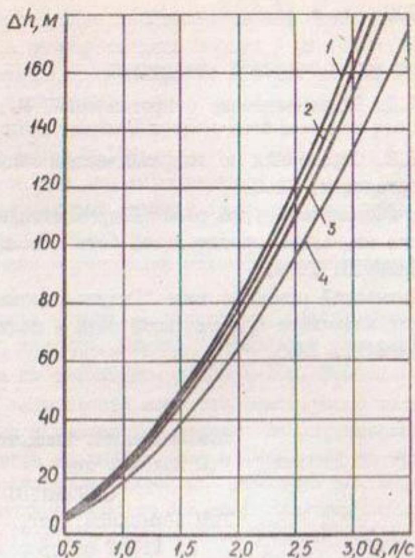
Рис. 4. Зависимость потерь напора (на 100 м) от расхода для полиэтиленового шланга d_{\text{вн}} = 24,5 мм с разными диаметрами навивки: 1 - d_{\text{н}} = 1 м; 2 - d_{\text{н}} = 1,5 м; 3 - d_{\text{н}} = 2 м; 4 - гладкий участок
