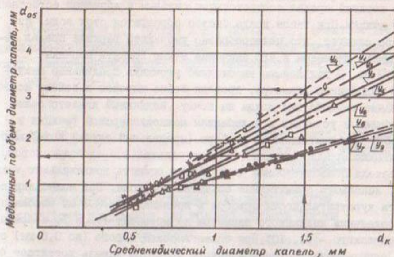
Рис.6. Связь медианного и среднекубического диаметров: y_1(\circ) - "Роса-3М"; y_2(*) , y_3(\circ) , y_4(+) - "Роса-2М"; y_5(\square) , y_6(\triangle) - "Роса-1"; y_7(\odot) , y_8(\oplus) , y_9(\diamond) - насадка; — — — ключ по определению диапазона допустимого медианного диаметра
