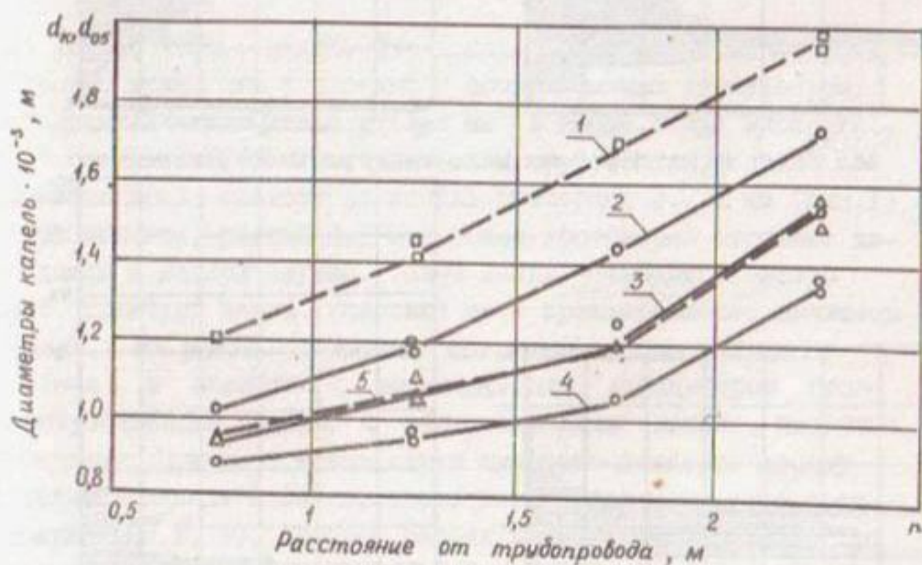
Рис. 4. Характер изменения крупности капель насадки с ложкообразным дефлектором при d_c = 6,5 \cdot 10^{-3} \text{ м} : □, Δ - медианный диаметр капель (1 - H = 5 \text{ м} ; 3 - H = 7,5 \text{ м} ; 5 - H = 10 \text{ м} ); o - среднекубический диаметр капель (2 - H = 5 \text{ м} ; 4 - H = 10 \text{ м} )
