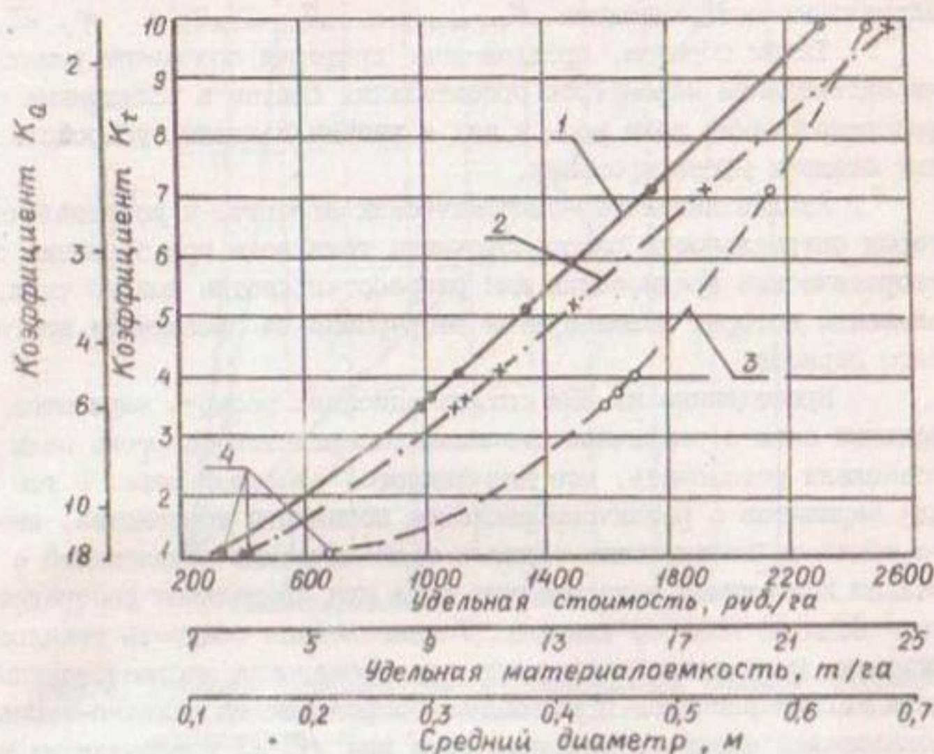
Рис 3. Графики зависимостей технико-экономических показателей сети для поверхностного орошения от коэффициентов K_t и K_d : 1 – удельная стоимость сети; 2 – удельная материалоемкость сети; 3 – средний диаметр сети; 4 – сеть с АППУ
