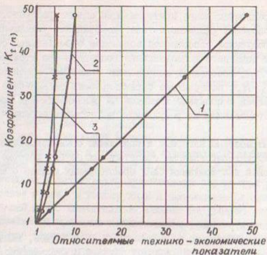
Рис. 4. Графики зависимостей относительных технико-экономических показателей водовода 1-ого порядка от коэффициента K_{tn} :
