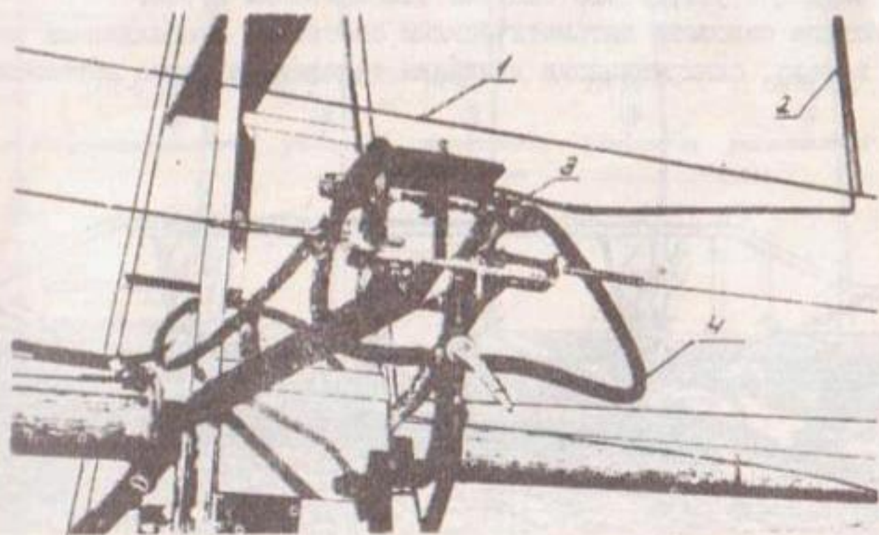
Рис. I. Узел синхронизации движения тележек ДМФ: 1 — управляющий трос; 2 — рычаг; 3 — регулируемый клапан; 4 — гибкий рукав к гидроцилиндру
