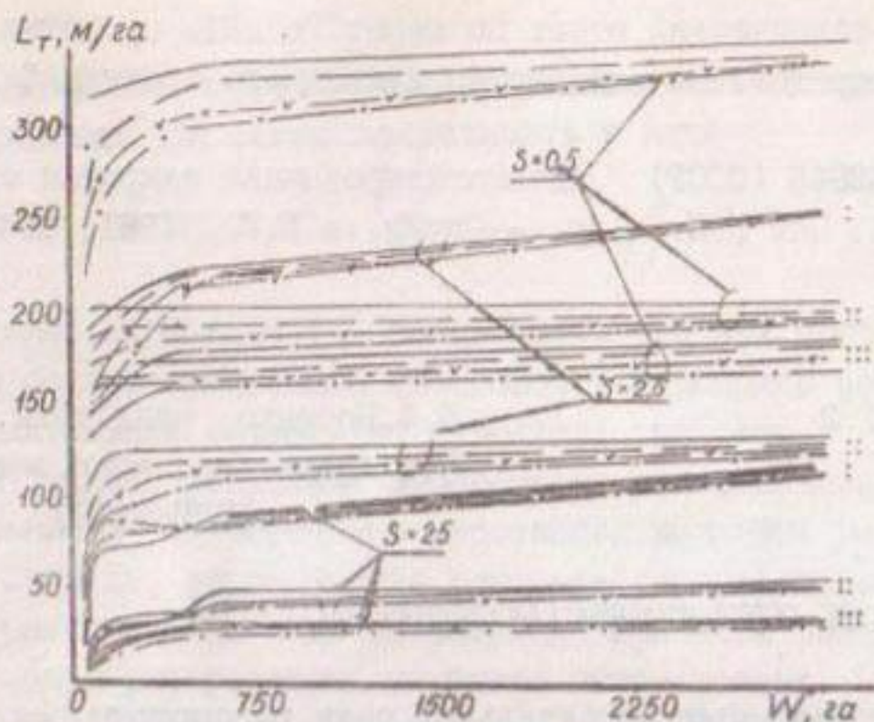
Рис.7. Удельный расход управляющей трубки для многоканальной схемы дистанционного управления группой запорных органов с гидроприводом: — при соотношении сторон 1:1; --- при соотношении сторон 1:2; —·— при соотношении сторон 1:5; ..... при соотношении сторон 1:10
