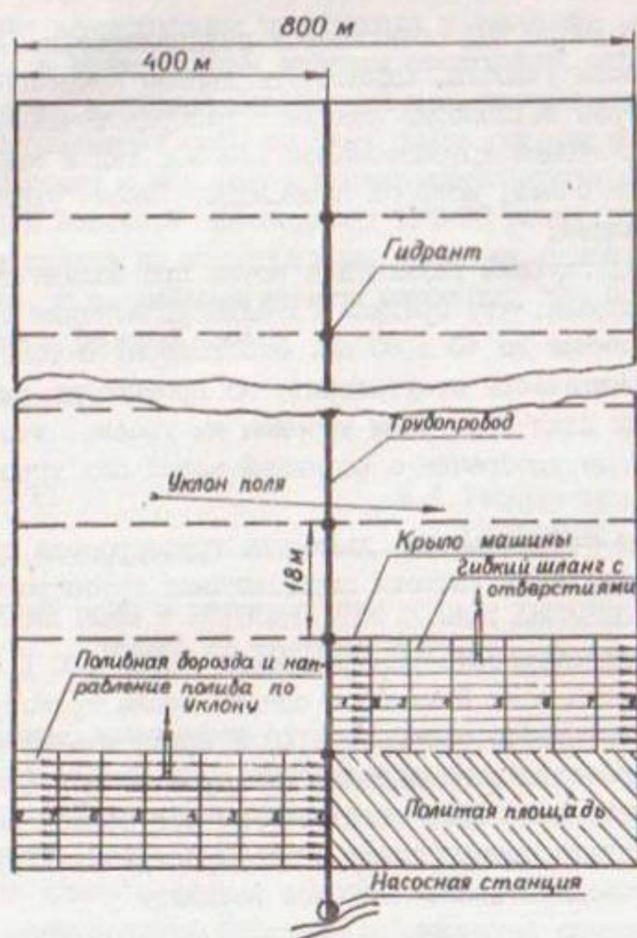
Рис.3. Схема полива
