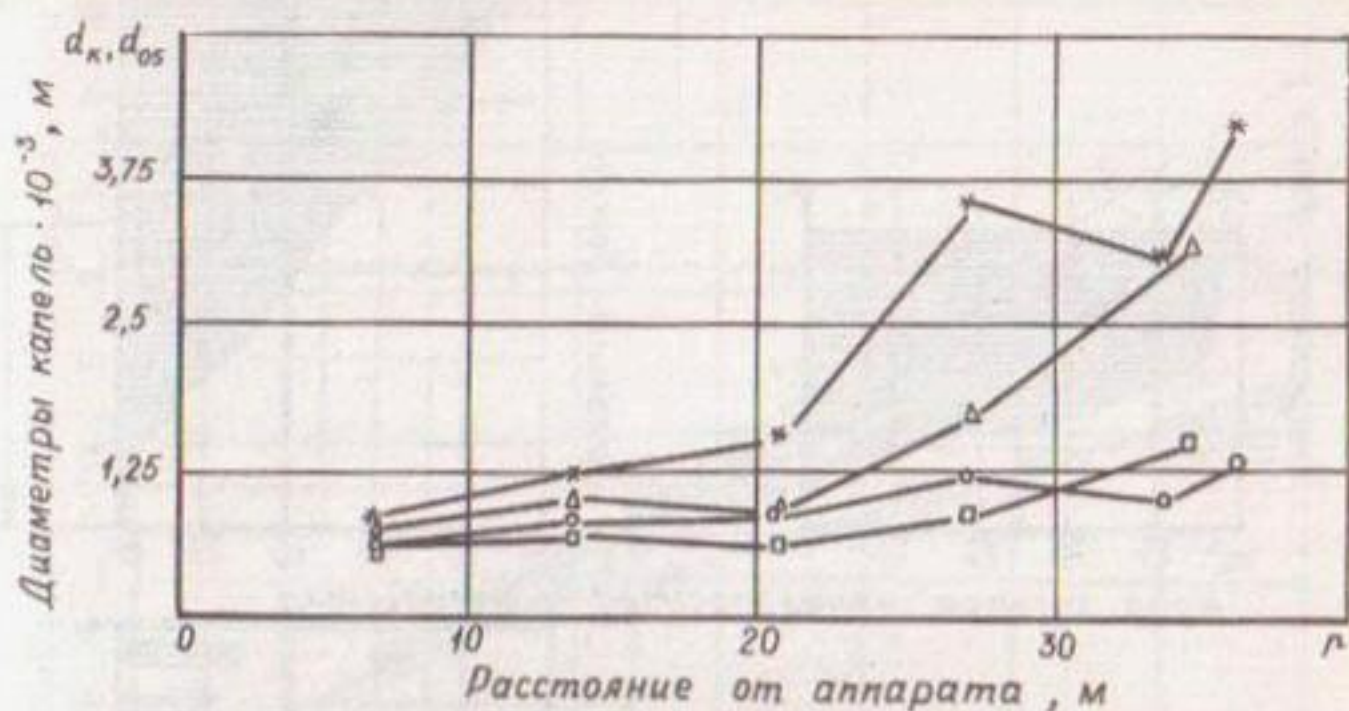
Рис. 3. Характер изменения крупности капель аппарата "Роса-3М" при диаметре сопла d_c = (7; 18; 4) \cdot 10^{-3} \text{ м} : o - среднекубический диаметр; * - медианный диаметр при H = 45 \text{ м} ; □ - среднекубический диаметр; Δ - медианный диаметр при H = 60 \text{ м}
