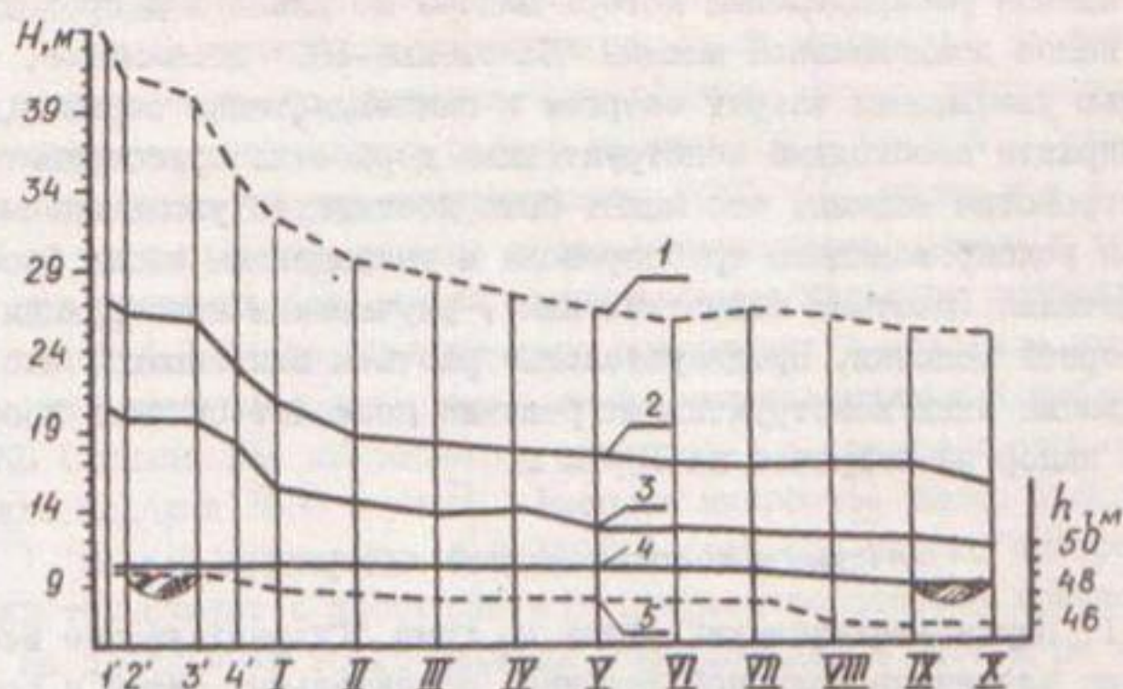
Рис. 5. Распределение напора H (1, 2, 3) и отметок поверхности земли h_z (4, 5) по длине водопроводящего пояса ДМ "Коломенка-100"
