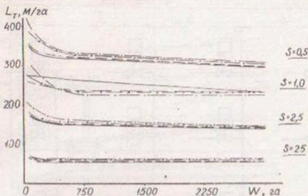
Рис.5. Удельный расход управляющей трубки при комбинированной (многоканальная и матричная) схеме дистанционного управления запорными органами с гидроприводом: — — — — при соотношении сторон 1:1; — — — — при соотношении сторон 1:2; — v — при соотношении сторон 1:5; — . — — при соотношении сторон 1:10
