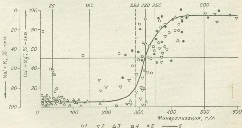
Рис. 7.8. Зависимость катионного состава от степени минерализации рассолов. Солёные воды и рассолы Ангаро-Ленского артезианского бассейна: 1 — терригенной формации 2 — солёной формации, 3 — карбонатной формации, 4 — надсолёных отложений; 5 — рассолы из других регионов; 6 — линия средних значений.
