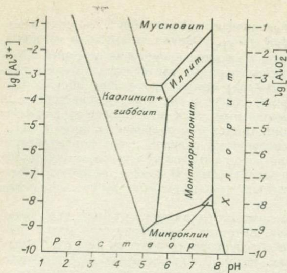
Рис. 4.2. Соотношения растворенных соединений алюминия с гиббситом, каолинитом, иллитом и монтмориллонитом при различных значениях pH.
