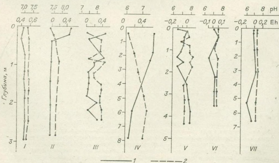
Рис. 7.3. Распределение значений Eh и pH в разрезе осадков Тихого океана (I), Алеутского жёлоба и Аляскинского залива (II), склона Северной Америки (III) и в иловых растворах Индийского океана (IV), Черного (V) и Каспийского (VI, VII) морей; 1 — Eh; 2 — pH.
