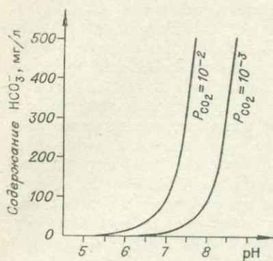
Рис. 6.2. Соотношение между содержанием иона \text{HCO}_3^- в растворе и величиной pH.
