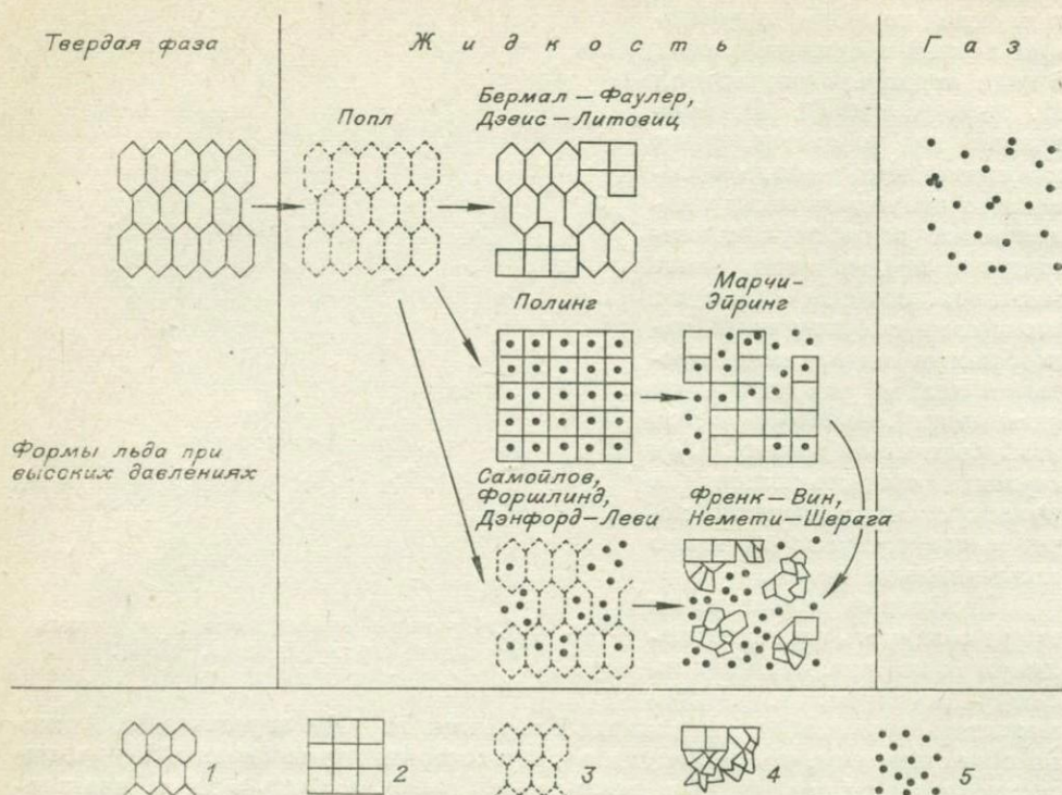
Рис. 1.6. Строение воды в представлении различных авторов.
