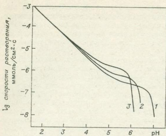
Рис. 4.1. Зависимость скорости растворения кальцита от величины pH и P_{\text{CO}_2} при 25°C
