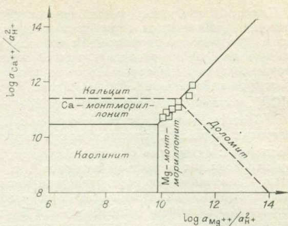
Рис. 4.7. Система CaO — MgO — Al 2 O 3 — SiO 2 — CO 2 — HCl — H 2 O при 75°C, lg [H 4 SiO 4 ] = -3,4 и P CO2 = 10 3 Па с нанесением данных по составу термальных вод района Абано, Италия [Norton, Panichi, 1977].
