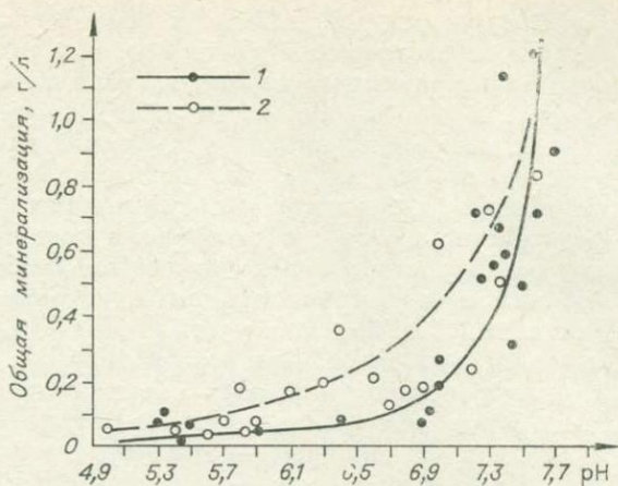
Рис. 6.3. Зависимость между величиной pH и общей минерализацией подземных вод. Области: 1 — умеренного климата, 2 — тропического.
