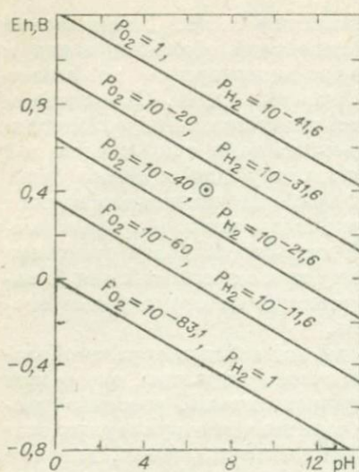
Рис. 1.7. Пределы устойчивости свободной воды, выраженные в виде функции Eh и pH при 25^\circ C и 1 атм общего давления с указанием местоположения точки абсолютной нейтральности.
