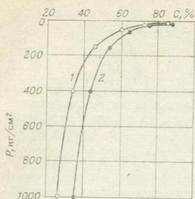
Рис. 3.6. Вынос солей из глин при гравитационном выщелачивании по двум экспериментам [Коротков, Павлов, 1972].
