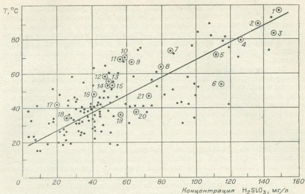
Рис. 6.10. Зависимость содержания кремнекислоты от температуры [Барабанов, Дислер, 1968]. Термальные источники:
