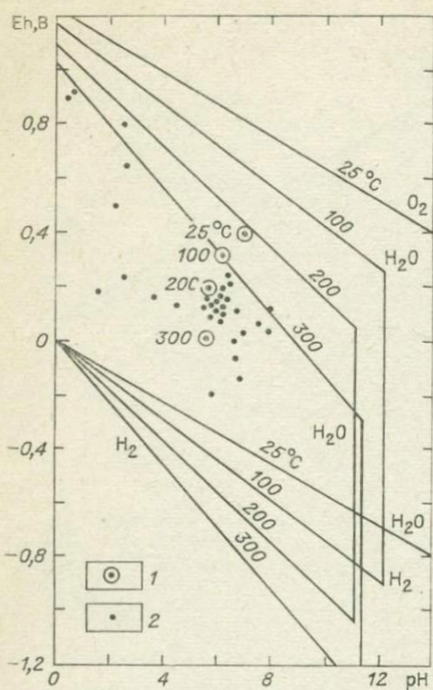
Рис. 1.9. Пределы устойчивости свободной воды в координатах pH — Eh при различных температурах и давлениях насыщенного пара.
