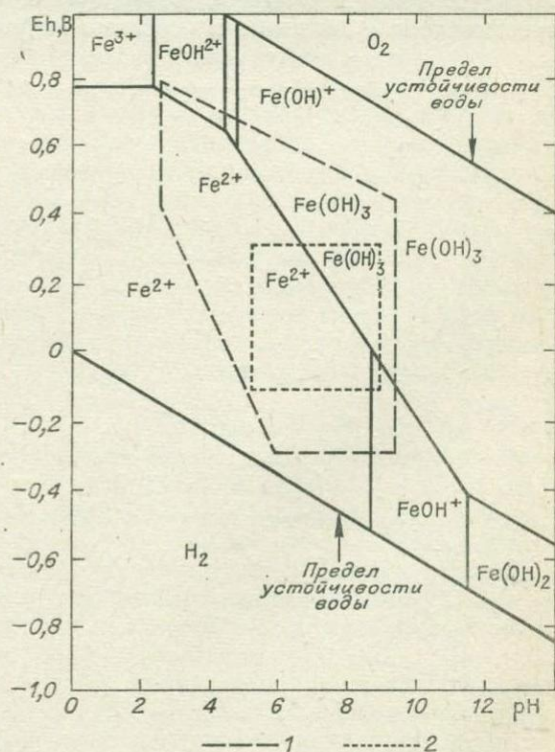
Рис. 3.2. Поля устойчивости окислов железа на pH — Eh-диаграмме.
