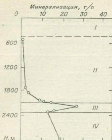
Рис. 6.4. Изменение минерализации подмерзлотных вод с глубиной в Намской опорной скважине, Якутия (по Р. С. Кононовой).
