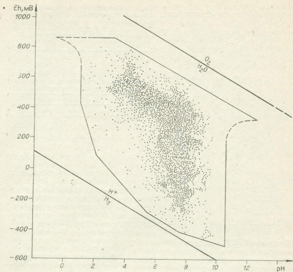
Рис. 1.8. Распределение значений Eh и pH природных водных сред [Баас-Беккинг и др., 1963].
