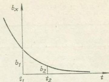
Рис. 5.3. Изменение содержания элемента x в системе при постоянной величине интенсивности миграции P_x .
