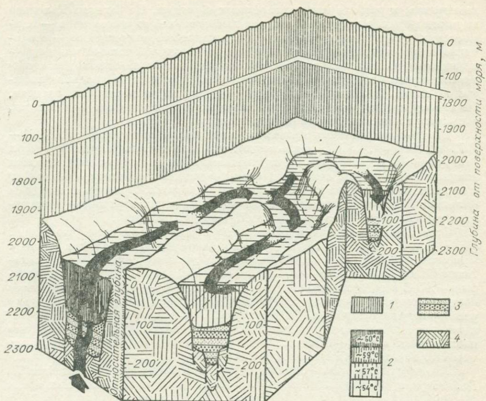
Рис. 8.4. Конвективные течения термальных рассолов во впадине Атлантик II [Shoell, 1976].
