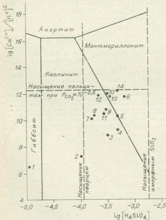
Рис. 4.5. Система \text{HCl} - \text{H}_2\text{O} - \text{Al}_2\text{O}_3 - \text{CaO} - \text{CO}_2 - \text{SiO}_2 при 25^\circ\text{C} с нанесением данных по среднему составу подземных вод различных ландшафтных зон.
