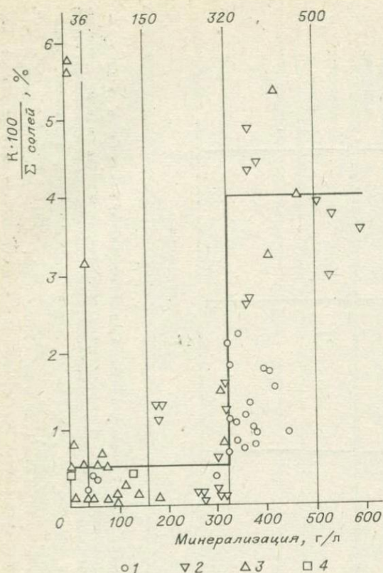
Рис. 9.3. Зависимость процентного содержания калия от минерализации рассолов Ангара-Ленского бассейна.
