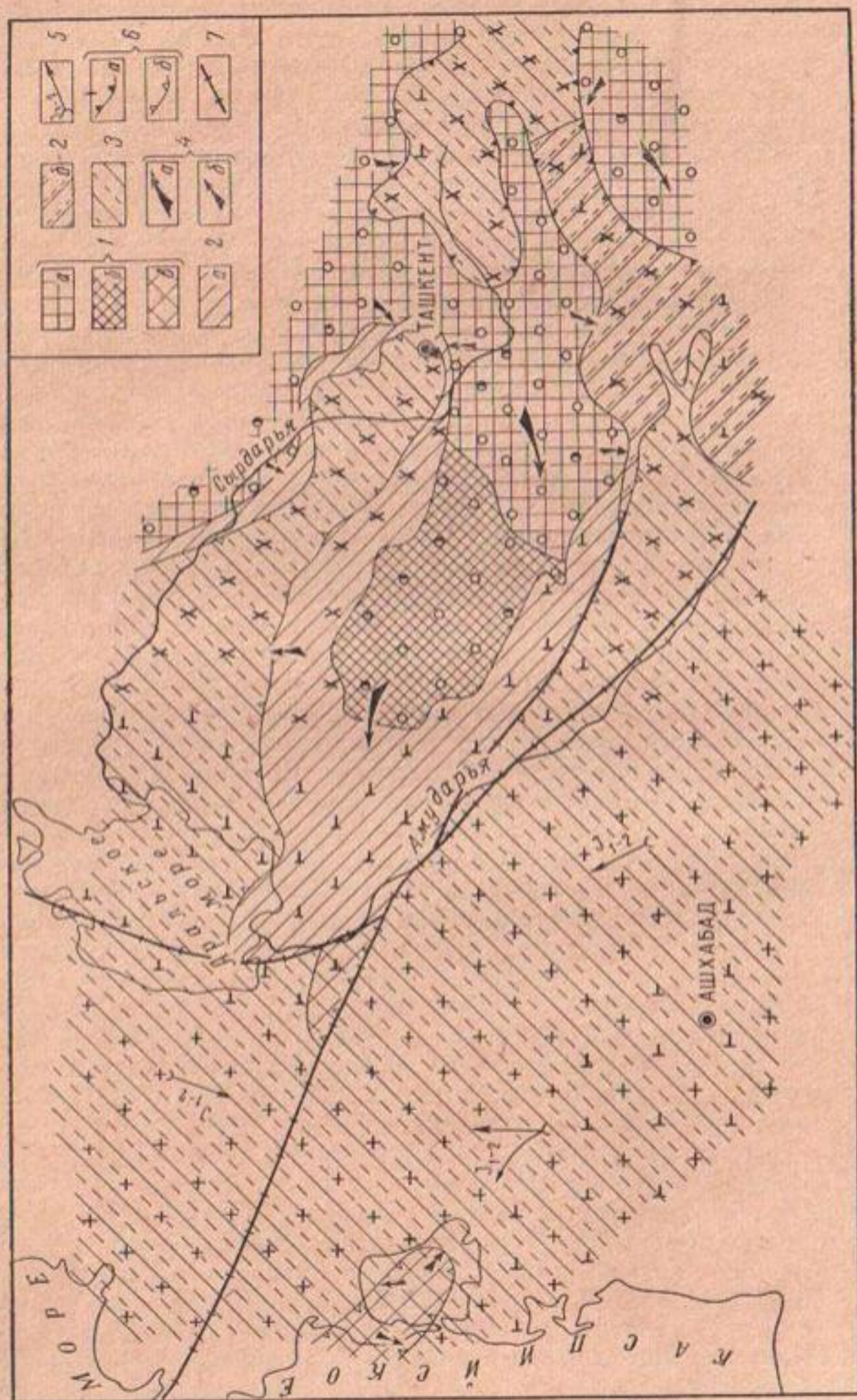
Рис. 5. Палеогеогеологическая схема раннего мела (неоком)
