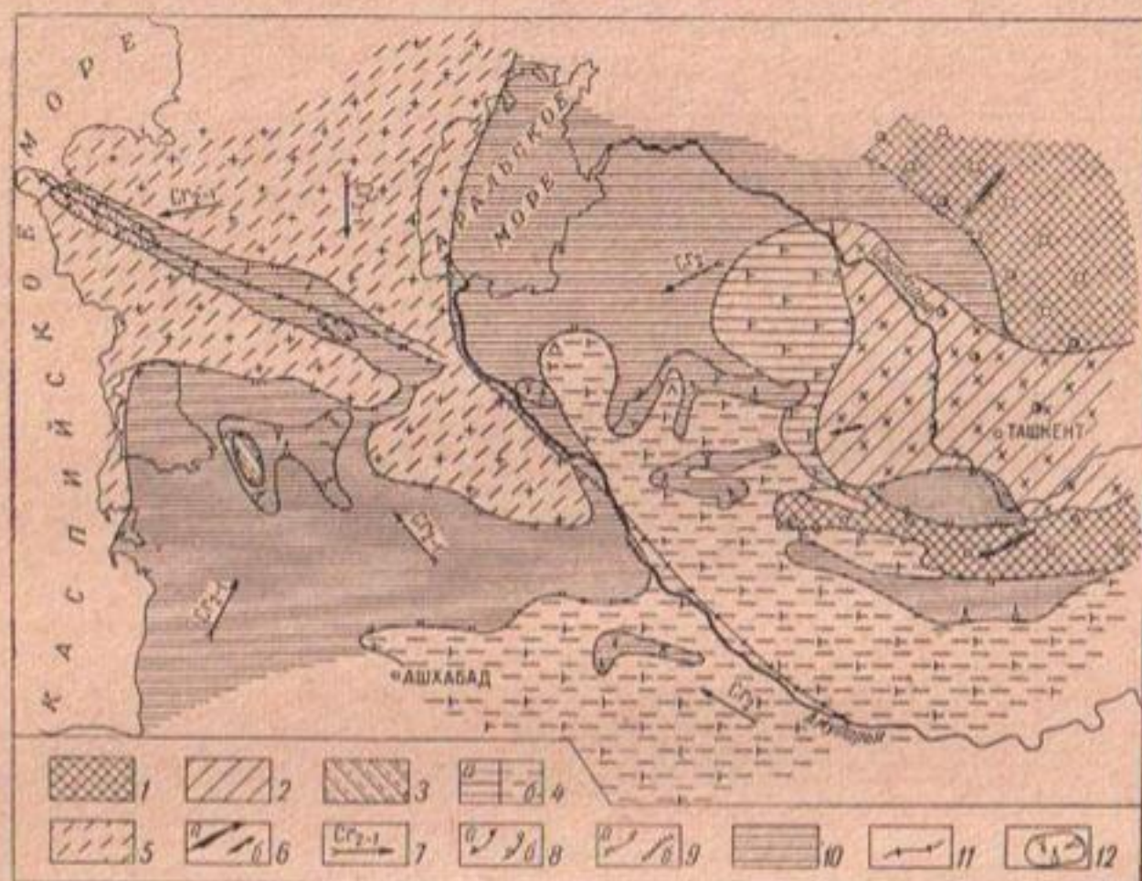
Рис. 10. Палеогидрогеологическая схема олигоцена
