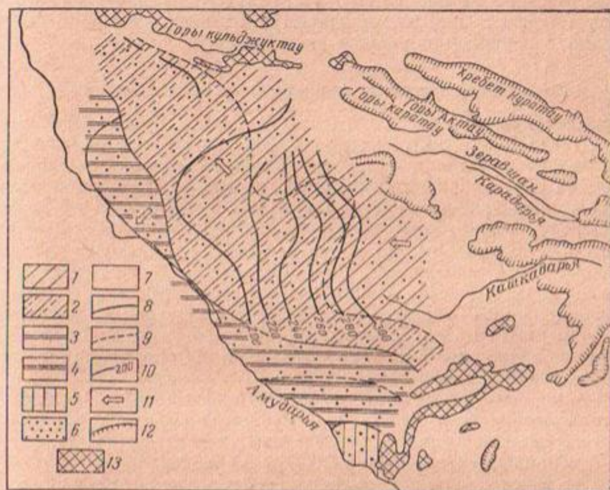
Рис. 22. Схематическая карта гидрогеохимических зон и гидродинамических условий палеоцен-верхнетуронского водоносного комплекса Бухаро-Каршинского артезианского бассейна. Составил Л. Е. Михайлов
