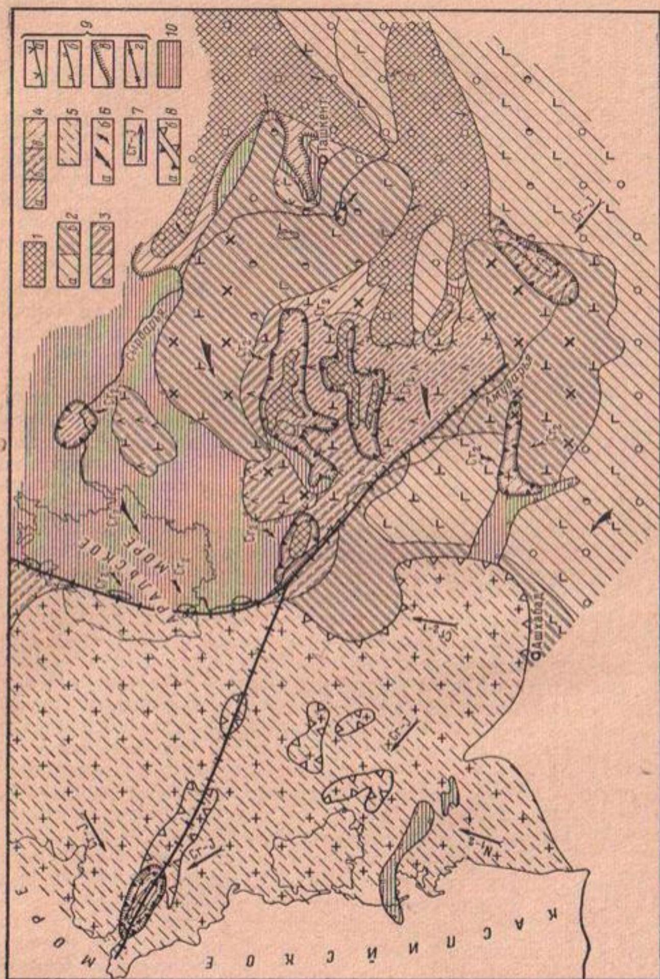
Рис. 13. Палеогеологическая схема верхнего миоцена
