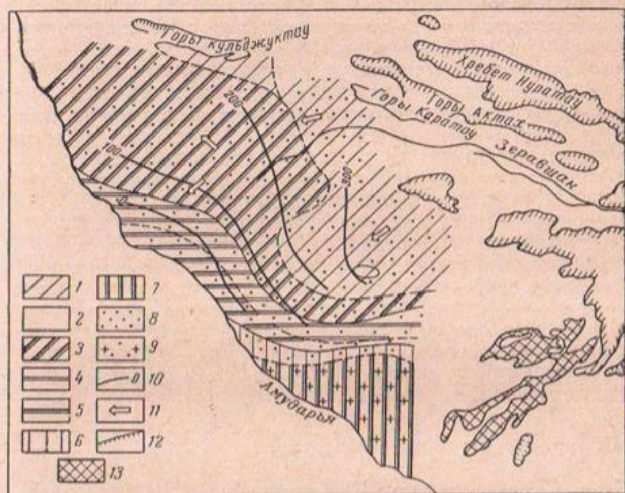
Рис. 23. Схематическая карта гидрогеохимических зон и гидродинамических условий сеноманских отложений (X пронизываемый горизонт) Бухаро-Каракумского артезианского бассейна. Составил Л. Е. Михайлов
