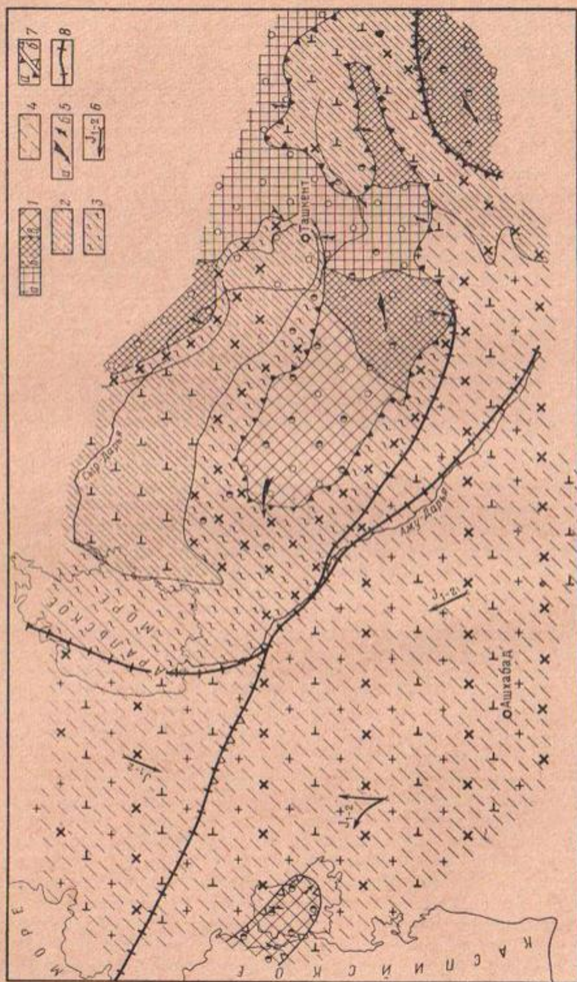
Рис. 6. Палеогеологическая схема ант-альба
