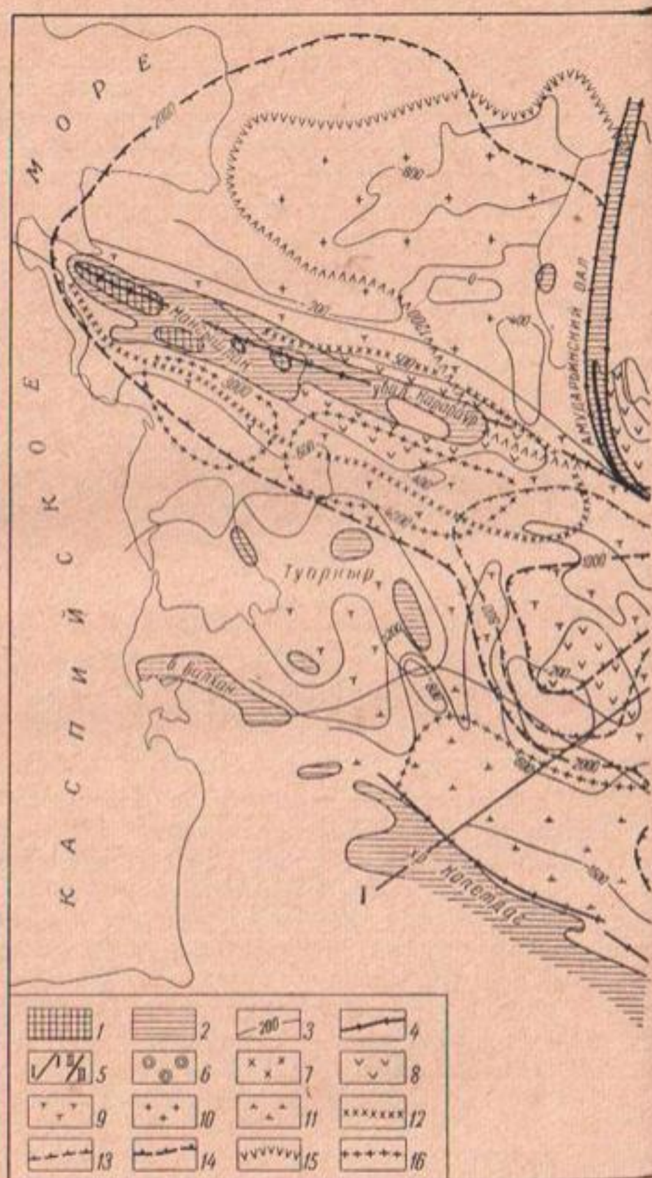
Рис. 26. Гидрохимическая схема под
