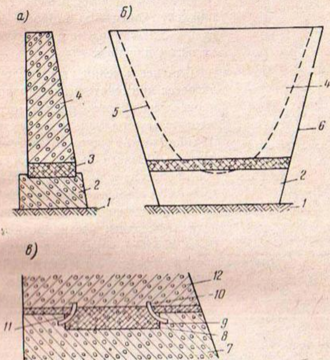
К анн. 7. Арочная плотина с пластичным элементом а—поперечное сечение арочной плотины; б—фасад; в—шов (деталь); 1—основание; 2—фундамент; 3, 9—пластичный элемент; 4—арочная плотина; 5—линия естественного рельефа; 6—врезка; 7, 12—отдель- ные элементы (арки); 8—паз; 10, 11—уплотнение.
