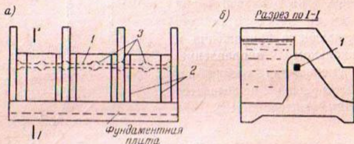
К анн. 11. Бетонная плотина на неоднородном основании а — продольный разрез; б — разрез по I-I; 1 — разгружающая балка; 2 — температурные полушвы; 3 — места анкерования разгружающей балки.
