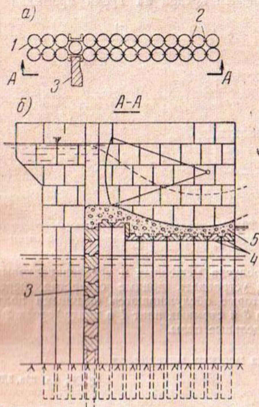
К анн. 19. Водосливная плотина из сборных элементов
