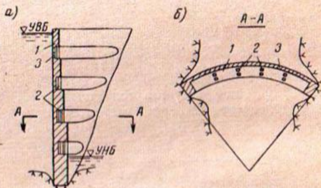
К анн. 2. Арочная плотина „на столбах“ а—разрез; б—план по А—А; 1—арочные элементы; 2—столбы; 3—напорное перекрытие.
