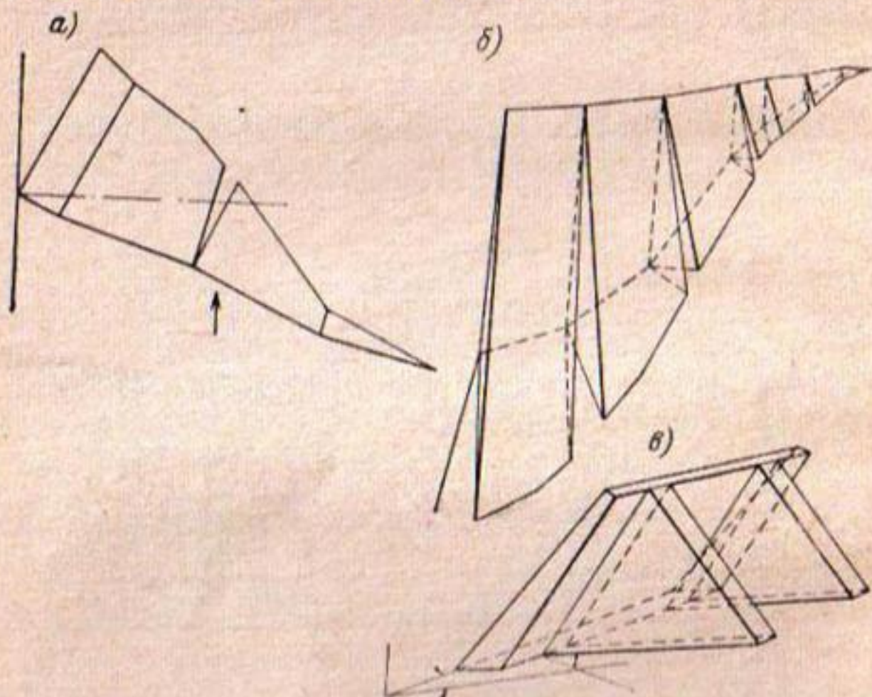
К анн. 14. Плотина с ломаной осью в плане а — план плотины, состоящей из секций; б — аксонометрия; в — вариант секции контрфорсного типа.
