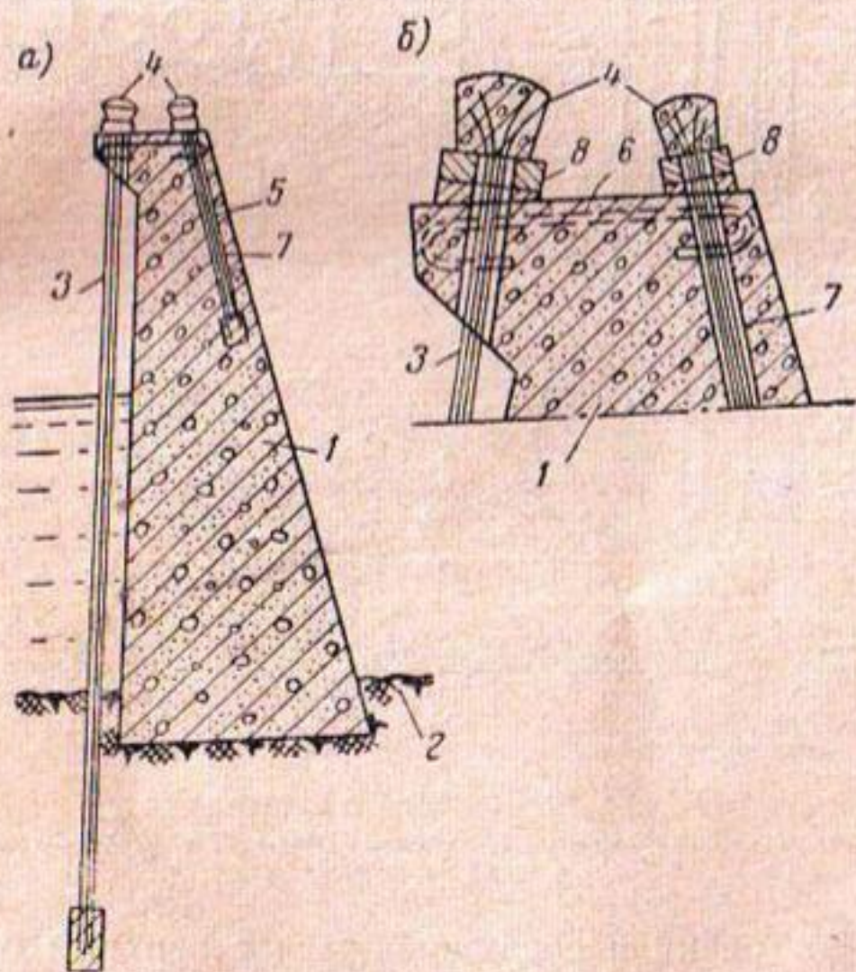
К апп. 15. Предварительно напряженная плотина а—поперечный разрез; б—деталь; 1—плотина; 2—основание; 3—тяж; 4—анкерующий блок; 5—канал; 6—арматура гребня; 7—вспомогатель- ный тяж; 8—шайба.
