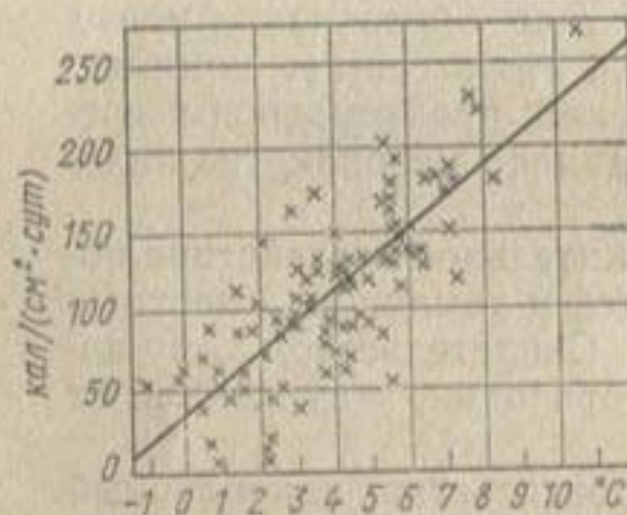
Рис. 3. График зависимости потери тепла от разности температур поверхности воды и атмосферы для октября. × — данные измерений.
