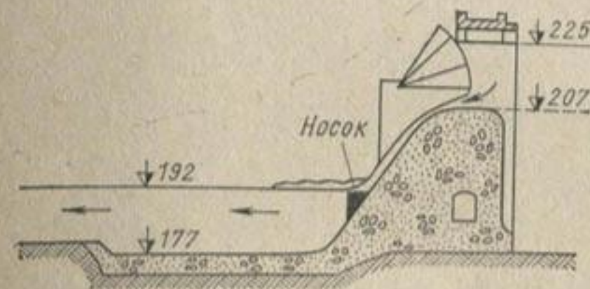
Рис. 9. Профиль водослива, рекомендуемый для плотины Лоуер-Гранит.
