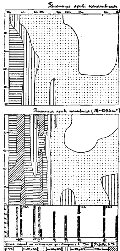
Диаграмма № 16. Динамика влажности в метровом слое под яровой пшеницей 1929 г.
