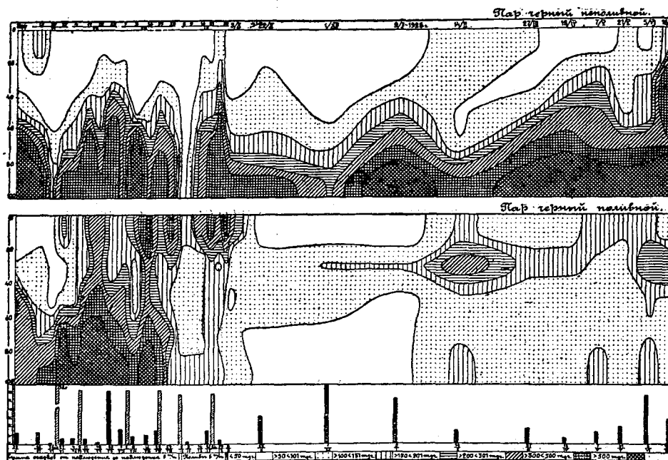
Диаграмма № 73. Динамика хлора в метровом слое почвы на черном пару 1927/28 гг.
