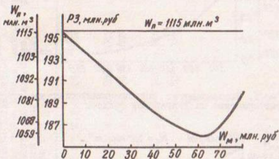
Рис.4. Эквивалентная водноэкономическая характеристика по Актыбинской области
