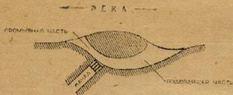
Рис. 6. Схема водозабора с вспомогательным криволинейным каналом
