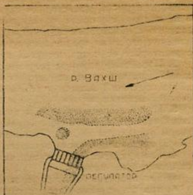
Рис. 12. Схема отложений донных наносов при отсутствии бара ниже поперечника № 4. Положение регулятора 1-ое Q реки = 220 м. 3 /сек., q канала = 100 м. 3 /сек.
