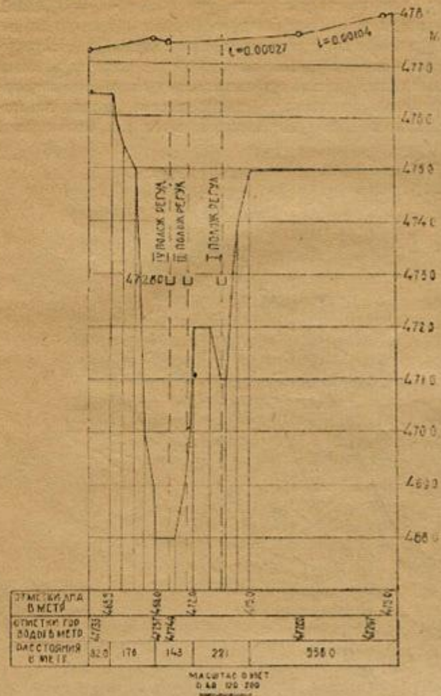
Рис. 3. Продольный профиль
