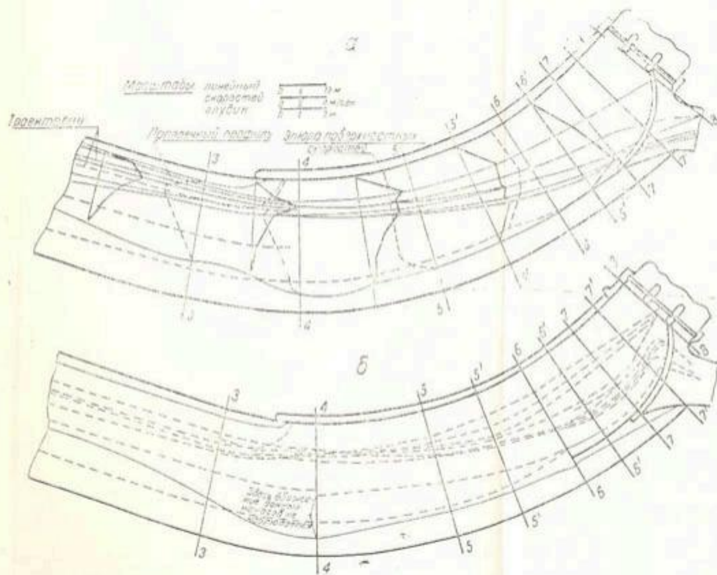
Рис. 38. План траекторий поверхностных струй и знаки поверхностных скоростей в подводящем русле (а), направление глубинных токов (б), профили горизонтов воды и дна (в).
