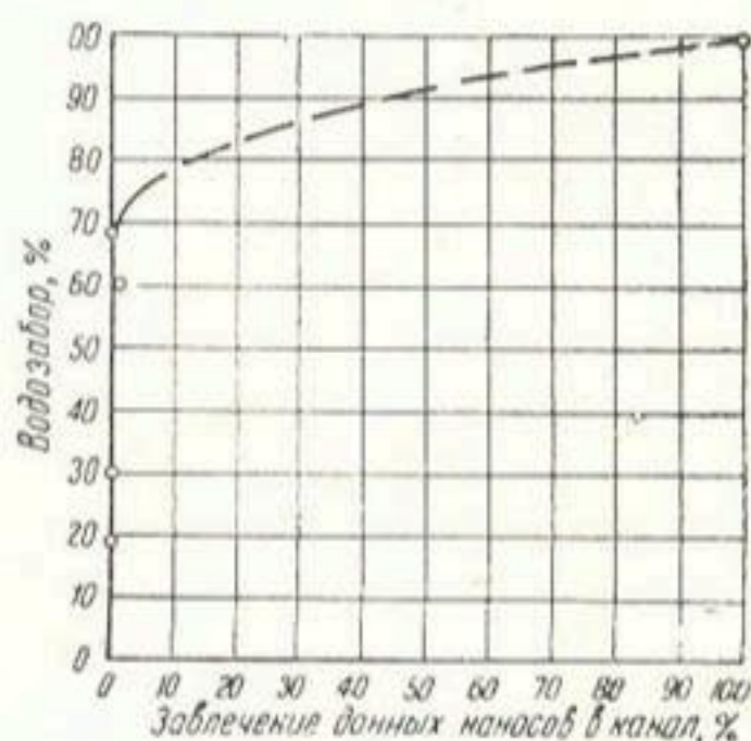
Рис. 34. Кривая зависимости завлечения донных наносов в канал от водозабора на модели Камыр-Раватского гидроузла (1940—1941 гг.).
