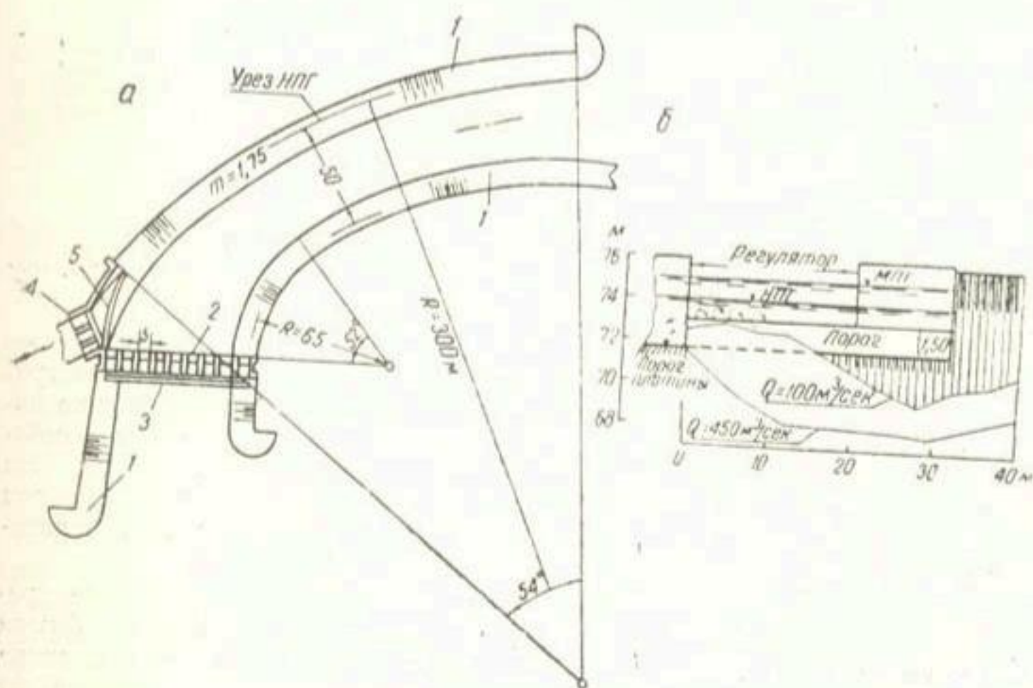
Рис. 17. Плотина Арысь-Туркестанского канала на р. Арысь. а — план: 1 — струенаправляющие дамбы, 2 — плотина, 3 — предохранительная плоскость, 4 — регулятор, 5 — вазо- приемный порог. б — профили дна через водоприемник с повышенным прямоугольным порогом (движе- ние напоя через порог показано пунктирными стрелками).
