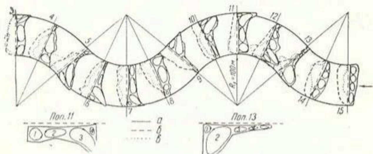
Рис. 3. Схема вертикальных течений в извилистом русле с размываемым дном и неразмываемыми берегами.
