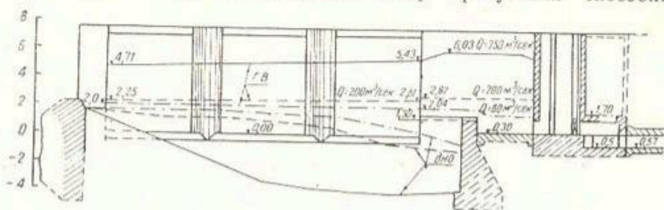
Рис. 31. Поперечные профили водной поверхности и дна в верхнем бьефе Ангренского гидроузла. Горизонты воды относятся к створу по линии носов бычков плотины.
