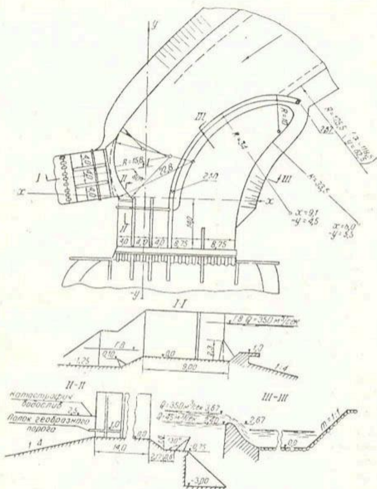
Рис. 28. Тупалаангский гидроузел на р. Каратаг (план и разрезы модели).
