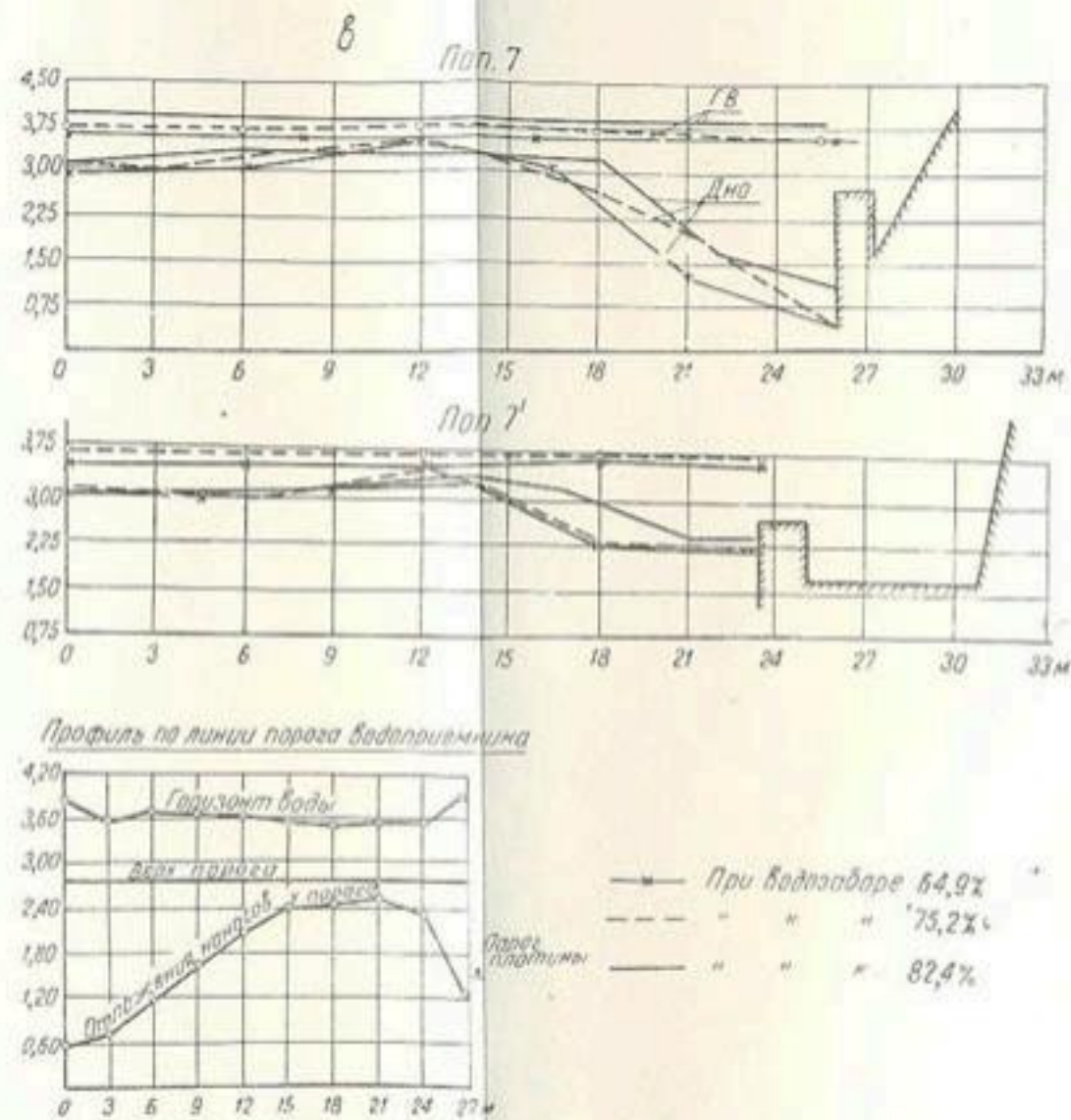
Рис. 38. План траекторий поверхностных струй и знаки поверхностных скоростей в подводящем русле (а), направление глубинных токов (б), профили горизонтов воды и дна (в).
