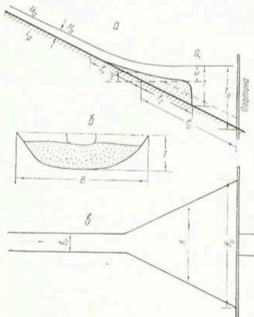
Рис. 43. Расчетная схема.
