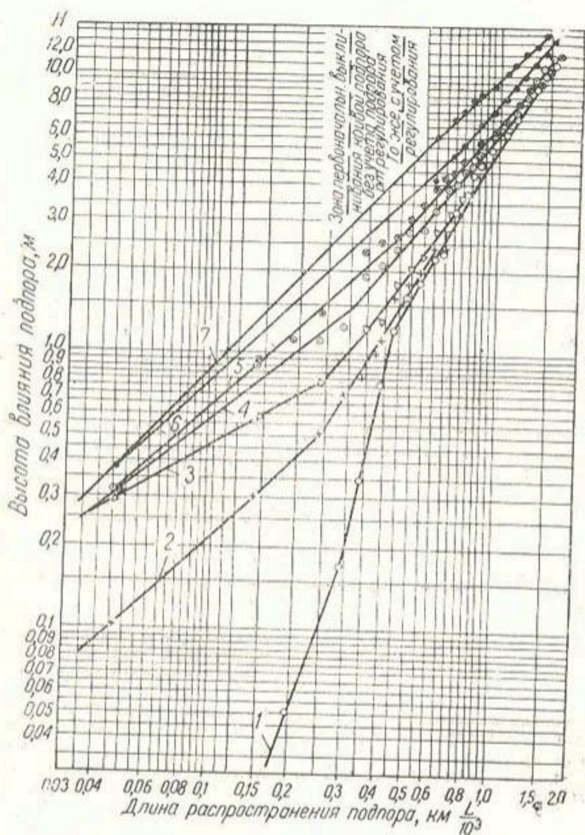
Рис. 53. Кривые изменения горизонтов воды в подпертом бьефе при средненаводковом расходе ( Q = 160 \text{ м}^3/\text{сек} ) по мере его формирования; I_0 = 0,0034 , \Delta H = 3,80 \text{ м} , подпертый бьеф руслового типа зарегулирован, B = 30-60 \text{ м} (модель).
