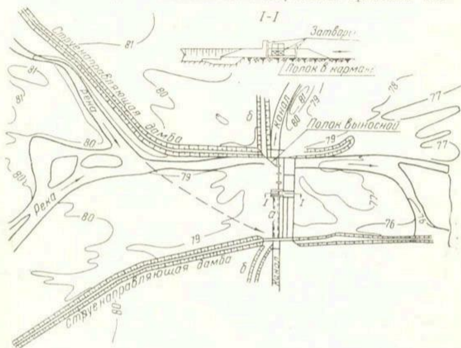
Рис. 13. Схема двустороннего водозабора на горной реке с делением потока по широте (русло XI 1938 г.). Вверху водозабор в разрезе. а — водосливная плотина с потерной в реку, б — водоудержательные дамбы.
