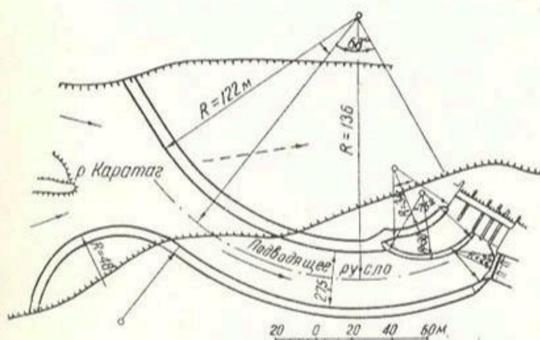
Рис. 10. План головного сооружения Тупалаинского канала на р. Каратаг (лабораторное проектирование).
