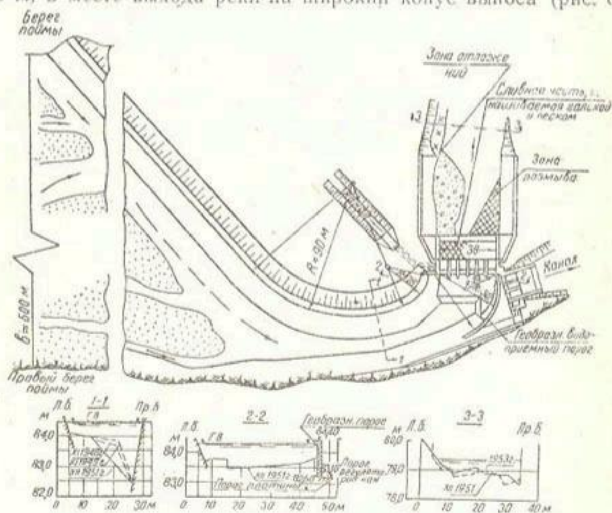
Рис. 8. Сары-Курганский водозаборный узел на р. Сох.
