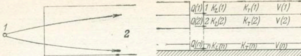
Рис. 4.2.19. Односкважинный геоэлектрический метод. Определение моделируемой области.
