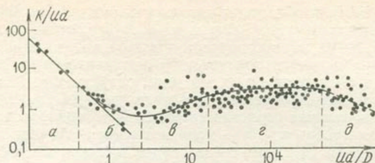
Рис. 2.4.3. Различные режимы дисперсии по экспериментальным данным. \alpha — чисто молекулярная дисперсия; \beta — переходный режим; \gamma — преобладание механической дисперсии; \delta — дисперсия за пределами закона Дарси
