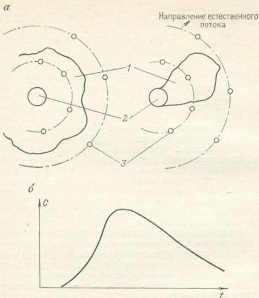
Рис. 4.2.8. Схема проведения многоскважинного опыта.
