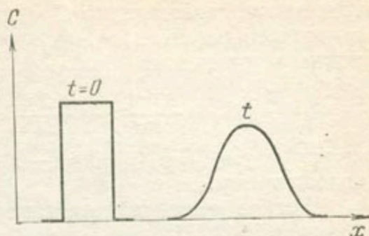
Рис. 2.5.2. Развитие ступенчатого импульса в результате дисперсии.
