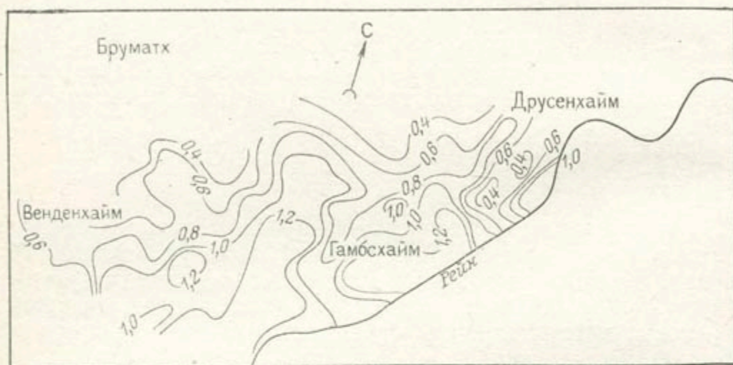
Рис. 4.3.2. План распределения проводимости (в 10^{-1} \text{ м}^2/\text{с} ) [71]
