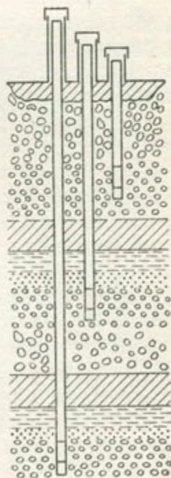
Рис. 6.1.11. Куст скважин для измерения давления и концентрации на различных глубинах
