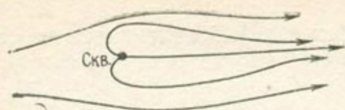
Рис. 4.2.9. Суперпозиция радиальной вынуждающей скорости и естественного фильтрационного потока
