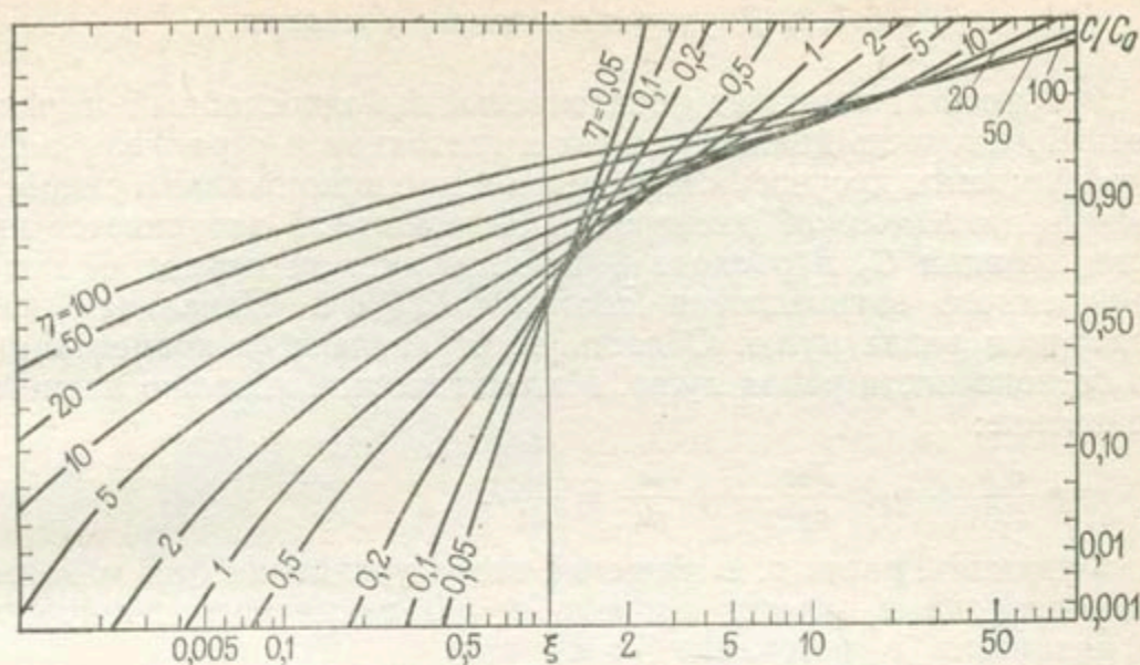
Рис. 5.3.1. Типичные кривые одномерной дисперсии; скорость постоянна [204]
