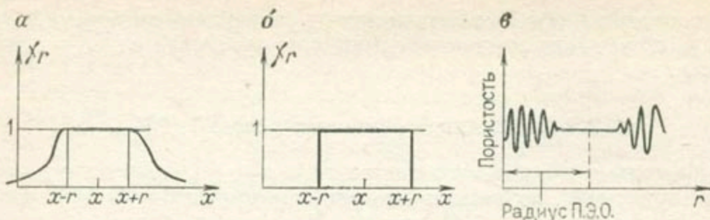
Рис. 2.3.7. Пример C^\infty \chi_r -функции (а); регуляризирующая функция Бэра (б); зависимость пористости от объема микрокосмического пространства (в)
