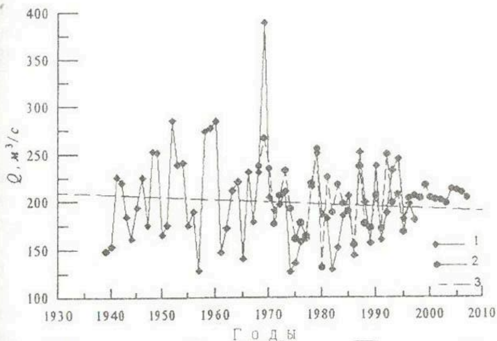
Рис. 2. Хронологический ход среднегодового притока воды в Чарвакское водохранилище и его прогноз. 1 — измеренные величины, 2 — прогнозные значения, 3 — тренд годовых величин.
