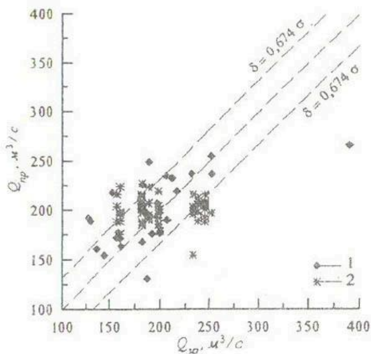
Рис. 1. Сопоставление прогнозных величин притока воды в Чарвакское водохранилище с измеренными значениями. 1 — зависимая, 2 — независимая выборка.
