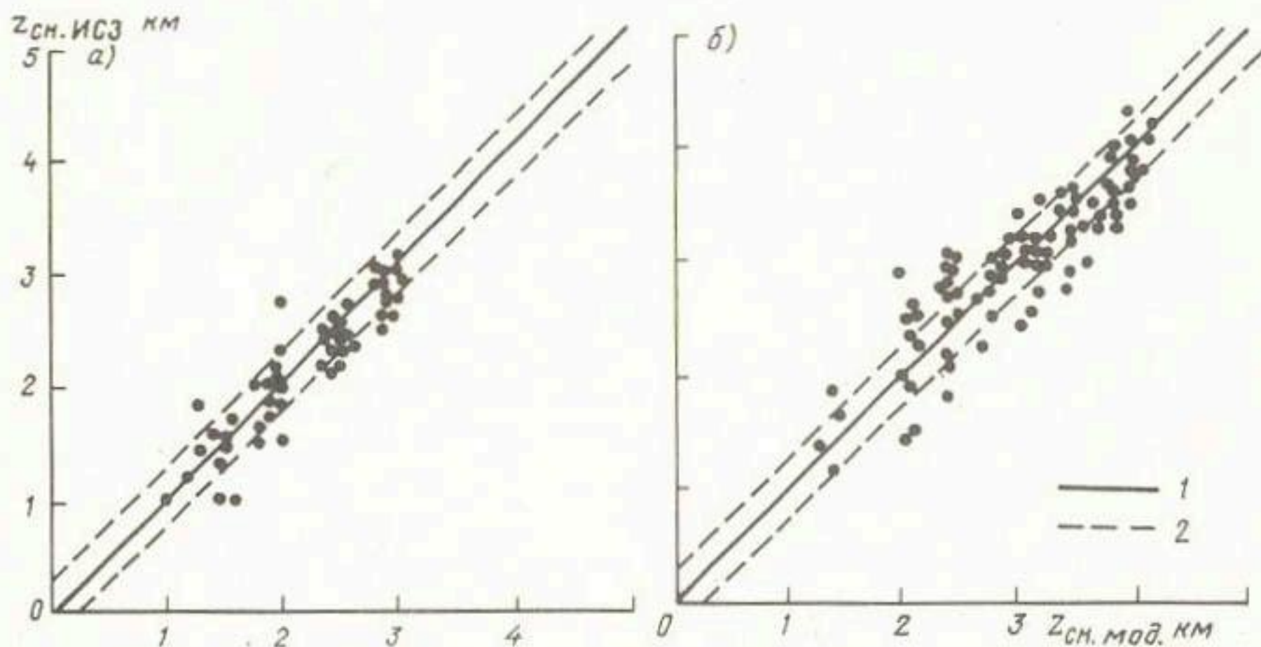
Рис. 7. Сравнение высот ССТГ, рассчитанных по модели и определенных по спутниковой информации, в бассейнах на юго-западном склоне Ферганского хребта (а) и на северном склоне Алайского хребта (б):
