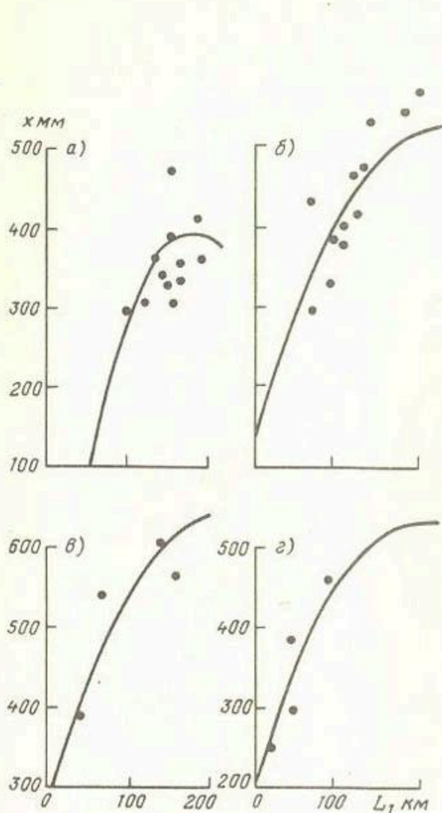
Рис. 3. График зависимости норм осадков за октябрь-март от расстояния от точки стыка Ферганского и Алайского хребтов на юго-западном склоне Ферганского хребта в разных высотных зонах: а - 1,0 км, б - 1,5 км, в - 2,75 км, г - 4,0 км. Точки - данные измерений
