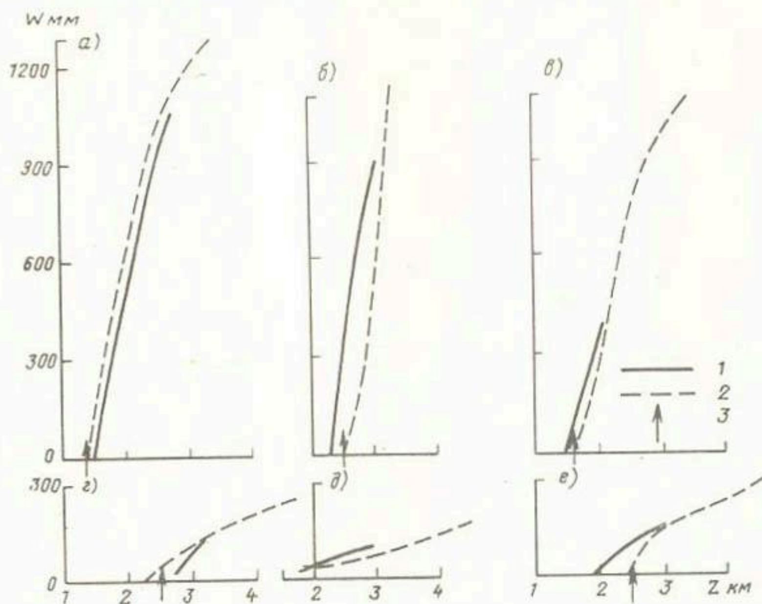
Рис. 5. Измеренные (1) и рассчитанные по модели (2) снегозапасы в 1969 г. в бассейнах рек Кутарт, 3-я декада марта (а); 3-я декада мая (б); Яссы, 3-я декада марта (в); Акбурн, 3-я декада марта (г); Сох, 3-я декада января (д); Исфайрамсай, 3-я декада марта (е); 3 - высота ССТ по спутниковой информации
