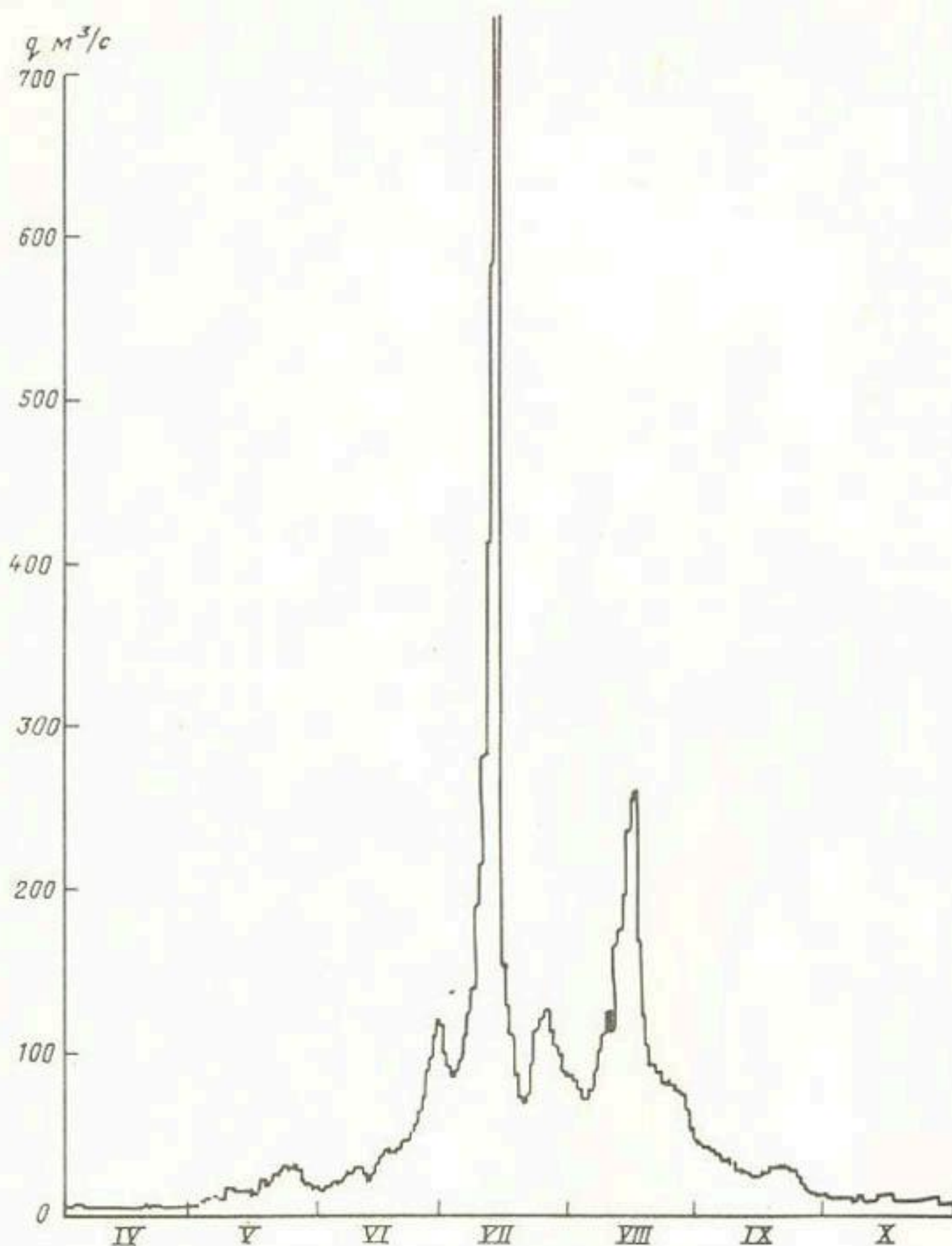
Рис. 2. Гидрограф стока р. Иньлечек в 1961 г. в створе, расположенном в 60 км ниже ледника
