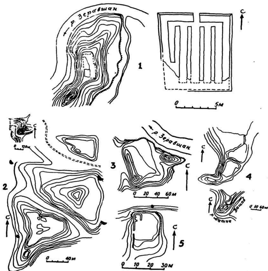
Рис. 2. Топографическая карта: 1—замка на горе Муг; 2—Сабие Кала в с. Рарз; 3—Калаи Дахони; 4—Калаи Джари Хисор в с. Вешаб. Планы: 1.
